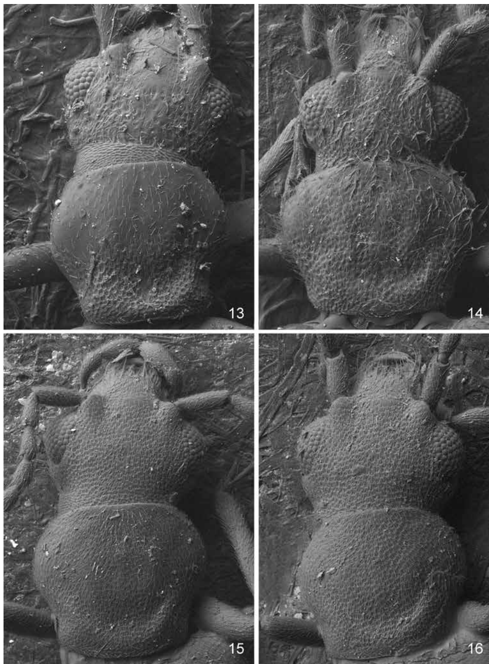
Figs. 13–16: Head and pronotum of 13) Thinodromus indicus (♂), 14) T. pubicollis (♂), 15) T. brincki (♂) and 16) same (♀).
