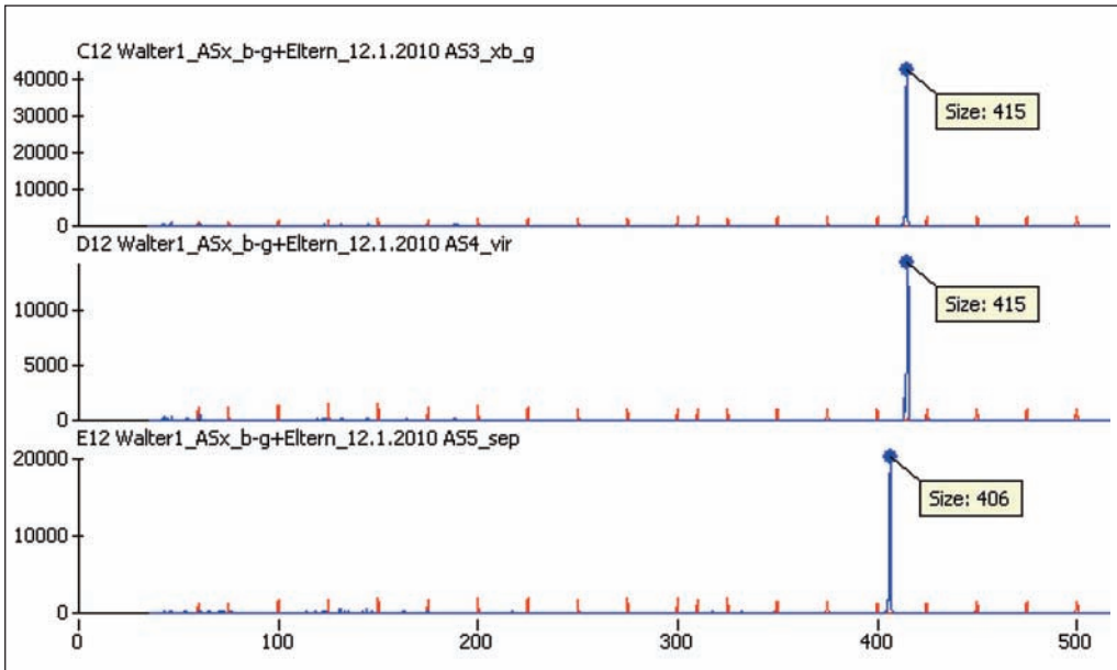
Abb. 5: Elektropherogramme von Genotypisierungen des trnL-trnF-Spacers von Asplenium xbosco-gurinense , A. viride (SJ-3762) und A. septentrionale (SJ-3678) (von oben) auf einem Kapillarsequenzierer (Amersham MegaBace). – Electropherograms of trnL-trnF spacer genotyping of A. xbosco-gurinense (top), A. viride (SJ-3762) and A. septentrionale (SJ-3678).
