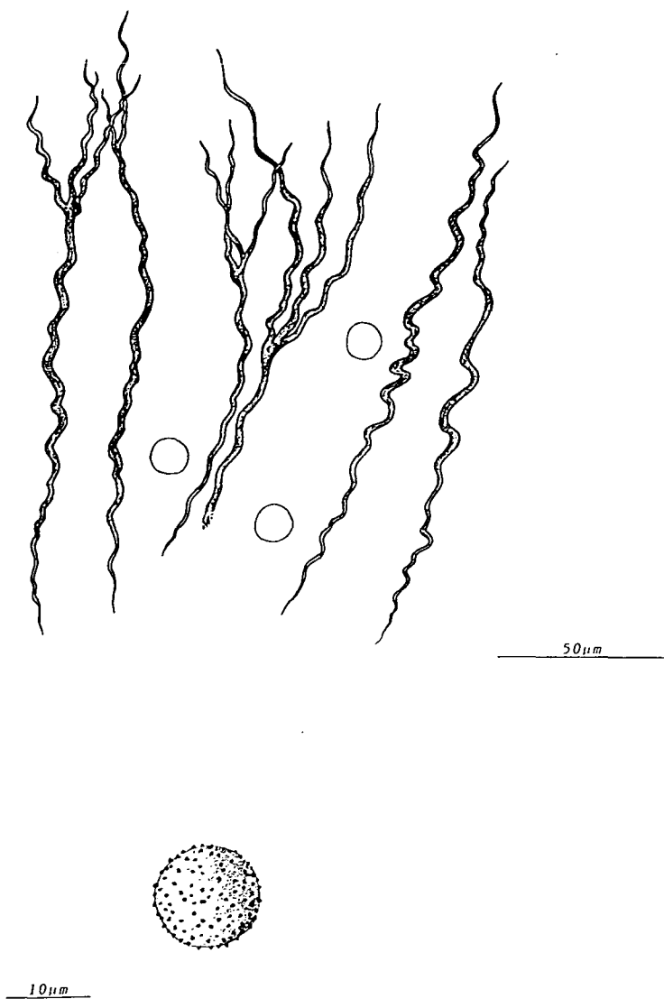
Abb.13: Didymium melanospermum : Nr. 1983: Capillitium und Spore
