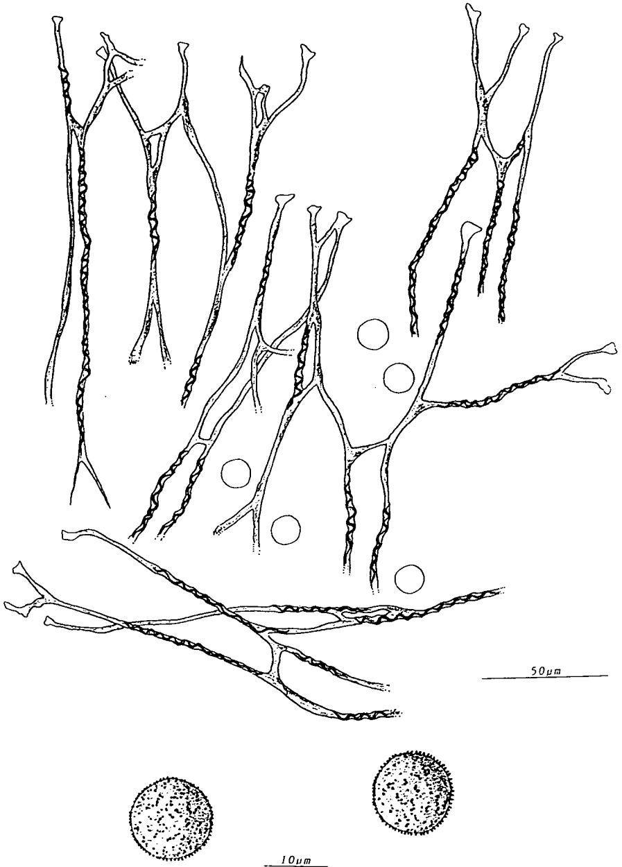
Abb.7: Didymium dubium (nivicol): Nr. 1723 (Frankreich): Capillitium und Sporen
