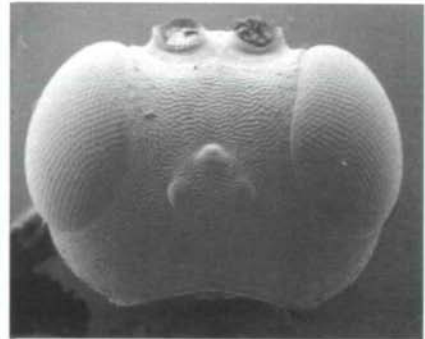
Abb. 60-61: G. rufipes (FÖRSTER) (♀); 60 – Clypeus, 61 – Mesonotum. Abb. 62-63: G. agilis (FABRICIUS) (♀); 62 – Kopf, 63 – Thorax und Propodeum.
