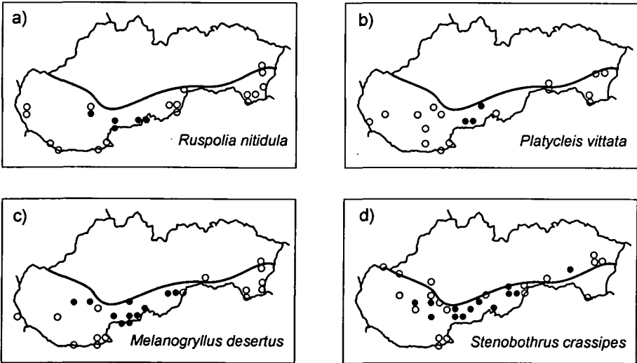
Abb. 2: Die Verbreitung von 4 Heuschreckenarten des pontischen Ursprungs in der Slowakei (schwarze Punkte – eigene Angaben, weisse Punkte – Literaturangaben, schwarze Linie – nördliche Grenze der Verbreitung der Zwergohreule in der Slowakei) (a - Ruspolia nitidula , b - Platycleis vittata , c - Melanogryllus desertus , d - Stenobothrus crassipes ).
