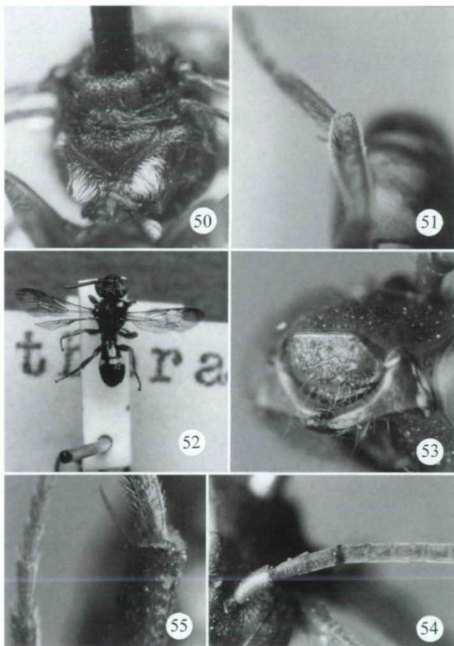
Abb. 50-55: (50-52) Nomada priscilla NURSE 1902 (Allolectotypus, ♂): (50) Skulptur und Behaarung des Propodeums; (51) Hinterschienende, rechts; (52) Gesamthabitus; (53-55) N. beata NURSE 1903 (53 Paralectotypus, 54-55 Lectotypus, ♀): (53) Labrumgestaltung; (54) Fühlerbasis, links; (55) Hinterschienende, rechts.
