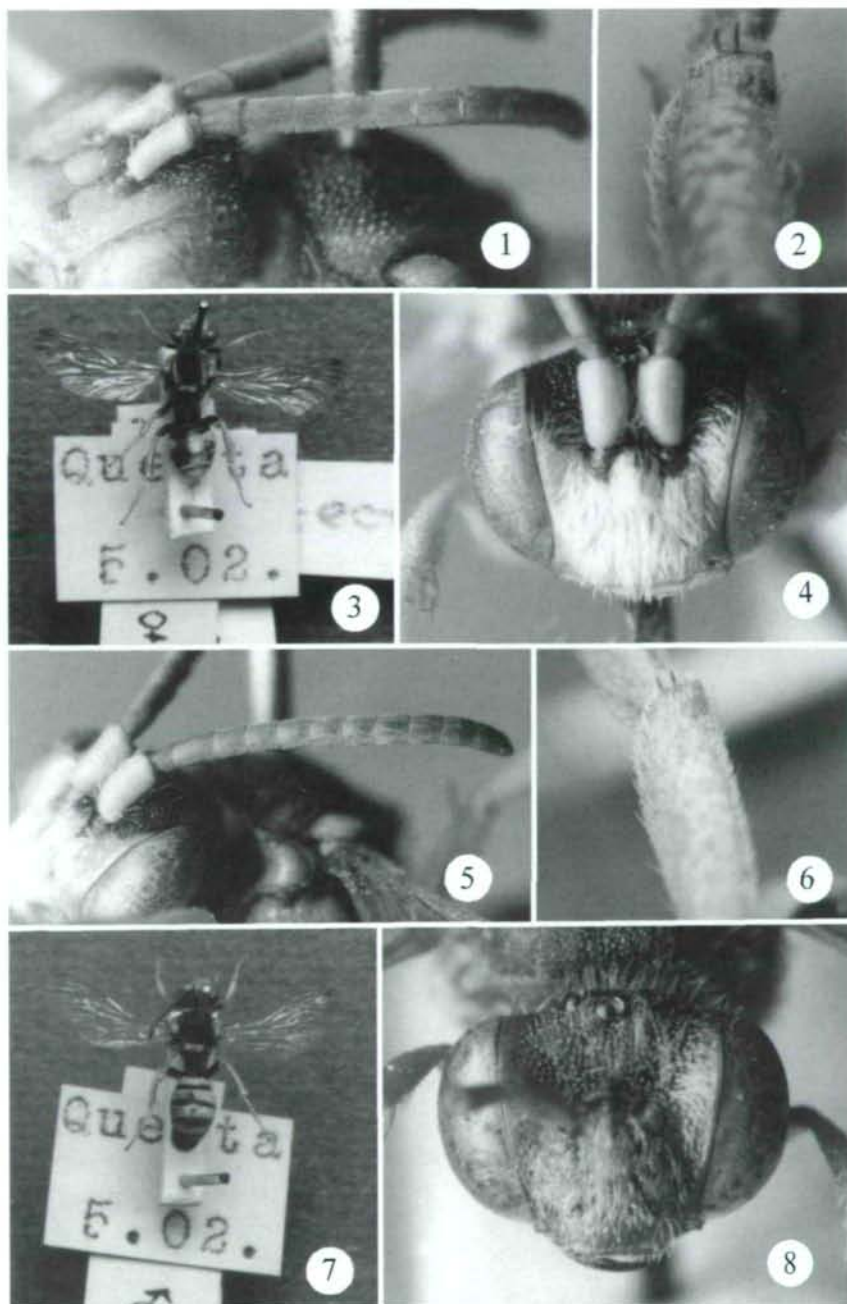
Abb. 1-8: (1-7) Nomada detecta NURSE 1904 (1-3 Paralectotypus, ♀; 4, 5, 7 Paralectotypus, ♂; 6 Allolectotypus, ♂): (1) Fühlerbasis, links, mit Gesichtsfärbung; (2) Hinterschienene, rechts; (3) Gesamthabitus; (4) Gesicht, Kopfform; (5) Fühlerbasis, links; (6) Hinterschienene, links; (7) Gesamthabitus; (8) N. flavozonata NURSE 1902 (Lectotypus, ♀): Gesicht.
