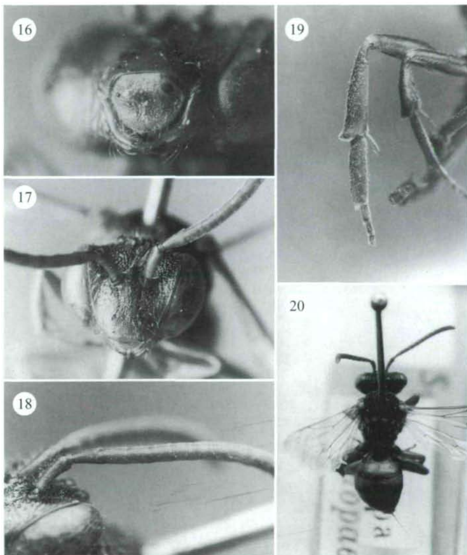
Abb. 16-20: Nomada subvirescens MORAWITZ 1875 ( N. desertorum MOR.) (18 Lectotypus, ♀ 16, 17, 19 und 20 Paralectotypus, ♀): (16) Labrumgestaltung; (17) Gesicht, Kopfform; (18) Fühlerbasis, links; (19) rechtes Hinterbein; (20) Gesamthabitus.
