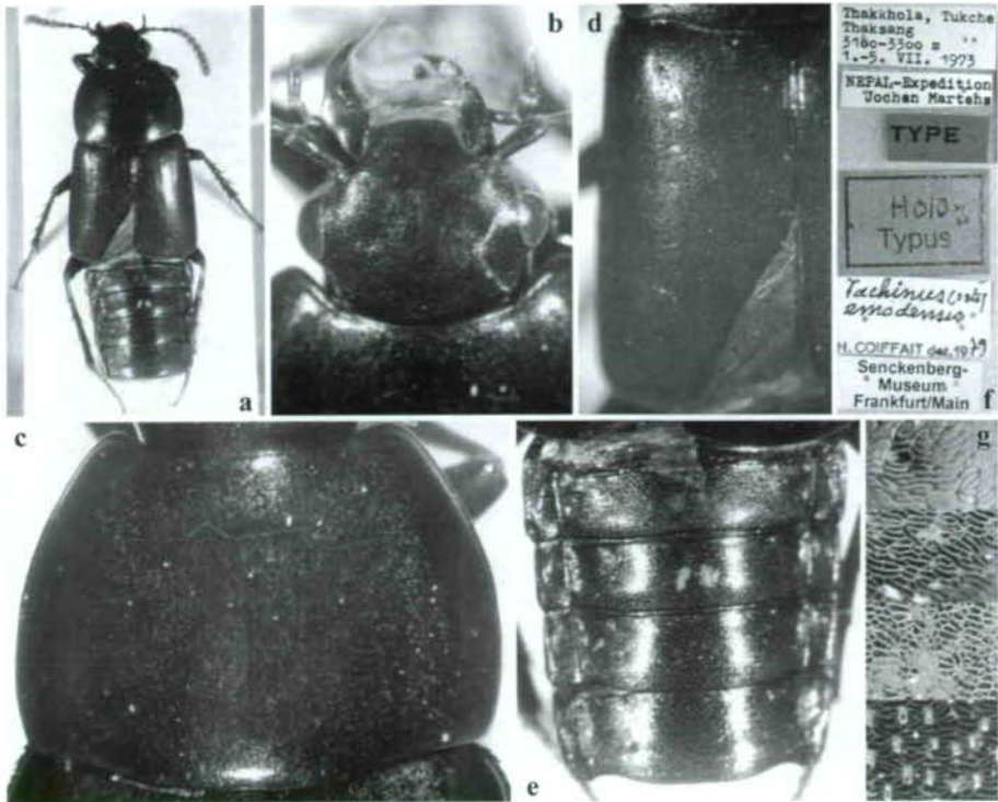
Abb. 7a-g: Tachinus bhutanicus ULLRICH ( \delta -Holotypus von Tachinus emodensis ): (a) Habitus; (b) Kopf; (c) Pronotum; (d) Elytre; (e) Abdomen; (f) Etikettierung; (g) Mikroskulptur (von oben nach unten: Kopf, Pronotum, Elytren, Abdomen).
