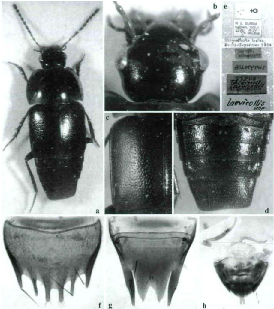
Abb. 9a-h: Tachinus laevicollis SCHEERPELTZ (♀-Allotypus): (a) Habitus; (b) Kopf; (c) Elytre; (d) Abdomen; (e) Etikettierung; (f) ♀-Sternit VIII; (g) ♀-Tergit VIII; (h) Segement IX/X und Spermathek.
