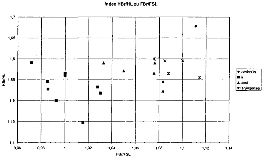
Abb. 18: Variabilität der Halschild- und Elytrenproportionen in der Tachinus laevicollis -Gruppe
