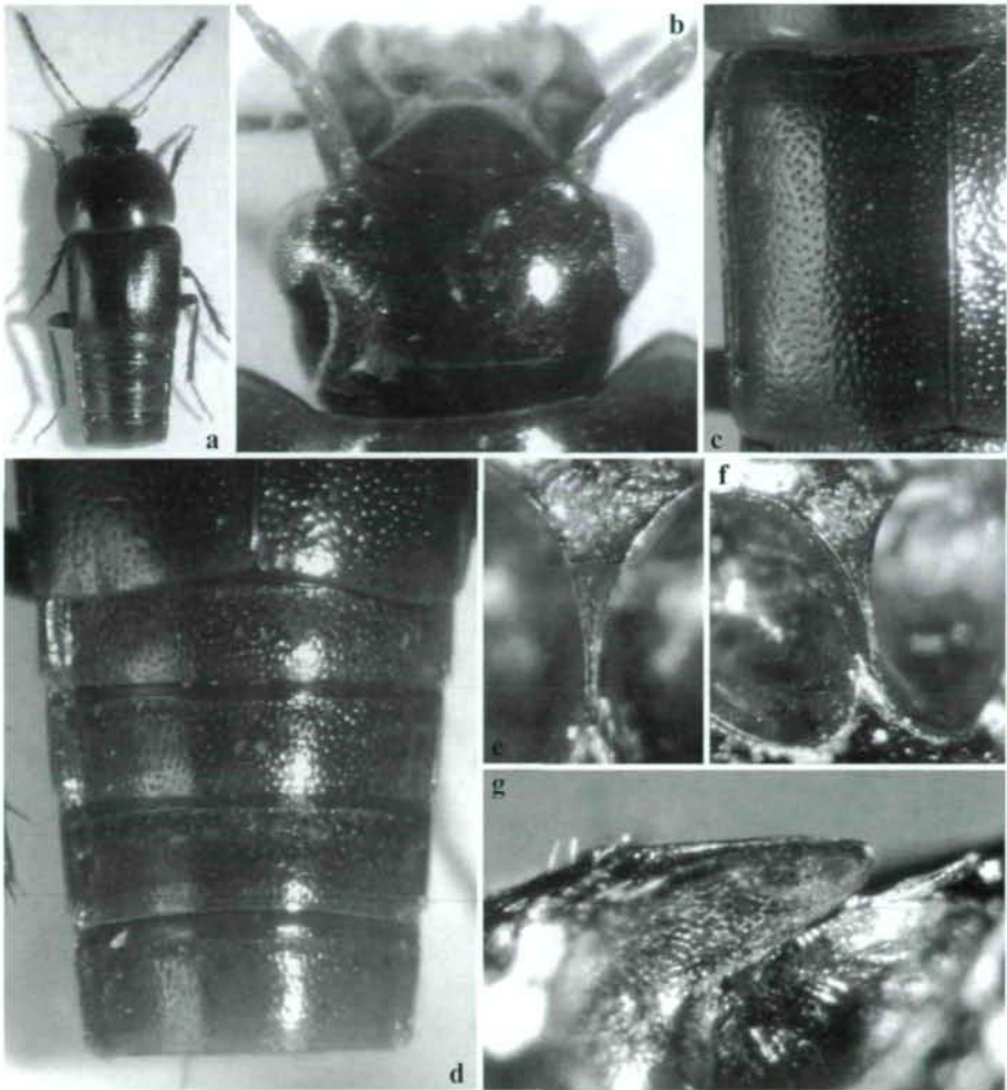
Abb. 15a-g: Tachinus alesi spec. nov., (a-d) Holotypus; (e-g) ♂-Paratypus, Nepal, Mechi: (a) Habitus; (b) Kopf; (c) Elytre; (d) Abdomen; (e) Mesosternalfortsatz, ventral; (f) Mesosternalfortsatz, ventrolateral; (g) Mesosternalfortsatz, lateral.
