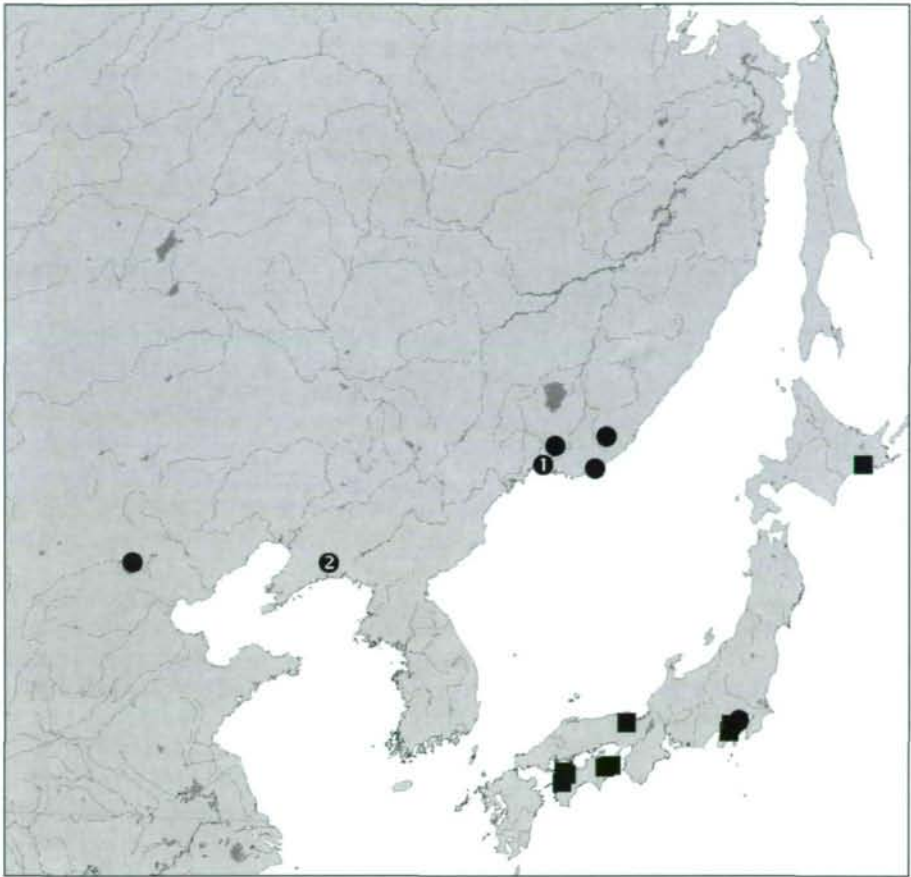
Karte 1: Bisher bekannte Verbreitung von Tachinus nigriceps SHARP: Holotypus von T. nigriceps manschuricus (❶); Holotypus von T. rubricollis (❷); Untersuchtes Material (●); Fundmeldungen von LI (1995) aus Japan (■).
