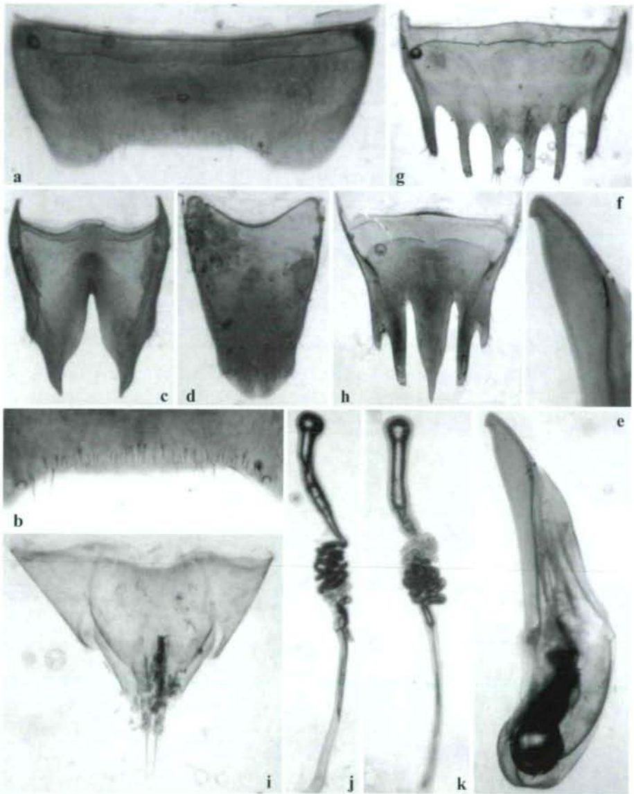
Abb. 22a-k: Tachinus striatipennis spec. nov., (a, b, e, f) ♂-Paratypus, Emei Shan; (c, d) Holotypus; (g-k) ♀-Paratypen, Emei Shan: (a) ♂-Sternit VII; (b) Hinterrand von ♂-Sternit VII; (c) ♂-Sternit VIII; (d) ♂-Tergit VIII; (e) Aedoeagus, lateral; (f) Apex der Parameren, lateral; (g) ♀-Sternit VIII; (h) ♀-Tergit VIII; (i) ♀-Segmente IX und X; (j, k) Spermatheken.
