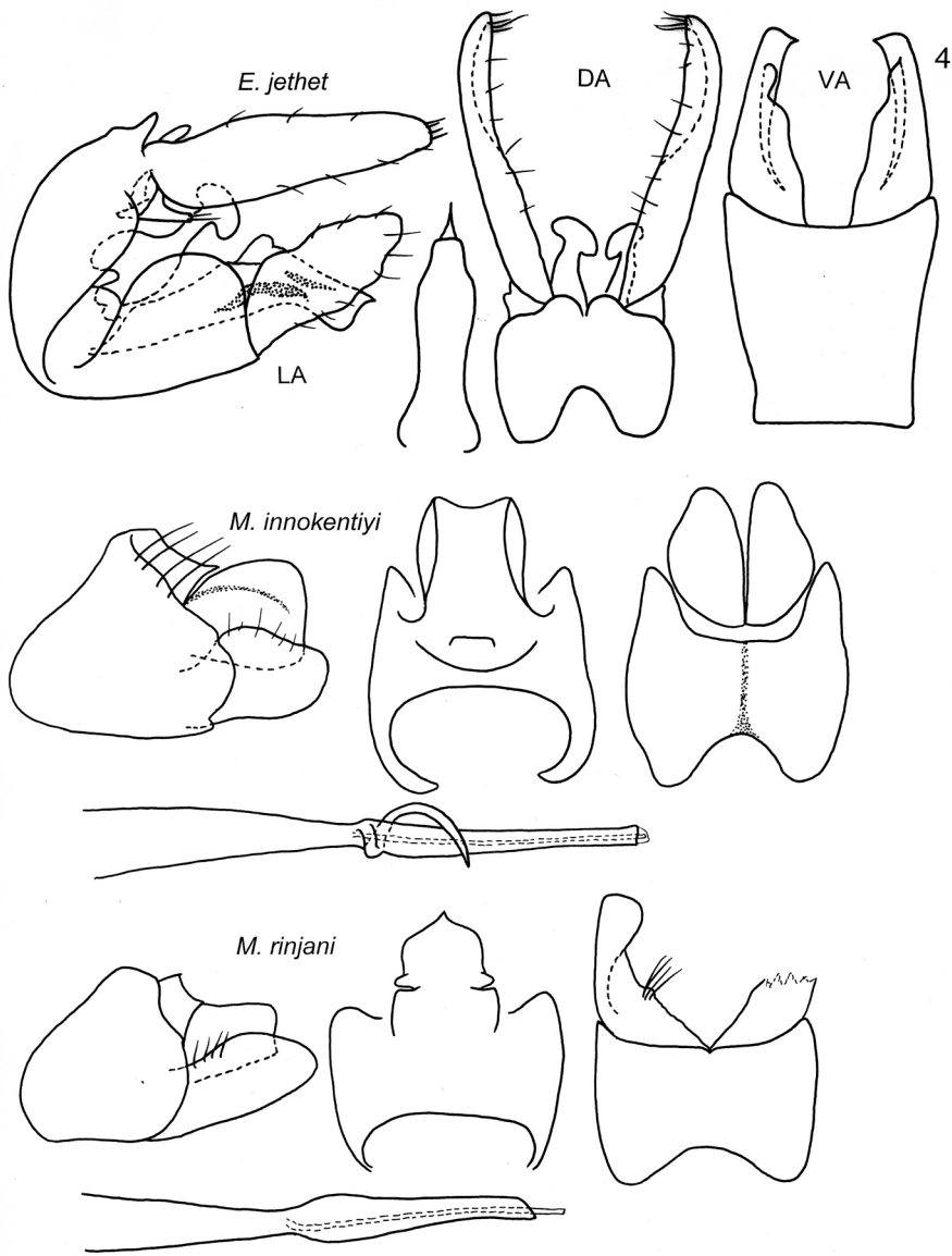
Tafel 4: ♂-Kopulationsarmaturen von Ecnomus jethet nov.sp., Microptila innokentiyi nov.sp. und Microptila rinjani nov.sp.
