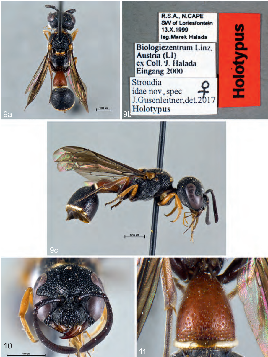
Abb. 9a-c: (9a) Stroudia idae nov.sp. ♀, Habitus; (9b) Etikett; (9c) Habitus lateral. Abb. 10-11: Stroudia idae nov.sp. ♀ (10) Clypeus; (11) 1. Tergit.
