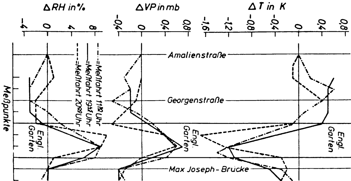
Abb. 7 Horizontalprofile von rel. Feuchte RH, Dampfdruck VP Und Lufttemperatur T während verschiedener Meßfahrten durch München ( aus BRÜNDL, 1980)
