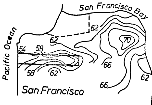
Abb. 6 Lufttemperaturen (in ° Fahrenheit) in San Francisco, 26. März 1952, 11 Uhr (aus DUCKWORTH und SANDBERG, 1954); das eingezeichnete Rechteck stellt den Golden Gate Park dar.
