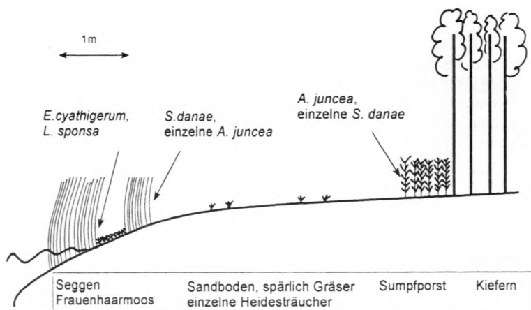
Abb. 1: Vegetationsstruktur und Schlupfporte vier verschiedener Libellenarten am Ufer des Sees Jezero Sasnowek, Nordpolen (poln. MTB 334.14). Die Daten stammen von einer Aufsammlung am 2. August 1995. Über die Anzahl festgestellter Exuvien siehe Tab. 1. - Vegetation and emergence sites of four different dragonfly species at the lake Jezero Sasnowek, northern Poland. All data were collected at 2 August, 1995. For the number of exuviae see Table 1.
