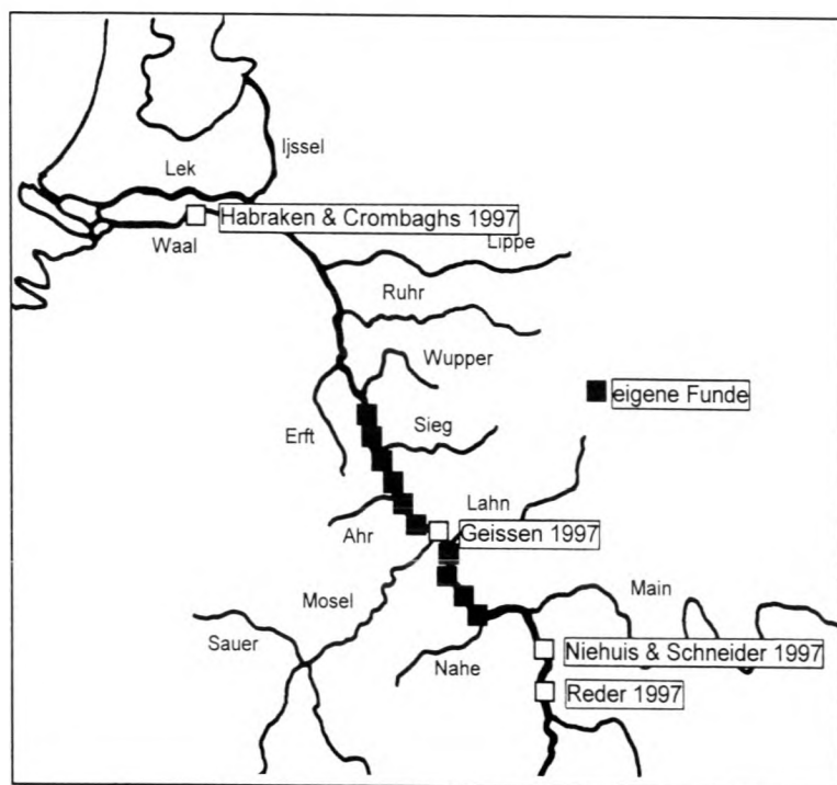
Abb. 1: Funde von Gomphus flavipes im Rhein.
