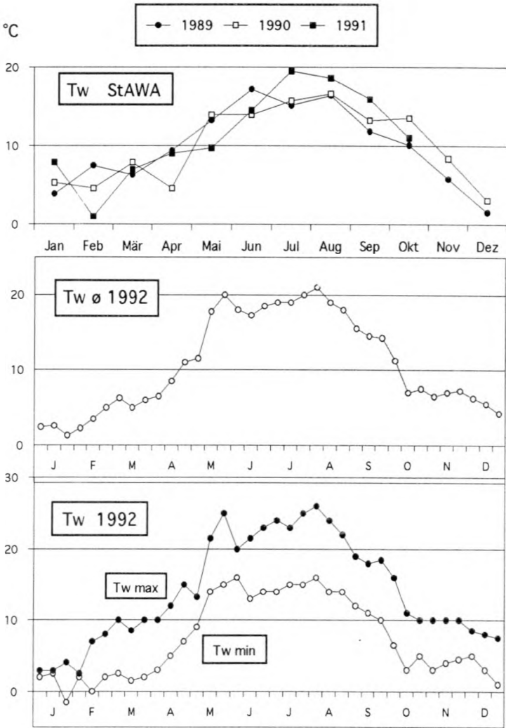
Abb. 6: Der Jahrestemperaturverlauf der Allerbeeke. Oben: Messungen des Staatlichen Amtes für Wasser und Abfall Sulingen (Je eine Messung pro Monat gegen 11:00 morgens); Mitte: Mittelwerte 1992 nach eigenen Messungen (drei bis vier Messungen pro Monat); Unten: Minimal- und Maximaltemperaturen 1992 nach eigenen Messungen (Tw = Wassertemperatur).
