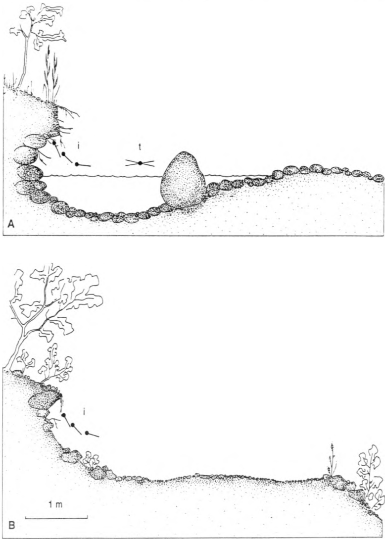
Abb. 1: Schnitt durch einen echten (A) und fiktiven (B) Rendezvous-/Eiablageplatz von Boyeria irene . (A) Ouvèze bei Buis-les-Baronnies, (B) Straßenböschung bei Puyméras. (i) Inspektionsflug, (t) Territorialflug. – Fig. 1: Cross section through a real (A) and a fictitious (B) oviposition / rendezvous site of Boyeria irene . (A) Ouvèze near Buis-les-Baronnies, (B) road side near Puyméras. (i) search flight, (t) territorial flight.
