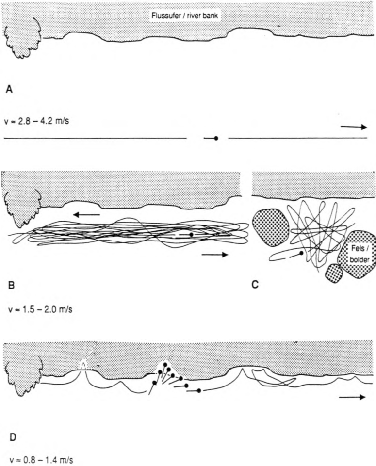
Abb. 2: Flugbahnen von Boyeria irene -Männchen beim Streckenflug (A), Territorialflug (B, C) und Suchflug (D). Sicht von oben auf das Flussufer. – Fig. 2: Flight paths of Boyeria irene during cruise flight (A), territorial flight (B, C) and search flight (D). View from above on the the river bank.
