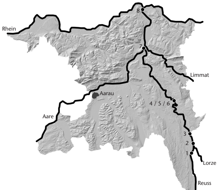
Abbildung 1: Lage der Projektgebiete an der Reuss (Nr. 1-6) und an der Aare (Nr. 7-8) im Kanton Aargau (Schweiz). Der Rhein bildet die Landesgrenze zu Deutschland. Grau: Kantonsfläche. — Figure 1: Location of the project sites on the rivers Reuss (no. 1-6) and Aare (no. 7-8) in the canton Aargau (Switzerland). The river Rhein constitutes the border between Switzerland and Germany. Grey: area of the canton Aargau.
