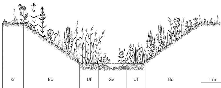
Abbildung 4: Querprofil durch den Seltenbach, Kanton Zürich, Schweiz. — Figure 4: Cross section through the Seltenbach stream, Canton of Zurich, Switzerland. Ge Gerinne, streambed; Uf Ufer, bank; Bö Böschung, slope; Kr Krone, crest.
