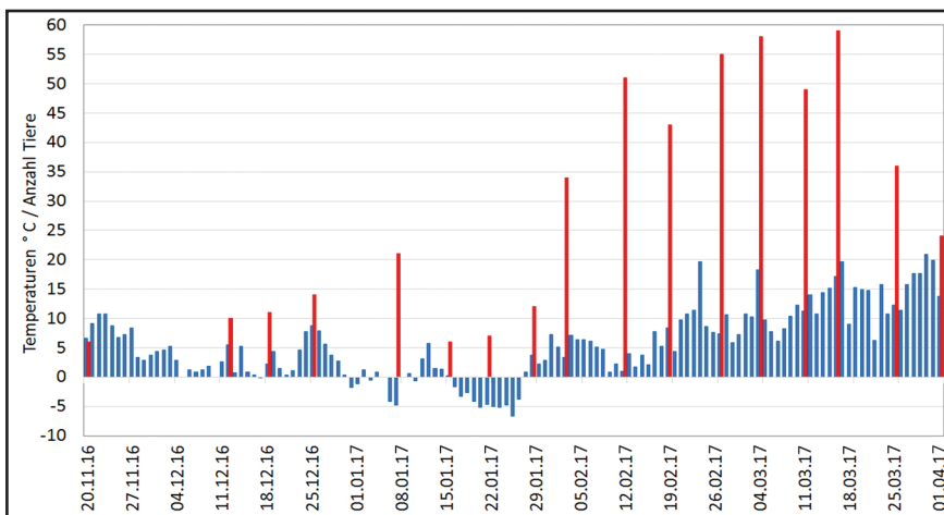
Abbildung 4: Temperaturverlauf mit den sprunghaften Veränderungen der Anzahl beobachteter Tiere in ihrem Winterhabitat 2016/17, Lengwiler Weiher. – Figure 4. Change in temperature with the rapid change in the number of observed insects in their winter habitat 2016/17, Lengwiler Weiher. ■ Anzahl Individuen, number specimens; ■ mittlere Lufttemperatur, air temperatur [°C]; Quelle Temperatur, source temperature: hydrodaten.tg.ch
