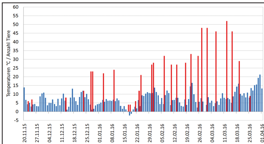
Abbildung 3: Temperaturverlauf mit den sprunghaften Veränderungen der Anzahl beobachteter Tiere in ihrem Winterhabitat 2015/16, Lengwiler Weiher. – Figure 3. Change in temperature with the rapid change in the number of observed specimens in their winter habitat 2015/16, Lengwiler Weiher. ■ Anzahl Individuen, number specimens; ■ mittlere Lufttemperatur, air temperatur [°C]; Quelle Temperatur, source temperature: hydrodaten.tg.ch
