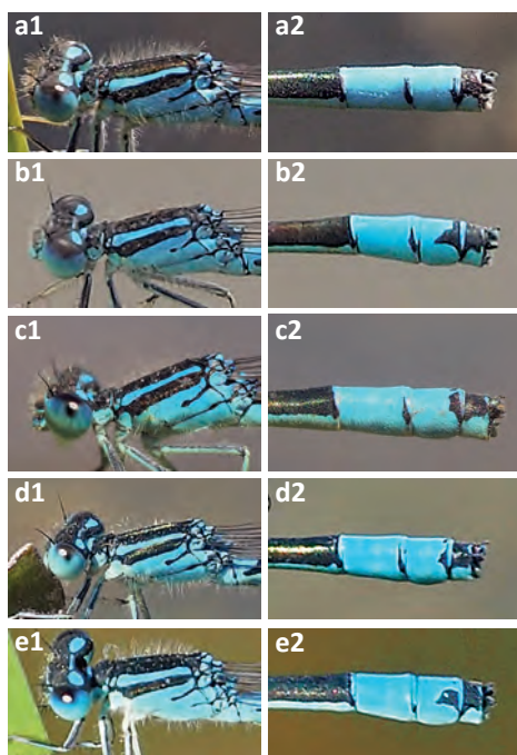
Abbildung 2: Individuelle Zeichnungsmuster an Thorax und Abdomenspitze von fünf Coenagrion scitulum -Männchen. – Figure 2. Individual patterns of thorax and abdominal tip of five male Coenagrion scitulum . a, b Egelseeriet/Schönbühl; c–e Weierried/Zell; a 26-vi-2015, b 04-vii-2018, c 16-vii-2018, d 10-vii-2019, e 18-vii-2019. Photos: HW
