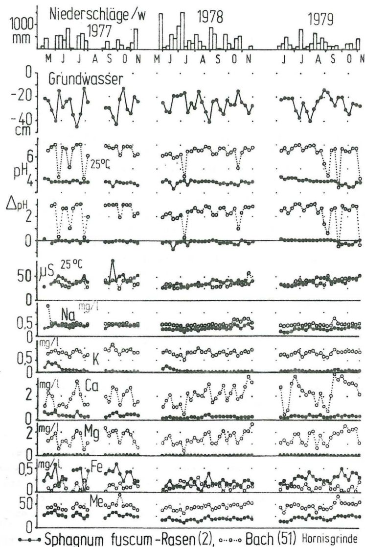
Abb.2: Niederschlag, Grundwasserstand und chemische Parameter an zwei Meßstellen aus den Biberkessel-Mooren (Nord-schwarzwald)
