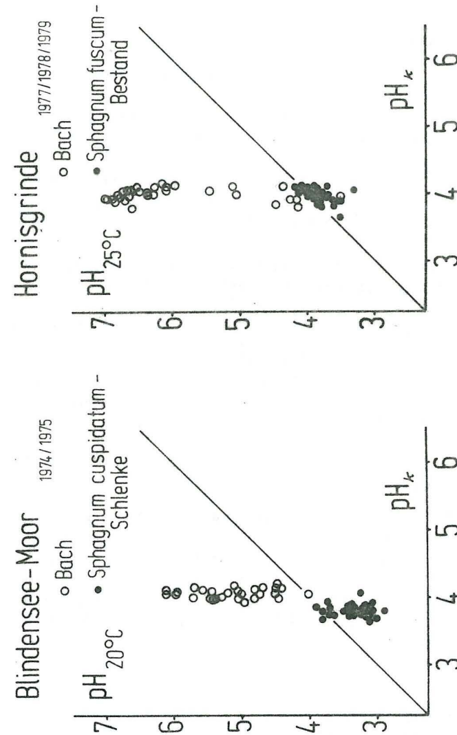
Abb.1 : Korrelation zwischen gemessenem und aus der Leitfähigkeit errechnetem pH - Wert
