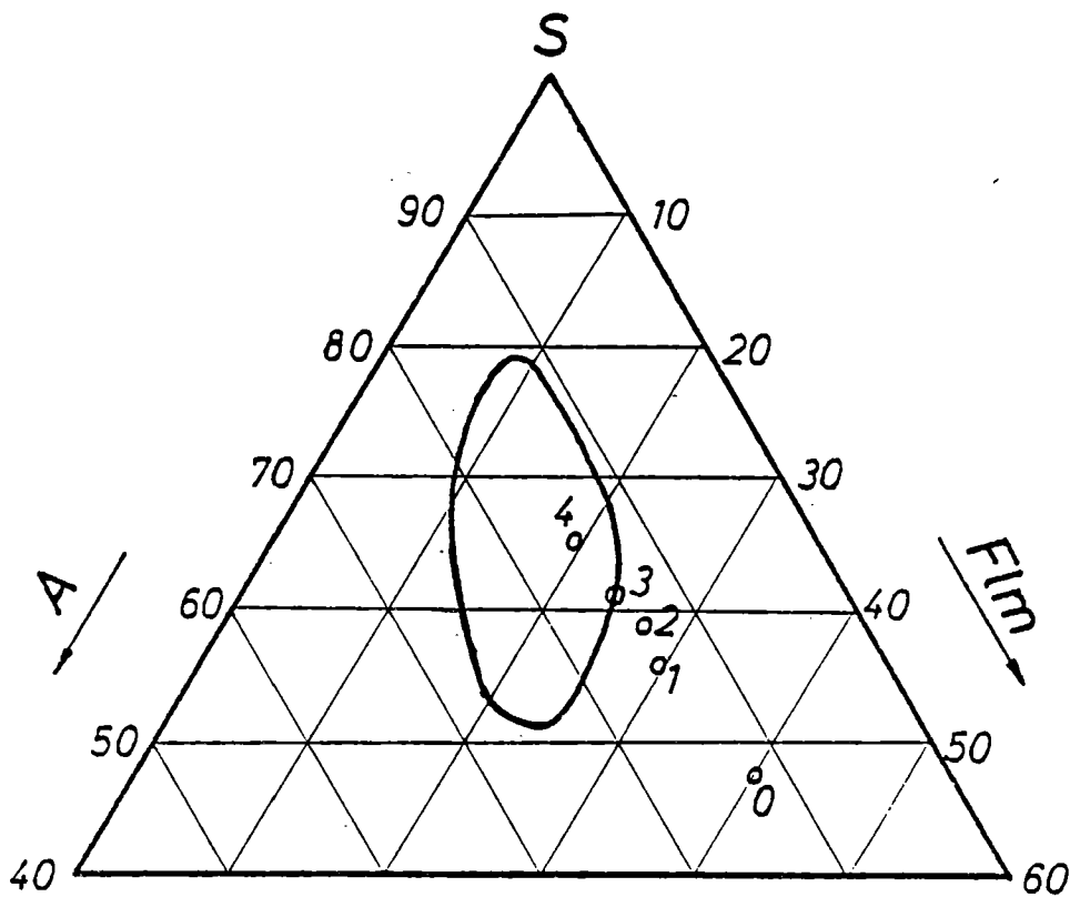
Bild 10: Dreistoffsystem nach Riley mit eingezeichneten Blähversuchsmischungen. S = \text{SiO}_2 , A = \text{Al}_2\text{O}_3 , Flm = Summe der Flußmittel nach 2 Riley (1). 3 Die Prozentangaben auf den Dreieckseiten sind Masse-%. Mischungsnummern sind dieselben, wie in Tabelle 3.
