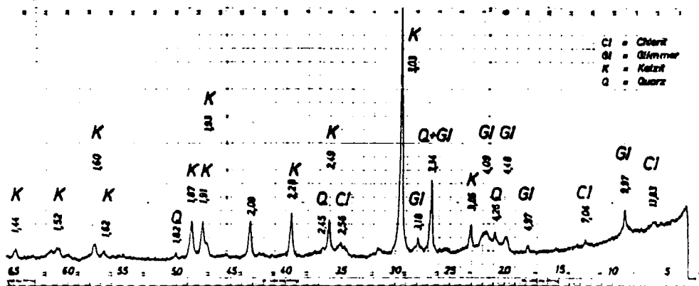
Bild 7: Röntgendiffraktometerdiagramm des Rohmergels.
