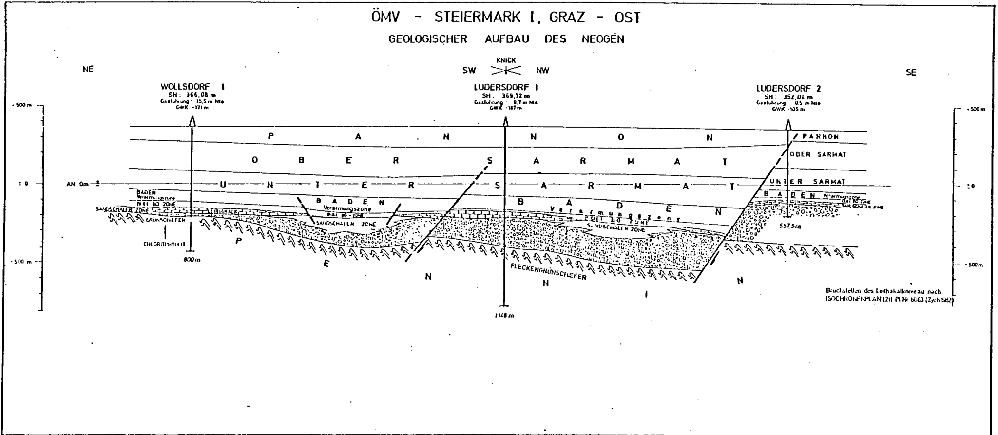
Abb. 2: Geologisches Profil im Raum Ludersdorf - Wollsdorf (von der ÖMV AG übernommen)
