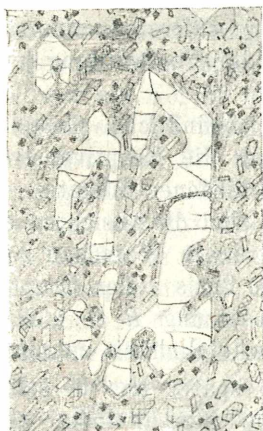
Fig. 2. Corrodirtter Olivin.
