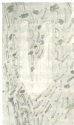
Fig. 3. Corrodirtter Augit.
