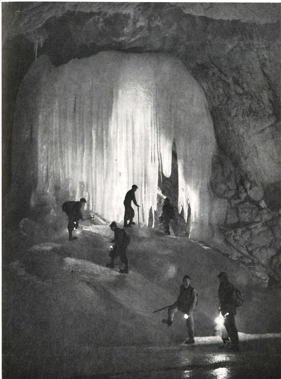
Abb. 3 Eisevorhang in der Eiseriesenwelt (Tennengebirge). Foto: C. Pospesch
