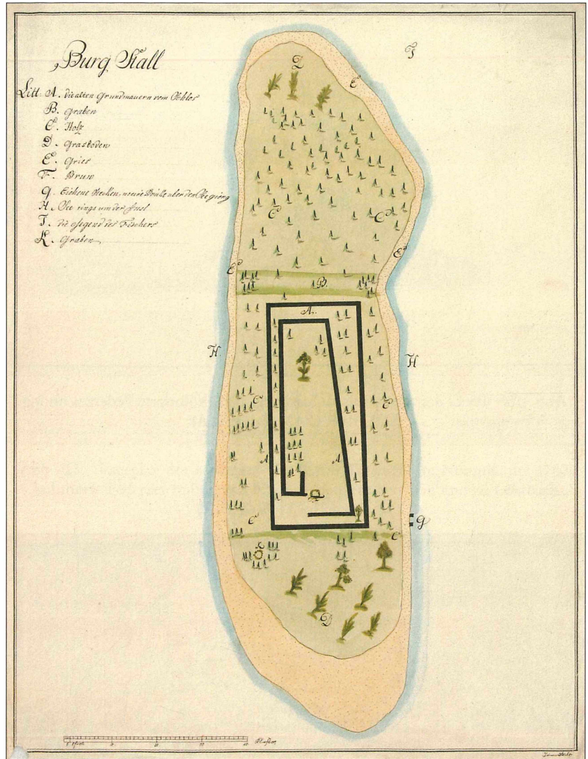
Abb. 17 Bauaufnahme (Grundriss) der Ruine auf der Insel Burgstall im Abtsee, um 1780, kolorierte Federzeichnung (SLA, KuR J.66; Foto: SLA).
