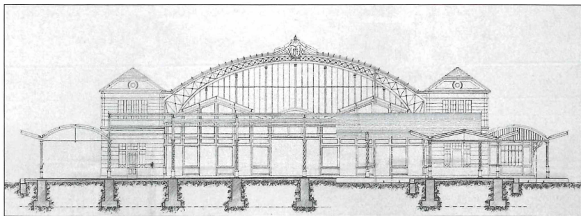
Abb. 31 Plan der noch bestehenden Halle am neu zu errichtenden Zentralperron im Zusammenhang mit dem Aus- und Umbau der „Personendienstanlage“ des k.k. Staatsbahnhofes Salzburg im Jahr 1907, vorgelegt am 8.1.1907 durch E. Baudisch vom k.k. Eisenbahn-Ministerium, Departement 18a (SLA, LAus 1880/1938 III 04/03/11; Foto: SLA).
