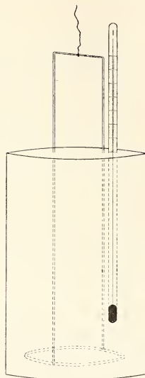
Abkühlungsgefäß.
