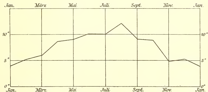
Die unperiodischen Schwankungen der Lufttemperatur. (Differenz zwischen Durchschnittsmax. und Durchschnittsmin.).
