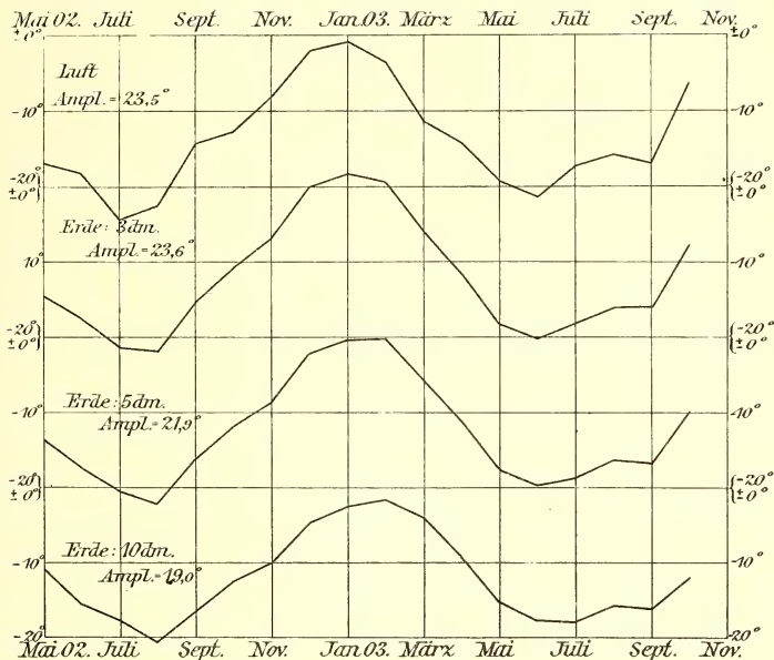
Jährlicher Gang der Temperatur in Luft und in Boden.
