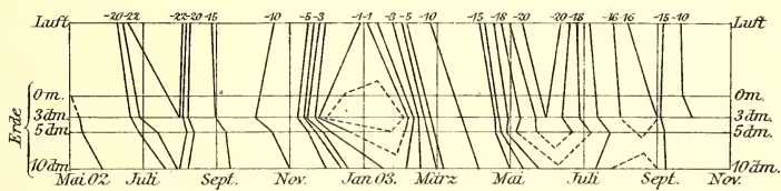
IsoPLETHEN die Bodentemperatur anzeigend.
