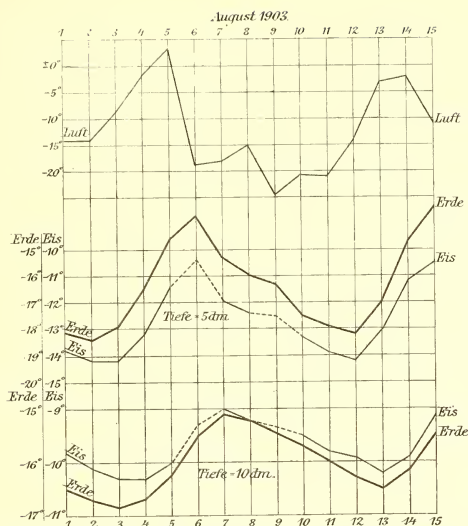
Vergleich zwischen dem Verlauf der Temperatur in der Luft, im Boden und im Meereis.
