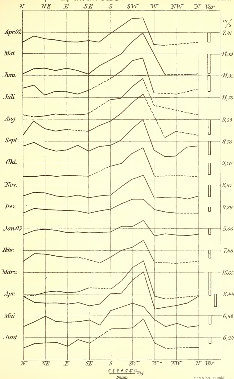
Dynamische Windrosen I.
