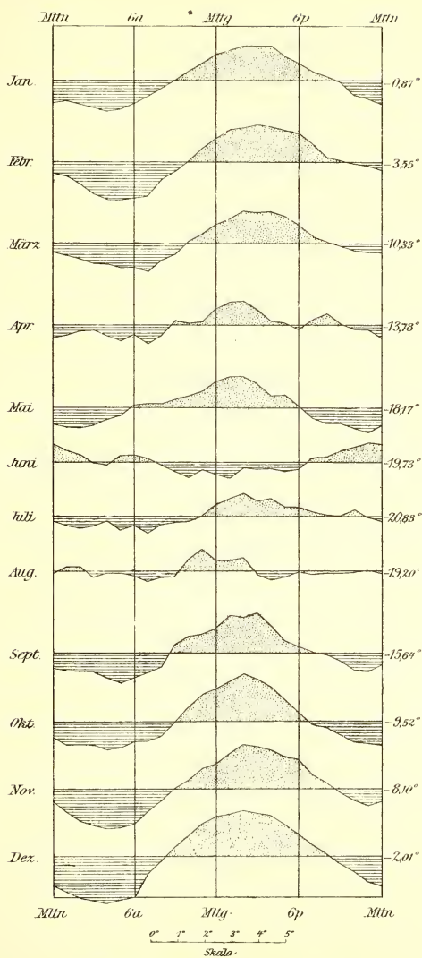
Täglicher Gang der Lufttemperatur I.
