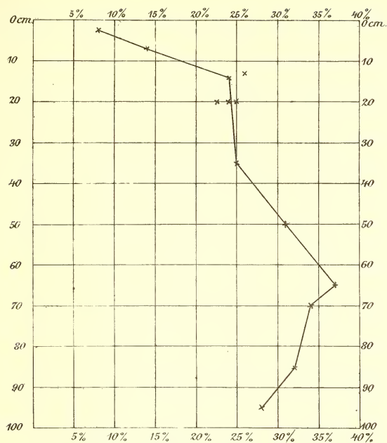
Wasserhalt des Snow-Hill-Bodens in verschiedenen Tiefen, ausgedrückt i Gewicht %.
