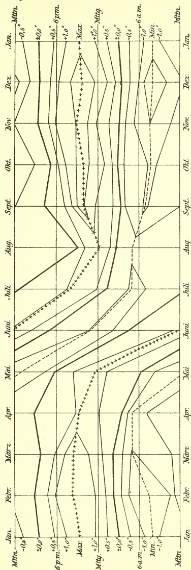
Isoplethen, die Abweichungen der Temperatur vom Tagesmittel angehend.
