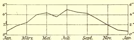
Jährlicher Gang der interdiurnen Veränderlichkeit der Lufttemperatur.
