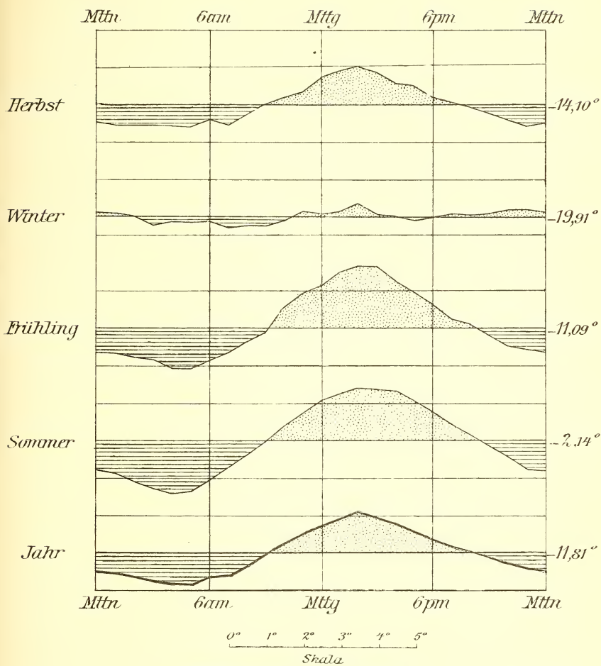
Täglicher Gang der Lufttemperatur II.
