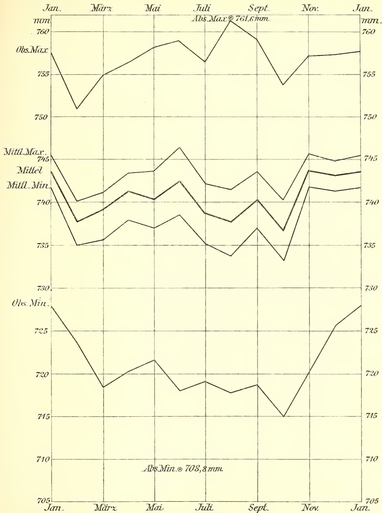
Jährlicher Gang des Luftdrucks.
