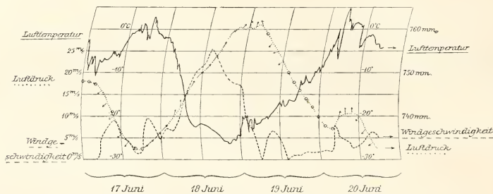
17 Juni—20 Juni 1902: Lufttemperatur, Luftdruck und Windgeschwindigkeit.
