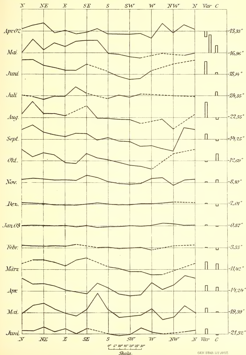
Thermische Windrosen I.
