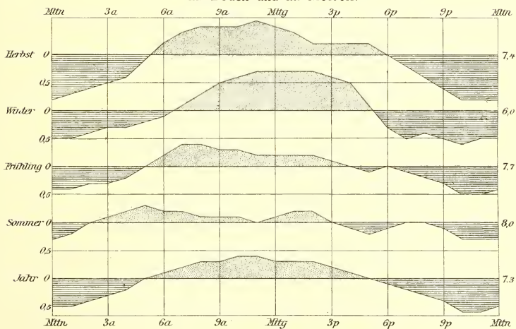
Täglicher Gang der Bewölkung.
