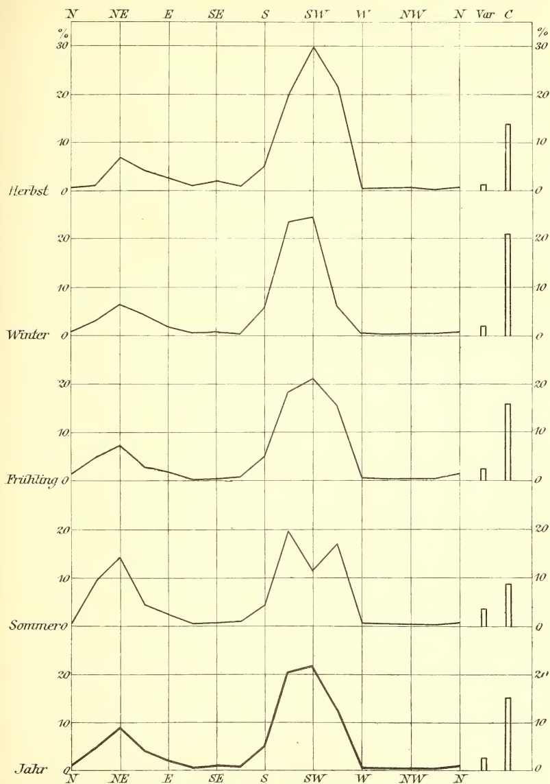
Prozentische Häufigkeit der verschiedenen Windrichtungen.
