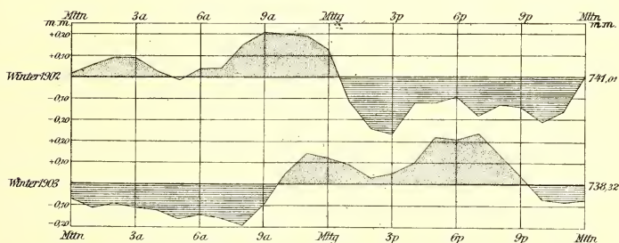
Täglicher Gang des Luftdrucks im Winter 1902 und im Winter 1903
