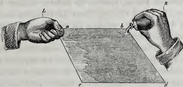
Fig. 7. Aufgiessen des Collodions auf die Glasplatte. L ) Linke Hand. R ) Rechte Hand. a b c d ) Die vier Ecken der Glasplatte.
