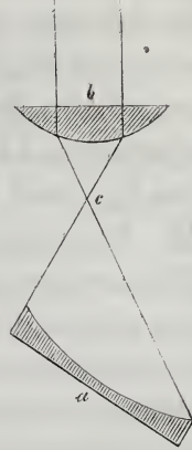
Fig. 1. Schematische Darstellung des Ganges der Lichtstrahlen zur Erzielung concentrirten parallelen Lichtes. a) Hohlspiegel. b) Planconvexe Linse. c) Brennpunkt beider.
