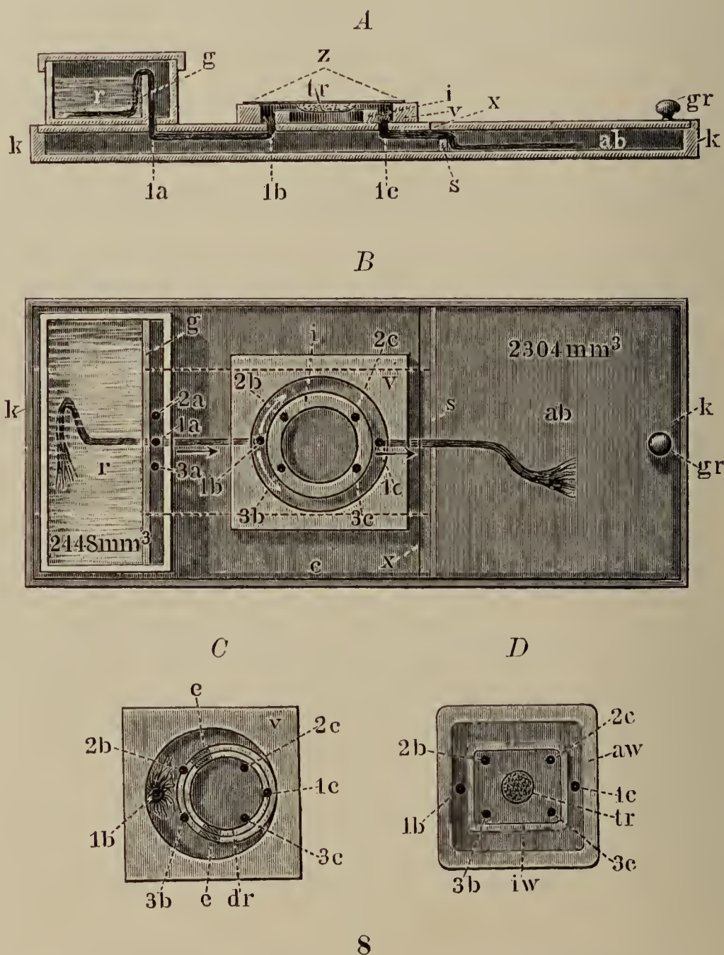
Circulationskästchen. A verticaler Durchschnitt. B Ansicht von oben, C Zelle mit Doppelring von Glas zum Ausspannen von Membranen, D die Oelrahmen einer Ricinusölzelle und ihre Lage zu den Löchern für die Wollfäden. r Reservoirkästchen, k Glaskästchen als Objectträger, gr Knopf zum Abheben der Deckelplatte rechts von der Linie x , ab Abflussraum, g Querwand im Reservoirkästchen, s Septum, welches den Abflussraum der Büchse abtrennt. 1a, 2a, 3a, 1b, 2b, 3b, 1c, 2c, 3c Oeffnungen, wo die zu- und ableitenden Fäden durchgeführt werden. v viereckige Glaszelle mit runder Oeffnung, i innerer Glasring, dr Doppelring, e Einschnitt am unteren Rand der Ringe, aw äusserer, iw innerer Wall von Ricinusöl, tr Tropfen mit dem Untersuchungsobject.
