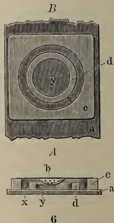
Combinirte Kammern für den hangenden Tropfen. A im verticalen Durchschnitt, B von oben gesehen. a Objectträger, b Deckglas mit dem hangenden Tropfen, c äussere Zelle, d innerer Ring, x Raum für Wasser, Algen etc., y centraler Raum für den Tropfen.
