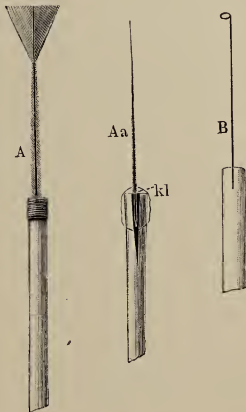
A Federpinsel von der Fläche, Aa von der Seite, in das gespaltene Ende eines Holzstäbchens hineingezwängt und mit etwas Klebwachs kl befestigt. B Drahtschlinge in das Ende eines Glasstäbchens gesteckt.
