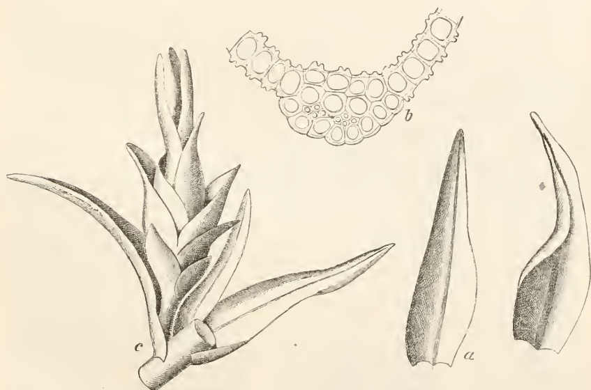
Molendoa tenuinervis . a 2 Laubblätter \frac{4}{1} , b Querschnitt durch die Blattrippe \frac{3}{1} , c ♀ Blüthenspross \frac{4}{1} .
