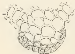
Tortula pulvinata. Blattrippe im Querschnitt \frac{2}{1} \frac{0}{1} .
