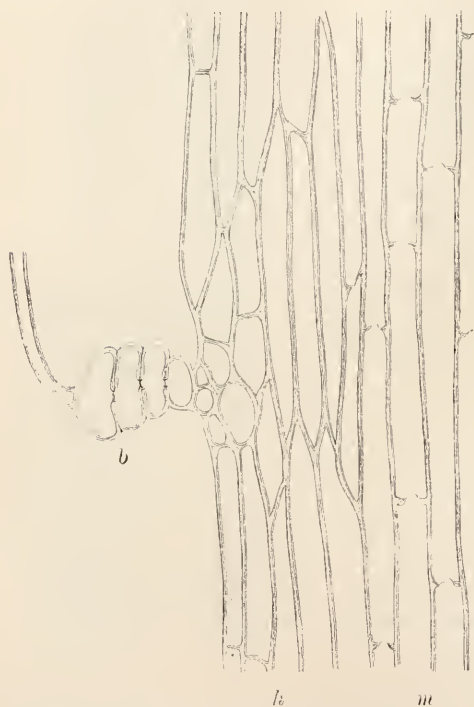
Insertion eines Stengelblattes (b) von Sphagnum riparium Aongstr. Längsschnitt durch einen Stengel; l Holzkörper, m Markscheit.
