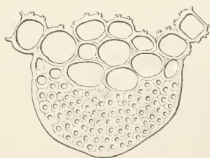
Tortula montana (Nees). Blattrippe im Querschnitt 2\frac{0}{1} .
