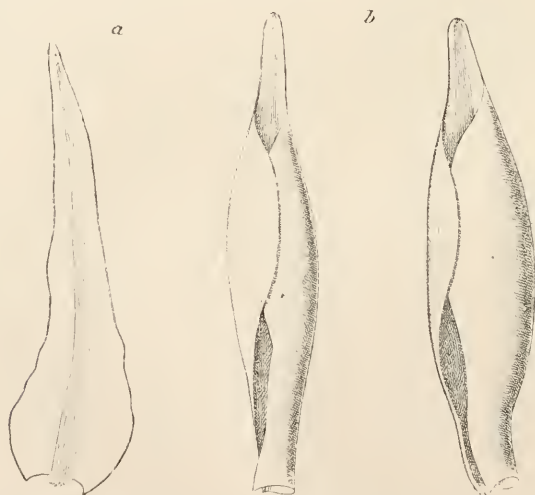
Andreaea Rothii W. & M. Westf. Laubm. No. 61. a Laubblatt, b die inneren Perichätialblätter 57 .
