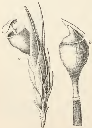
Stylostegium caespitium (Schwägr.). a Spross mit seitlich austretender Kapsel, b reifes Sporogon. \frac{2}{1} .
