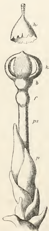
Fruchtsack von Andreaea petrophila ( \frac{2}{1} ). b ungetheilte Basis der Kapsel; f Fusstheil des Sporogons; h Haube; k Klappen der Kapsel; p Perichätialblätter; ps Pseudopodium.
