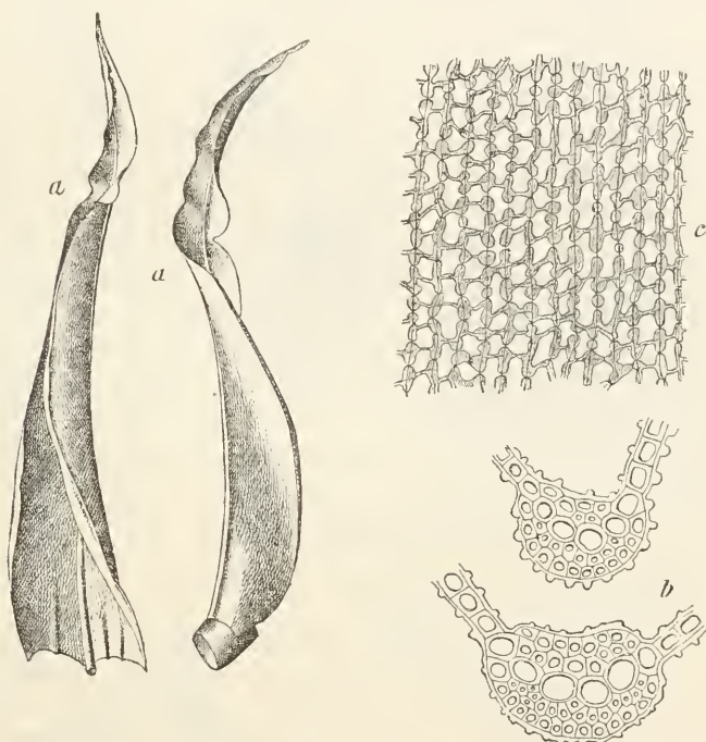
Didymodon giganteus (Funck). a Blätter \frac{2}{1} \frac{4}{1} , b zwei Querschnitte durch die Blattrippe \frac{2}{1} \frac{8}{1} \frac{0}{1} , c Zellnetz der Blattmitte \frac{2}{1} \frac{8}{1} \frac{0}{1} .
