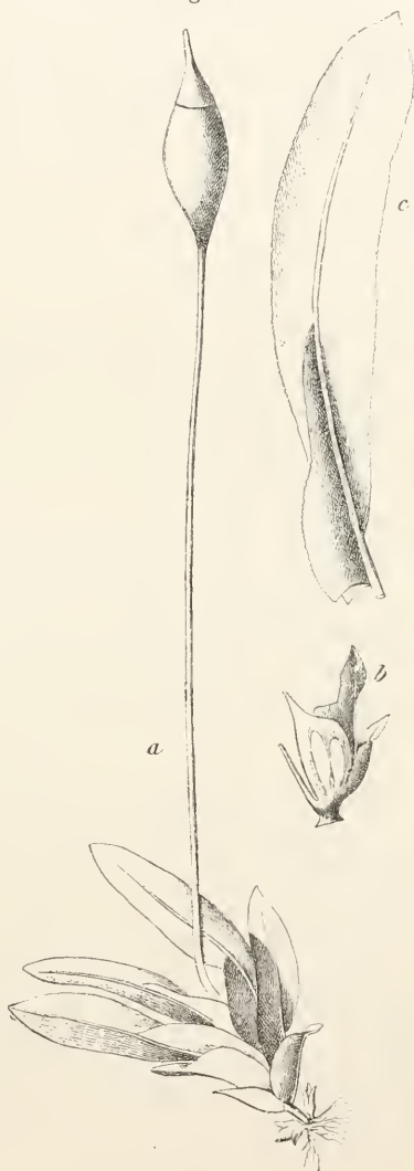
Fissidens exilis Hedw. a Habitus- bild \frac{2.0}{1} , b Grundständiges ♂ Pflänz- chen \frac{4.5}{1} , c Perichätialblatt \frac{4.5}{1} .
