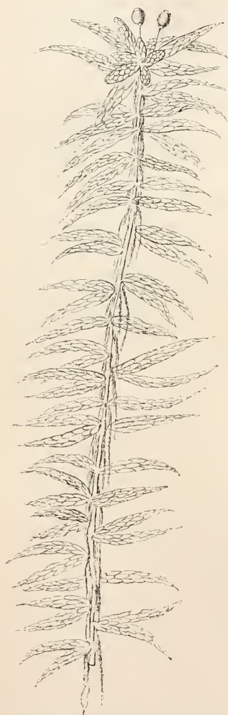
Sphagnum cymbifolium Ehrh. Habitusbild in natürlicher Grösse.
