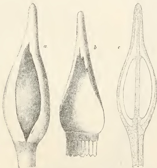
Voitia nivalis Hornsch. a Kapsel in der Haube eingeschlossen \frac{3}{4} . b Haube frei \frac{3}{4} . c Kapsellängsschnitt \frac{3}{4} .
