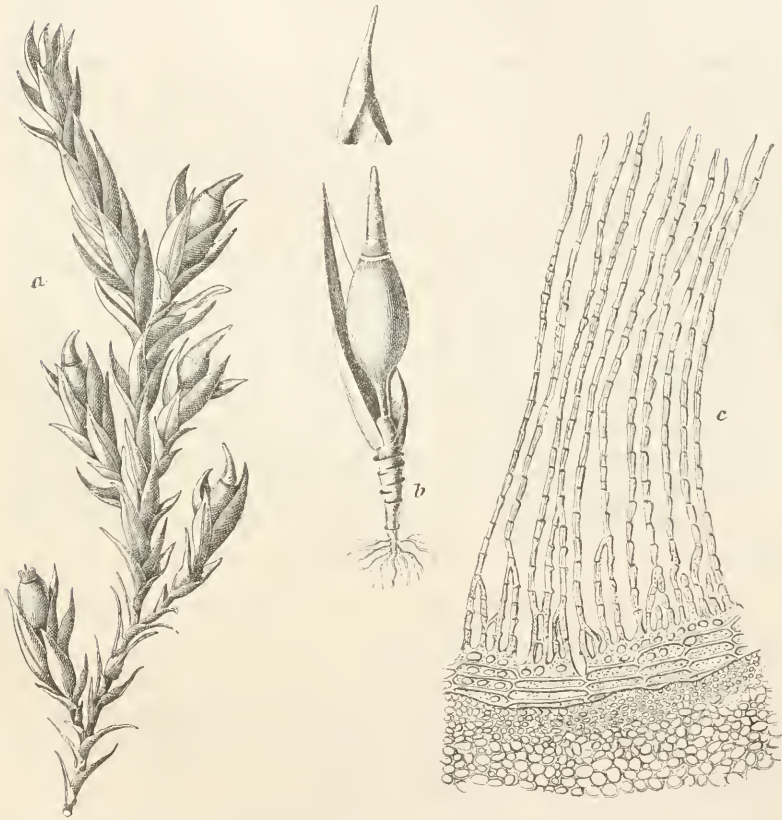
Cinclidotus fontinaloides (Hedw.). Habitusbild \frac{1}{4} , Fruchtabzweig mit Sporogon und dem innersten Hüllblatte \frac{8}{4} , Peristom \frac{100}{1} .
