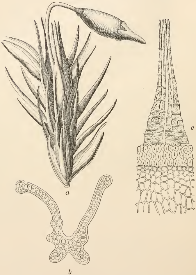
Dryptodon patens . a Habitusbild 4\frac{2}{1} , b Blattquerschnitt 3\frac{2}{1}\frac{5}{1} , c Peristom und Ring 2\frac{0}{1}\frac{0}{1} .
