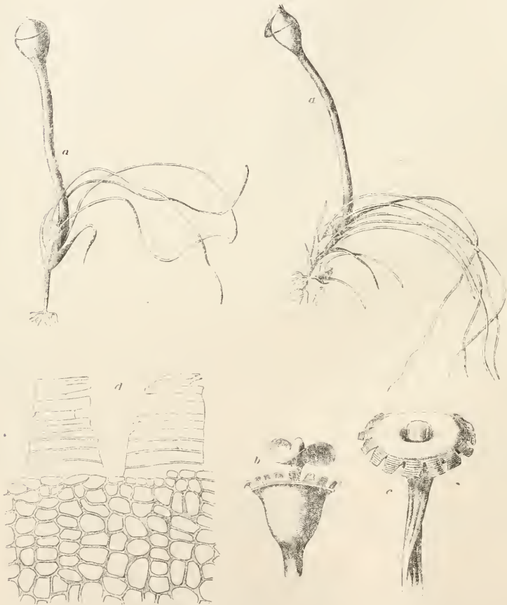
Trochobryum carniolicum Breidl. & Beck. a Zwei Habitusbilder \frac{1}{4} . b Kapsel mit emporgehobenem Deckel \frac{3}{1} , c alte Kapsel \frac{3}{1} , zwei Peristom- zähne \frac{2}{1} \frac{8}{1} .
