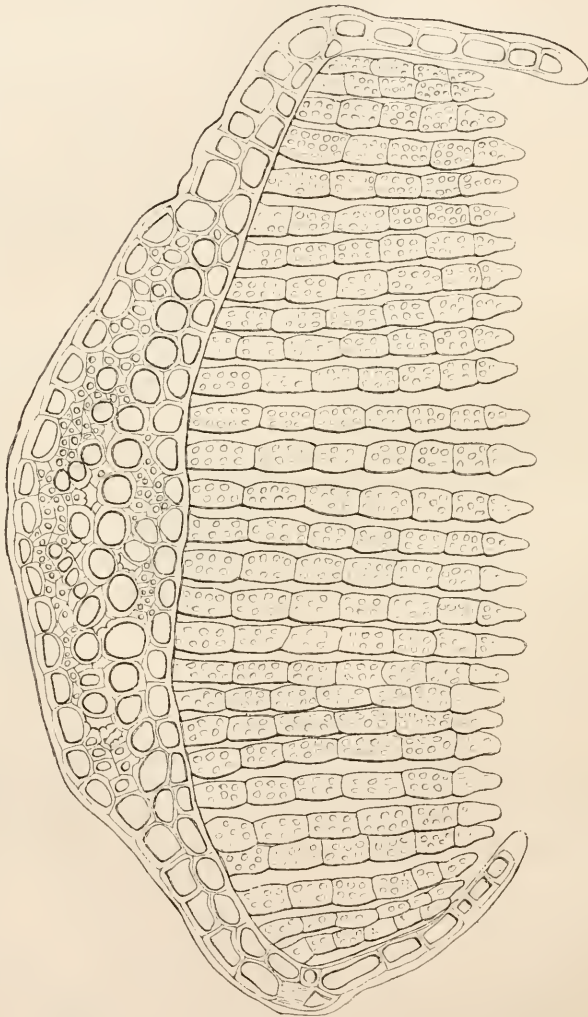
Blattquerschnitt und Lamellenbildung von Polypodium sexangulare Flörke. Vergr. 400.
