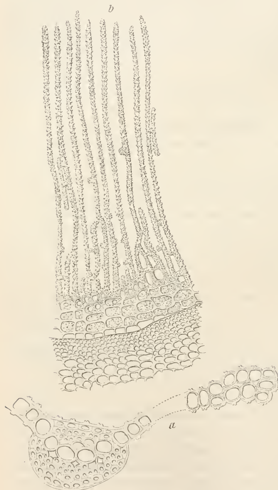
Dialytrichia Brébissoni . a Theil eines Blattquerschnittes, b Peristom \frac{1}{100} .
