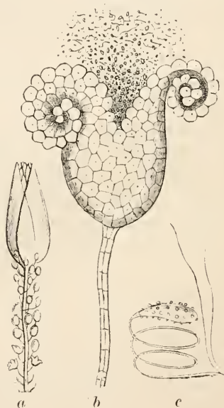
a Die Spitze eines zum Theil entblätternen ♂ Astes, b ein geöffnetes Antheridium und c ein Spermatozoid von Sphagnum : alle Figuren nach Schimper.
