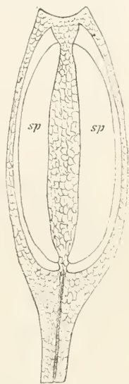
Längsschnitt durch die entdeckte Kapsel von Hymenostomum squarrosum Bryol. germ. Zellnetz schematisch. sp. Sporenraum. \frac{1}{2} .
