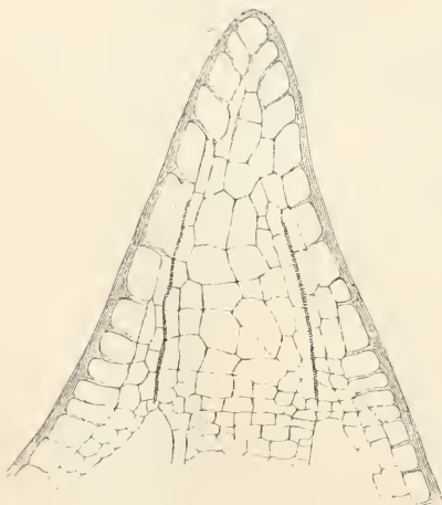
Fig. 72. Längsschnitt durch den Kapseldeckel von Mildeella bryoides 189 .
