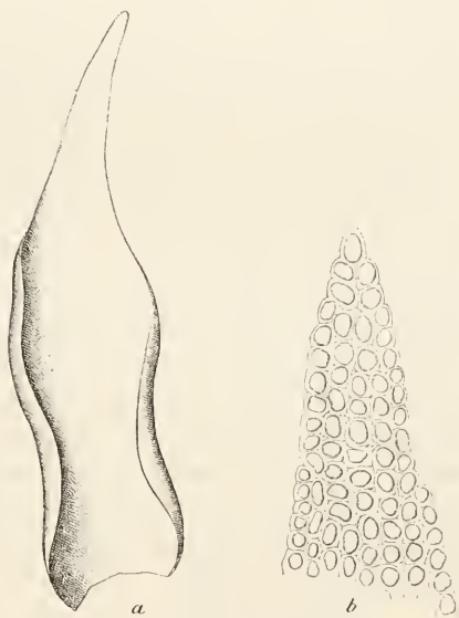
Andreaea sparsifolia Zett. a Laubblatt ( \frac{8.0}{1} ). b Spitze eines Laubblattes ( \frac{2.8.0}{1} ).
