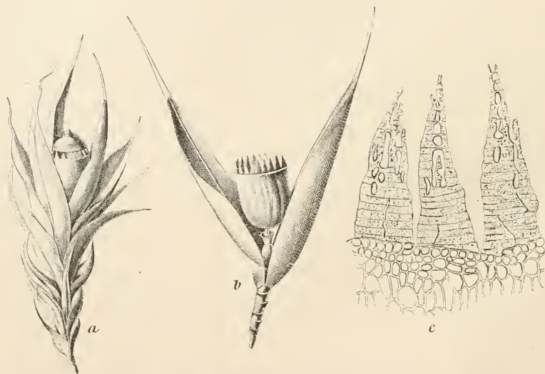
Grimmia triformis De Not. a Habitusbild \frac{1}{1} , b entleerte Kapsel \frac{1}{1} , c drei Peristomzähne \frac{1}{1} .
