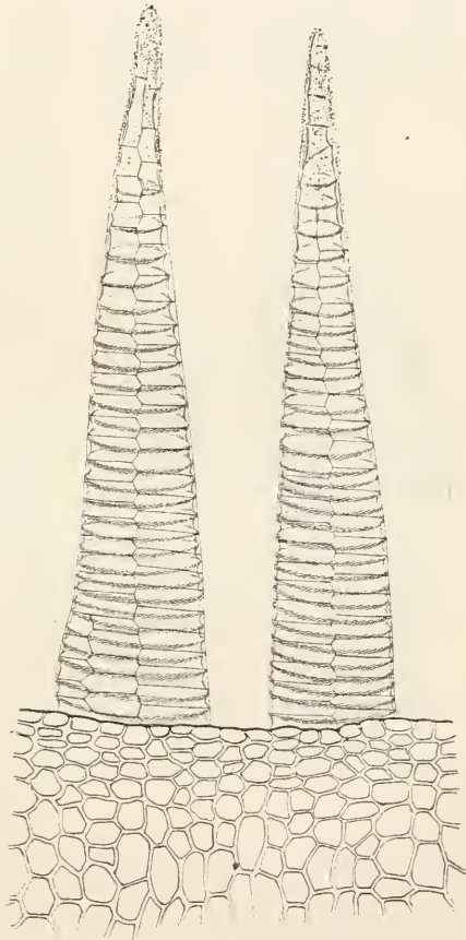
Zwei Zähne des äusseren Peristoms von Mnium medium Br. eur. von der Aussenfläche mit den durchleuchtenden Lamellen der Innenfläche. Vergr. \frac{1}{4} \frac{2}{1} \frac{5}{1} .
