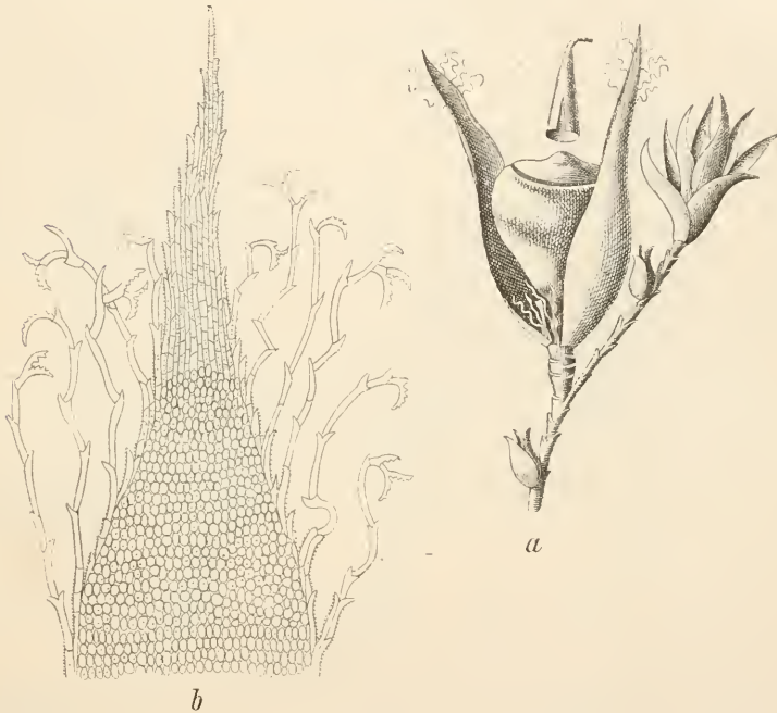
Hedwigia albicans . a Habitusbild (Sporogon, Haube, 2 innere Hüllblätter und 2 ♂ Blüthen) \frac{1}{1} , b Spitze eines Perichätialblattes \frac{5}{1} .
