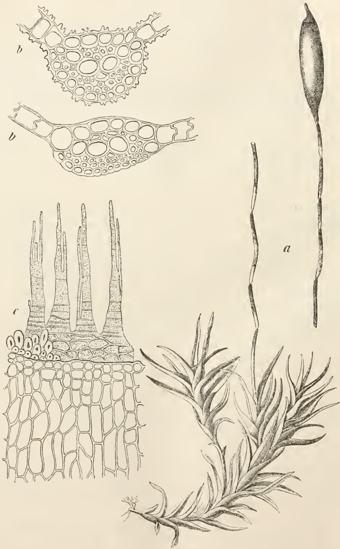
Didymodon rubellus (Hoffm.). a Habitusbild \frac{4.5}{4} , b zwei Querschnitte durch die Blattrippe \frac{3.50}{4} , c Peristom \frac{4.50}{4} (die Zellenzüge der Grundhaut gehören der Innenschicht an).
