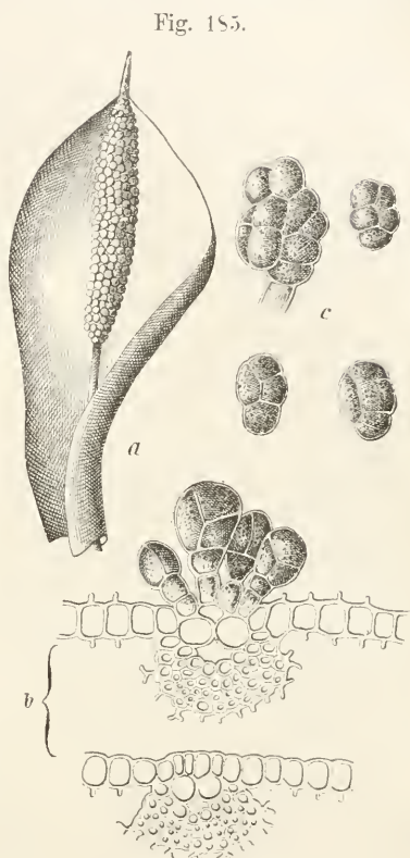
Fig. 185. Tortula papillosa Wils. a Blatt mit Brutkörpern \frac{2}{1} , b Rippe mit und ohne Brutkörper \frac{1}{1} , c einzelne Brutkörper \frac{1}{1} .
