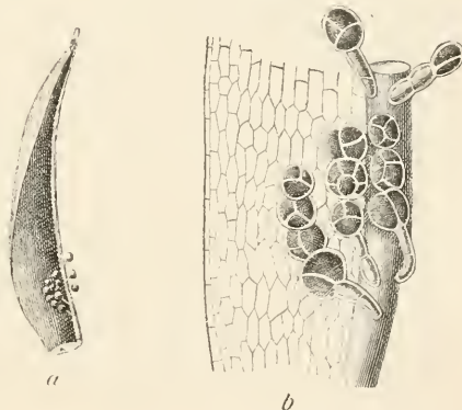
Grimmia torquata (Hornsch.). a Laubblatt \frac{3}{1} , b Blattgrund mit Brutkörpern \frac{12}{4} .
