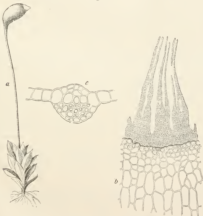
Desmatodon cernuus (Hüben.). a Habitusbild \frac{1}{10} , b Peristom \frac{17}{3} , c Blattrippe im Querschnitt \frac{28}{1} .
