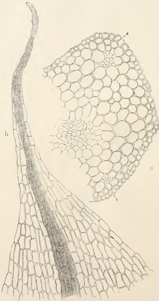
Voitia nivalis Hornsch. a Theil eines Stengelquerschnittes mit Centralstrang und 2 Blattspursträngen (bei \uparrow ) \frac{2.2}{1.0} . b Zellnetz der Blattspitze \frac{1.8}{1.3} .
