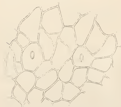
Zwei schildförmige Spaltöffnungen von Physcomitrella ( \frac{3}{1} \frac{6}{1} ).
