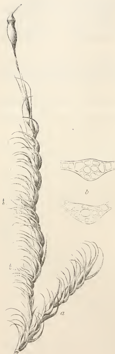
Dieranum fulvellum (Dicks.). a Habitusbild \frac{1}{10} , b zwei Querschnitte durch die Rippe \frac{1}{100} .
