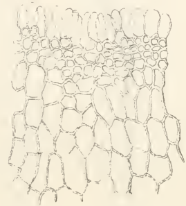
Ein Theil des Urnenrandes mit den Ringzellen von Gyroweisia tenuis (Schr.) \frac{1}{2} a.
