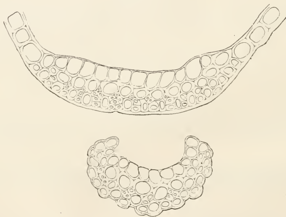
Campylopus turfaceous Bryol. eur. Zwei Blattquerschnitte \frac{1}{4} 0.0.
