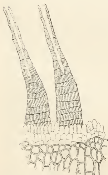
Cynodontium polycarpum (Ehrh.). Peristomzähne (Aussenfläche) und Ringzellen ( \frac{180}{1} ).
