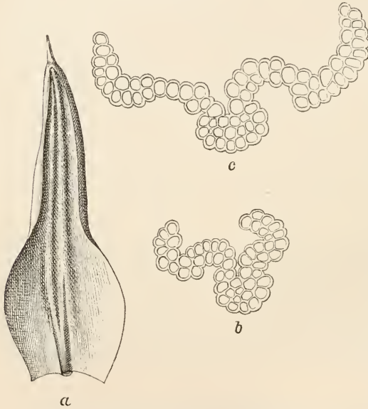
Grimmia caespiticia . a Laubblatt \frac{5.0}{1} , b und c Blattquerschnitte \frac{2.5.0}{1} .
