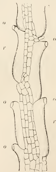
Retortenzellen (r) der Astrinde von Sphagnum molluscum . Bruch: bei o deren Oeffnung.
