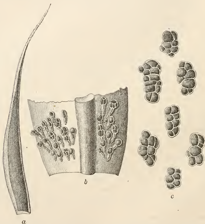
Grimmia trichophylla propagulifera. a Laubblatt \frac{3}{1} \frac{3}{1} , b Blattgrund mit Brutkörpern \frac{1}{1} \frac{2}{1} \frac{5}{1} , c einige entwickelte Brutkörper \frac{2}{1} \frac{2}{1} \frac{0}{1} .
