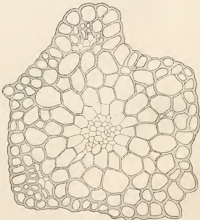
Stengelquerschnitt von Bryum turbinatum nach P. G. Lorentz; oben und links unten falsche Blattspuren (s. pag. 25). Vergr. ca. \frac{320}{1} .
