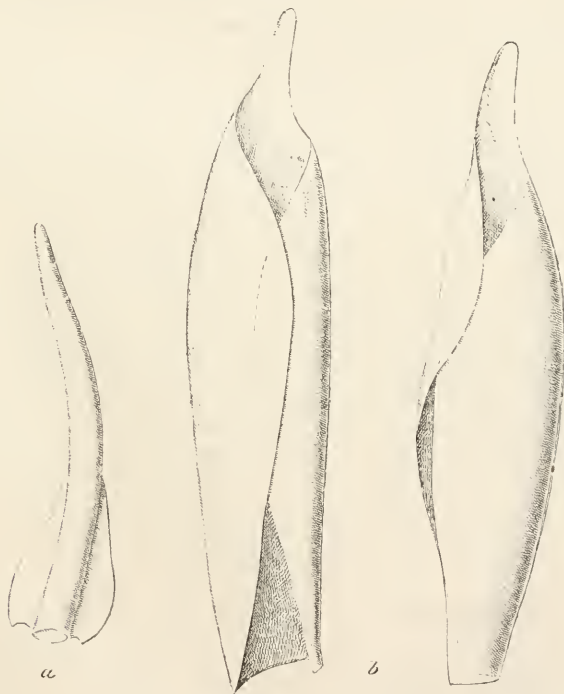
Andreaea crassinervia Bruch. 57. 1 a Laubblatt. b die beiden inneren Perichätialblätter.
