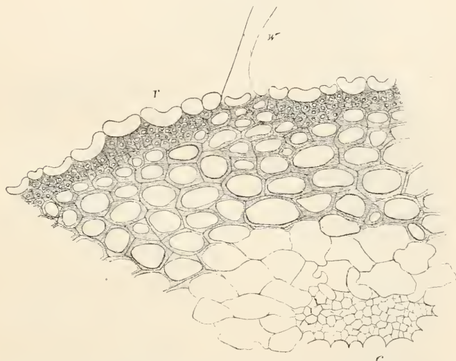
Theil eines Querschnittes durch ein Stämmchen von Bretelia arcuata : c Centralstrang, r Aussenrinde, w Wurzelhaar. Vergr. \frac{280}{1} .
