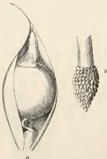
Phascum cuspidatum var. \epsilon .
