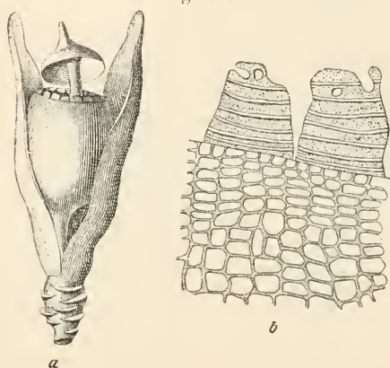
Schistidium atrofusum (Schimp.). a Sporogon und zwei Hüllblätter \frac{2}{1} , b Peristom \frac{1}{1} \frac{2}{1} \frac{5}{1} .
