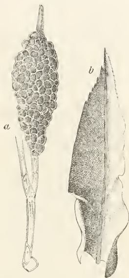
Barbula paludosa Schleich. a Stengelbürtiger Brutkörper \frac{1}{100} , b Laubblatt \frac{3}{10} .
