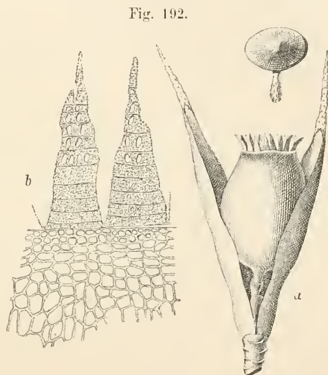
Schistidium brunnescens nov. spec. a Sporogon mit zwei Hüllblättern und dem abgefallenen Deckel, b Peristom ( 1\frac{2}{3} ).
