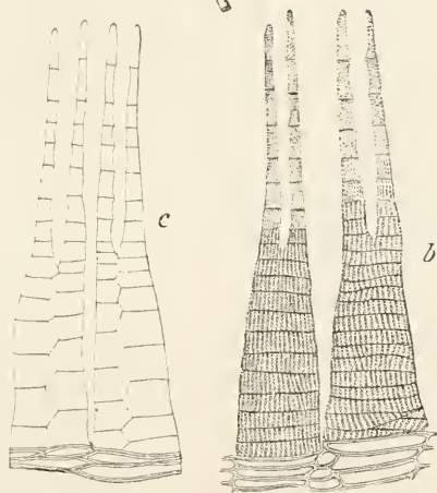
Cynodontium strumiferum (Ehrh.). a Kapsel mit kropfigem Hals ( \frac{15}{1} ), b Aussenfläche und c Innenfläche der Peristomzähne ( \frac{180}{1} ).
