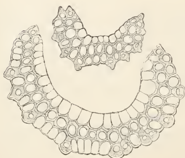
Dicranum longifolium Ehrh. Zwei Querschnitte durch den Pfriementheil des Blattes \frac{280}{1} .
