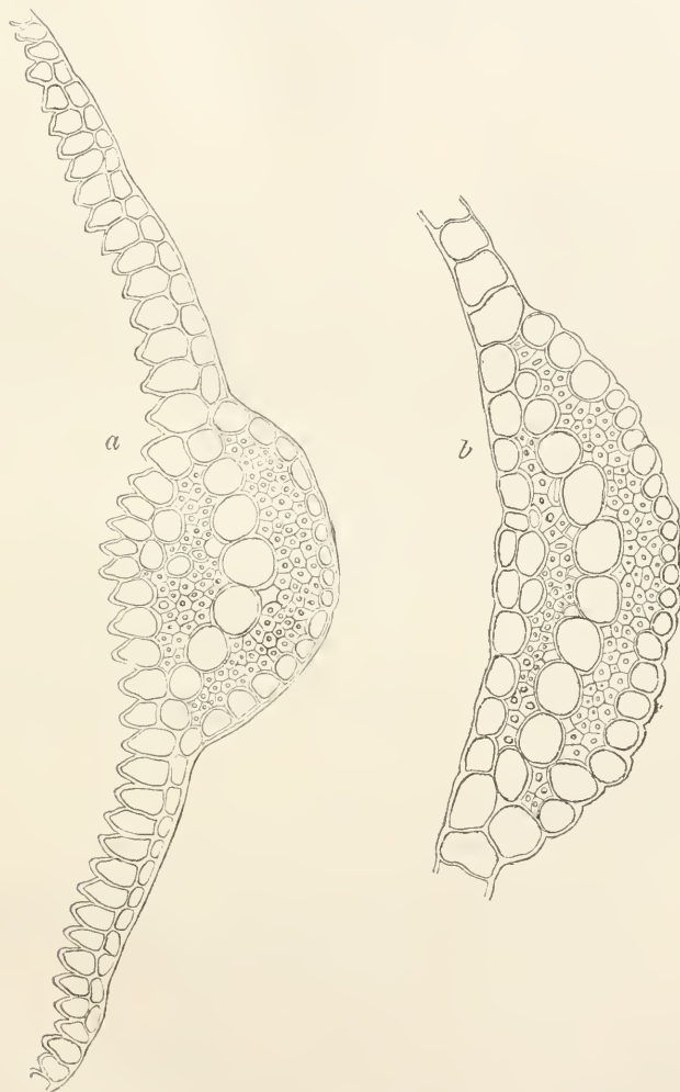
Timmiella anomala (Bryol. eur.). Querschnitte: a durch die Blattmitte, b durch die basale Blattrippe \frac{1}{100} .
