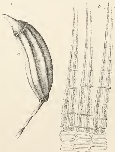
Ceratodon purpureus (L.).
