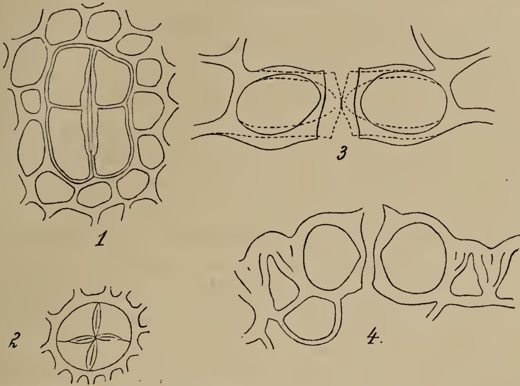
Abb. 2. Spaltöffnungen von Bryophyten. 1. Vierlingsspaltöffnung von Polytrichum juniperinum (nach H a b e r l a n d t). 2. Desgleichen (nach B ü n g e r). 3. Querschnitt durch die Spaltöffnung von Hypnum cuspidatum (nach B ü n g e r). 4. Desgleichen von Anthoceros punctatus (nach C o p e l a n d).
