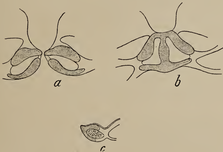
Abb. 4. a—b Larix (nach Mahler). a) medianer, b) polarer Querschnitt, c) Todea barbara medianer Querschnitt (nach Vinge).
