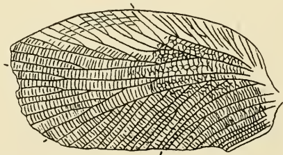
Fig. 2. Archimylacris Desaillyi Leriche \times 3\frac{1}{2} . (Nach Leriche.)
