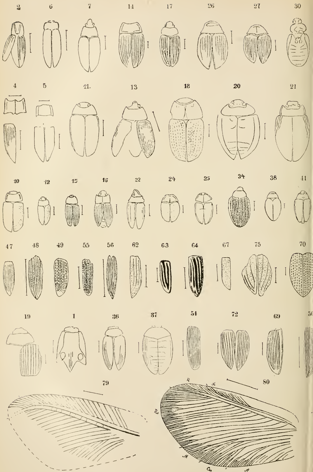
Lias-Insekten: Coleoptera (1-77) = Neuroptera (78-84).
