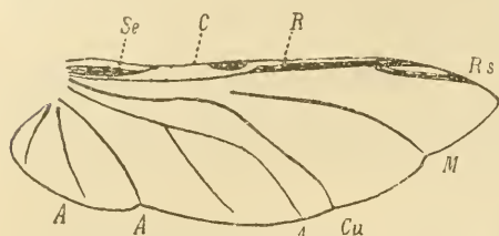
Fig. 2. Hinterflügel von Necrophorus . (Staphylinidentypus.)
