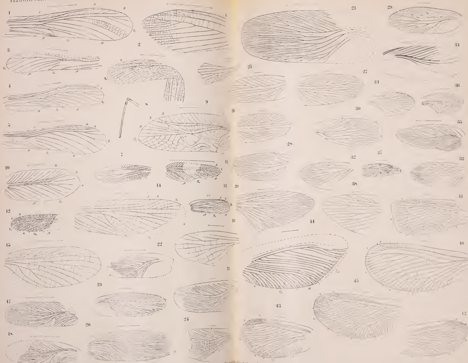
Lias-Insekten: Locustoidae (1-10) - Mantodea (11-16) - Blattodea (17-39) - Neuroptera (40-45).
