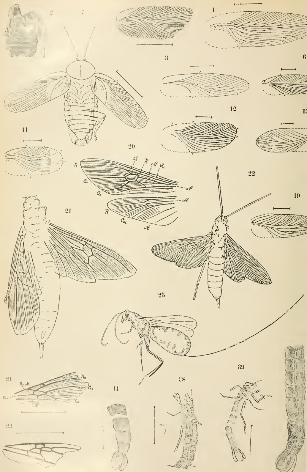
Jura Insecten: Blattoidea (1-19) — Hymenoptera (20-25) — Plectoptera (26-33) —
