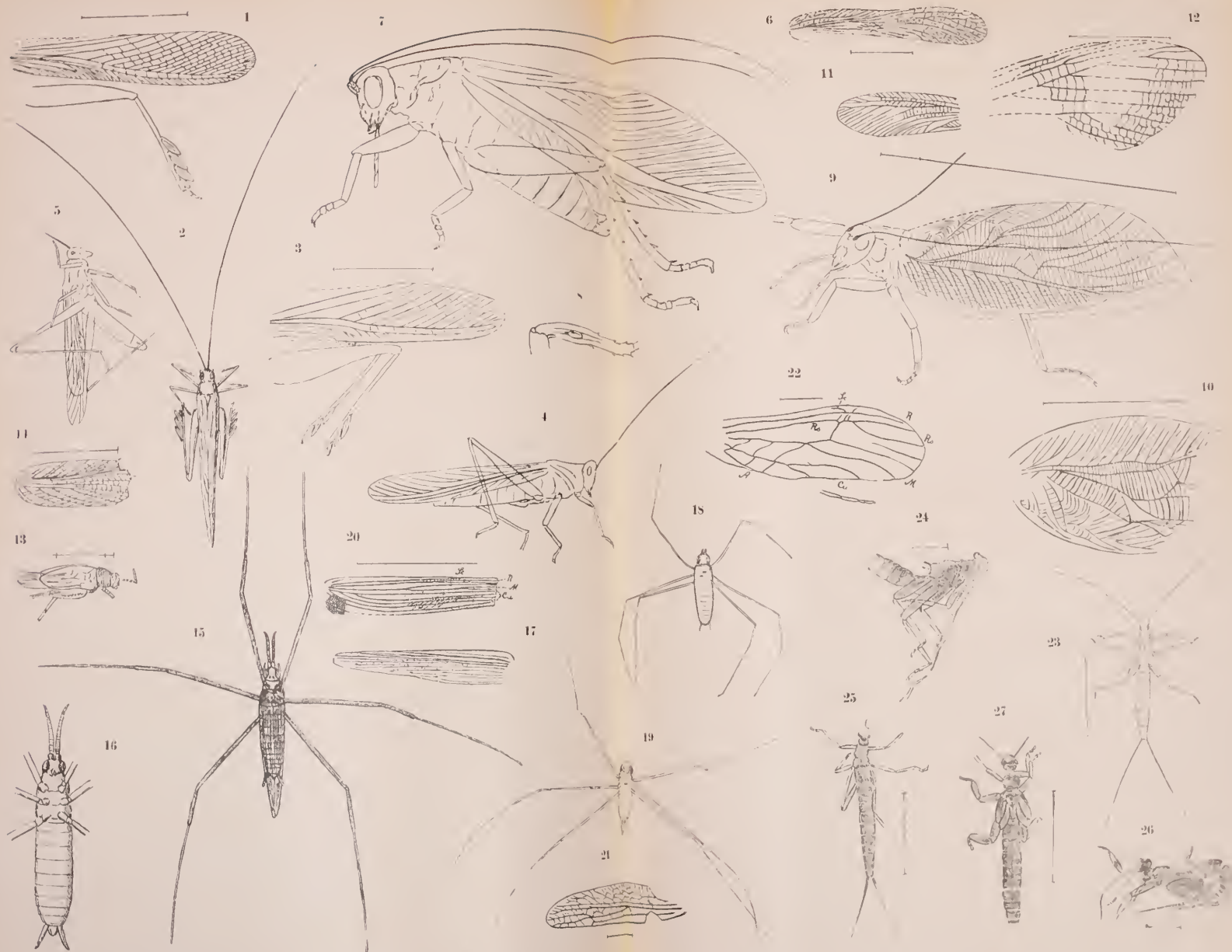
Jura-Insekten: Locustoida (1-14) — Phasmoidea (15-21) — Perlaria (22-27).
