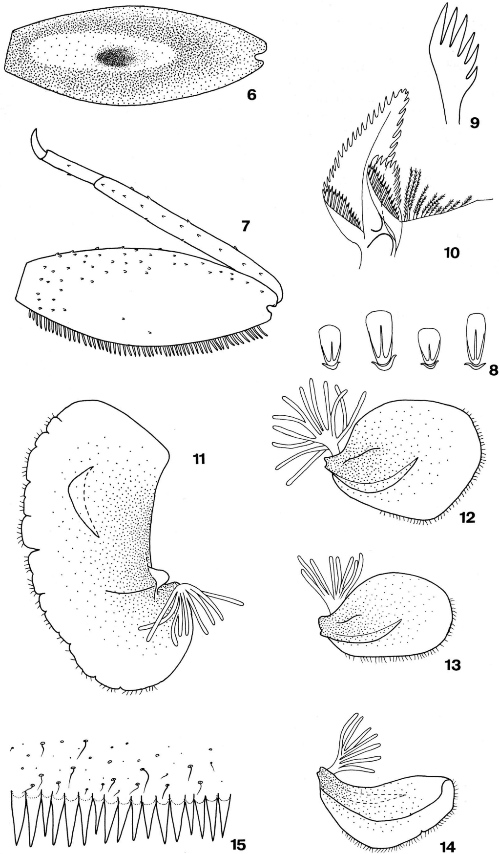
Figures 6-15. – Rhithrogena carpatoalpina sp. n., larve: 6. Dessin de la face supérieure des fémurs postérieurs; 7. Patte postérieure; 8. Epines de la partie centrale des fémurs postérieurs; 9. Peigne de la partie distale de la lacinia maxillaire; 10. Partie de la mandibule droite en vue ventrale; 11, 12, 13, 14. Première, deuxième, sixième et septième branchie; 15. Partie centrale du cinquième tergite abdominal.
