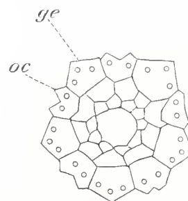
Apicalpol von Palaeochinus elegans nach Zittel's Lehrbuch.
