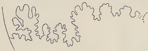
Fig. 26. Lobenlinie von Hoplitoides Wohltmanni v. K. Elephantenbank am Mungo (Stück II der Tabelle). a) bei 5 mm Windungsradius. 10/l. b) Rechte Sutura bei 30 mm Windungsradius. 2/l. c) Erster linker Lateral bei 30 mm Windungsradius. 2/l.
