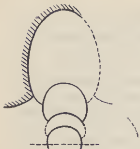
Fig. 24. Querschnitt der Jugendwindungen von Hoplitoides Wohltmanni v. K. Elephantenbank (Stück II der Tabelle). 10/l.
