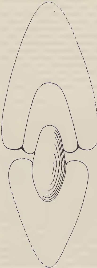
Fig. 8. Querschnitt eines erwachsenen Neopt. telingae n. sp. (von dem auf Taf. III Fig. 2–4) abgebildeten Exemplar). Nat. Gr.
