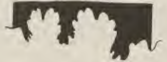
Fig. 4. Lobenlinie von Bac. cf. grac. St. vom Mungoufer unterhalb Balangi. 4/1.
