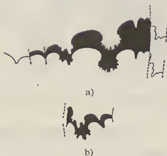
Fig. 51. Linke Sutura bei 18 mm Windungsradius. 2/1. a) Äußere Loben. b) Innenloben.
