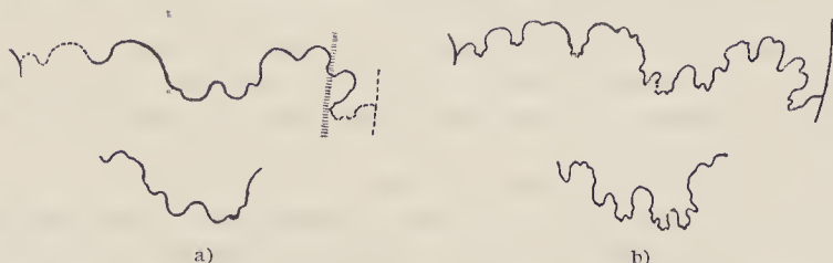
Fig. 42. Lobenlinie von Hopl. Koeneni n. sp. Elefantbank am Mungo. (Stück I der Maßstabelle.) a) Linke Suture und erster Laterallobus der rechten Suture bei 4 mm Windungsradius. 10/1. b) Desgl. bei 23 mm Windungsradius. 2/1.
