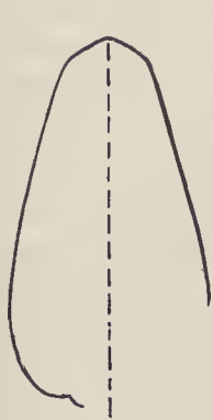
Fig. 59. Äußere Windung. 2/l.
