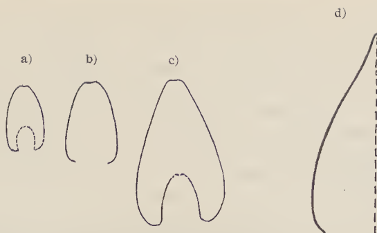
Fig. 28. Querschnitt verschiedener Windungen von Hopl. ingens nodifer . a—c) 2/1. d) Nat. Gr.
