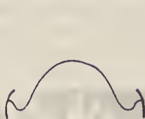
Fig. 60. Embryonalkammer von Barr. Haberfellneri var. Harléi. 40/l.
