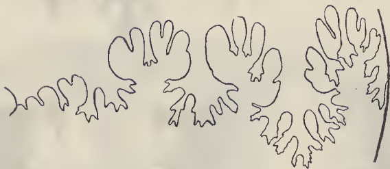
Fig. 20. Lobenlinie eines Neopt. telingacif. n. sp. (Göttinger Universitätssammlung), 1/1.
