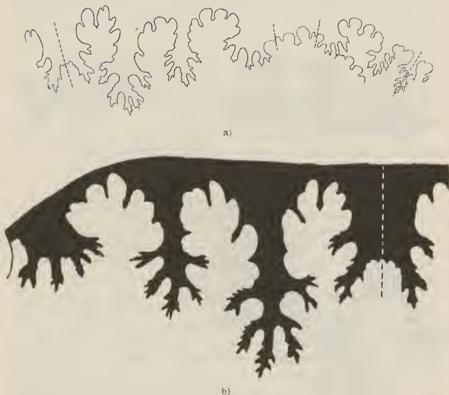
Fig. 18. Lobenlinie von Neopt. crassus n. sp. von Balangi. a) rechte Suture einschließlich der Innenloben bei 35 mm Windungsradius, 3/2 . b) linke Suture bei 40 mm Windungsradius, 2/1 .
