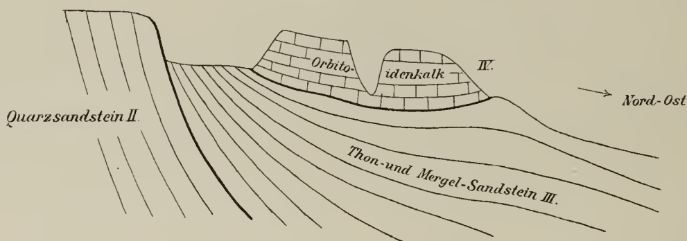
Profil der Eocän-Schichten bei Batoe Mendjoeloer, Hochland von Padang, Sumatra.
