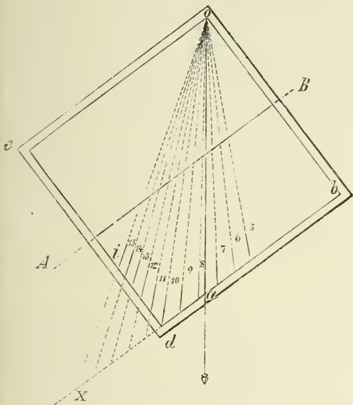
Fig. 435. Meßbrettchen von Smalian.
