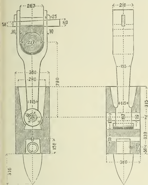
Fig. 462. Querschnitte des Spaltkeiles einer Holzspaltmaschine.
