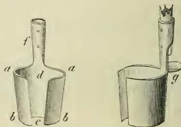
Fig. 453. C. Heyers Hohlbohrer. — a a oberer Rand. bei großen Bohrern 14 5/8—15 5/8 cm, bei kleinen 4 5/8 cm weit; b b unterer Rand, bei großen Bohrern 12—13 cm, bei kleinen 4 cm weit; a b als Höhe, ebensoviel Centimeter als a a enthält; c d offener Spalt (etwa 4 cm breit); f Stielhülse; g Eisenplättchen, bis zu welchem der Bohrer jedesmal beim Gebrauche in die Erde gedrückt wird.
