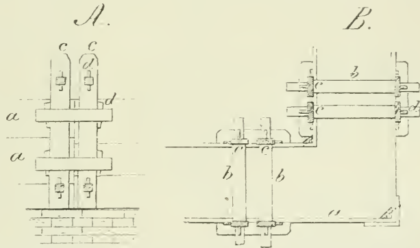
Fig. 487. Seitenansicht A und Grundriß B einer Wandform für Kalksandpfeismauern. a Wandbohlen, b Riegelholzer, c Leistenholzer, d Holzsteile.
