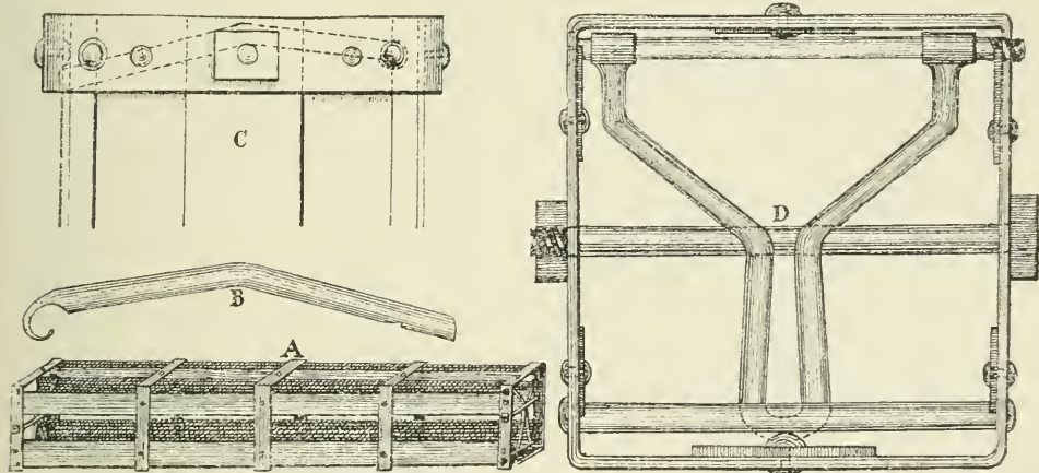
Fig. 452. Eiserne Hohlfalle von A. Freiherrn v. Hausstein. — A Totalansicht, B Abzughebel, C Ansicht eines Bandes von oben, D Eingang der Falle.
