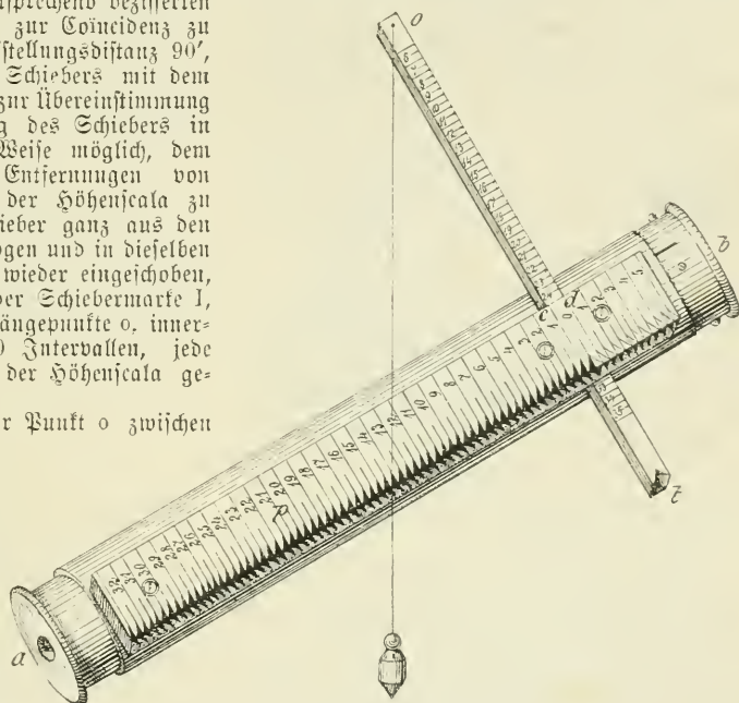
Fig. 444. Der Weisse'sche Höhenmesser.
