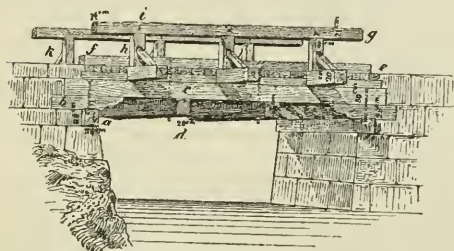
Fig. 454. Ansicht einer Balkenbrücke. a Mauerlatten oder Mauerbänke, b Sattelhölzer, c Brückenbalken (Streckbalken, Dohlbäume), d Durch- oder Unterzüge, e Bohlenüberlag (Brückenstreu), f Saumschwellen, g Geländer, h Geländerpfosten, i Geländerholm, k Geländerstreben.
