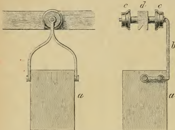
Fig. 414. Transportkästen der Trahfseilriehe, System Hodgson. — a Tragkästen, b Tragstange, c Räder von Eisen, d Sattel von Holz.
