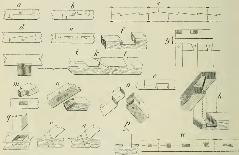
Fig. 461. Holzverbindungen. a Einfache oder gerade, b schiefe, c einfach verzahnte, d schiefe verzahnte, e doppelt verzahnte Überblattung, f Schaffhausen'sches Schloß, g vollkommene Überblattung, h schwalbenschweifsförmige Überblattung, i einfacher, k kreuz-, l schwalbenschweifsförmiger Mann, m einfacher, n schiefer, o Scheers-, p schwalbenschweifsförmiger Zapfen, q gerade, r schiefe, s doppelte Einlassung, t Verzäpfung, u Verdöbelung.
