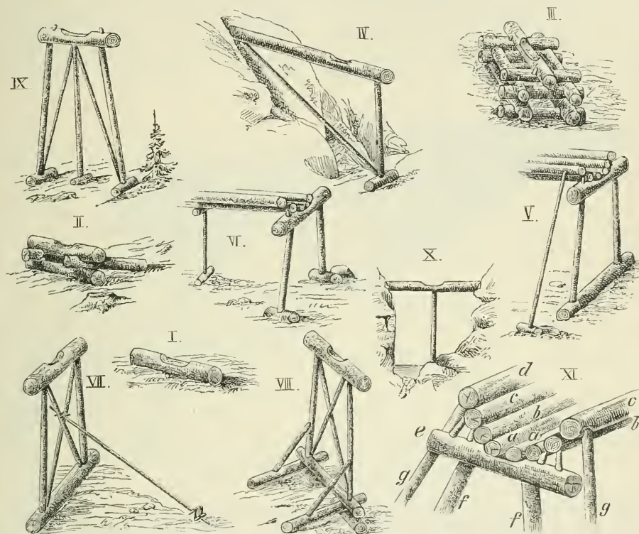
Fig. 457. I. Rothjoch, II. Legjoch, III. Kastenjoch, IV. Bergjoch, V. und VI. Hochjoch, VII. und VIII. Kreuzjoch, IX. Kralljoch, X. Hundjoch, XI. Überfattelte Stangenrieße: a Bodenbäume, b Wehren, c Sattel, d Überfattelholzer, e Jochdrehling, f Jochstützen, g Sattelstrecken.
