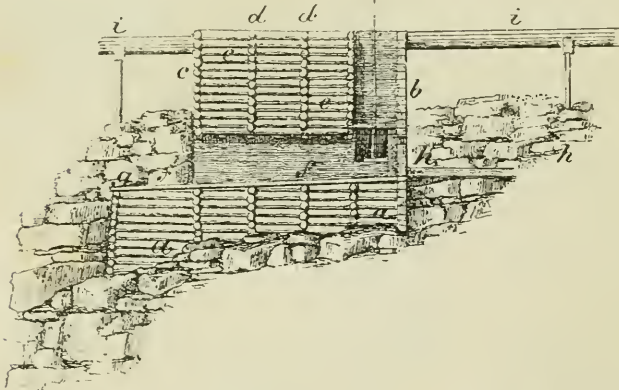
Fig. 499. Querschnitt einer Steinkastenklaufe. a Fundamentbau, b Krainerwand, Rückwand, d Mittelwände, e Einschloß- oder Querwände, f Wasserablaßcanal, g Vorfeld, h Klaushof, i Wasserrieße.
