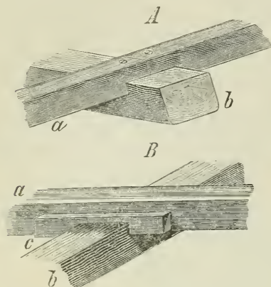
Fig. 459. A Verbindung von Längs- und Querschwellen (a und b) durch Überblattung und Nagelung. — B Verbindung von Längs- und Querschwellen (a und b) durch Überblattung und vorgegeschlagene Keilhölzer c.
