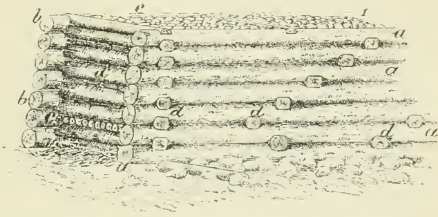
Fig. 500. Ansicht einer Kästen- oder Doppelwehr (Uferschutzbau). a Wasserwandbalken, b Rückwandbalken, c Schwebbodenbölzer, d Zinschloßhölzer (Zangen), e f Ausgeschwüre.
