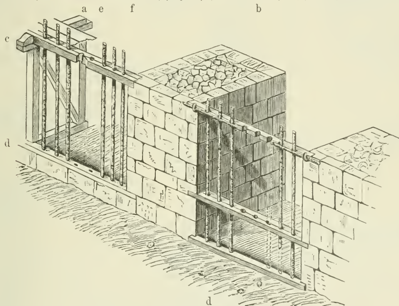
Fig. 456. a Rechenjoch, b Rechenpfeiler, c Streckbaum oder Spindelbaum, d unterer Spindelbaum, e Laufbretter f Rechenzähne, Spindeln oder Sperrhölzer.
