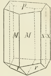
Fig. 464. Hornblende. Zwillingstrypit nach ∞ P ∞
