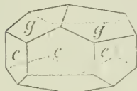
Fig. 488. c = \infty R ; g = -\frac{1}{2}R
