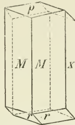
Fig. 463. Hornblende oP (P); P (r) ∞ P (M); ∞ P ∞ (X).
