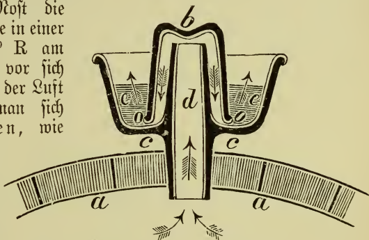
Fig. 306. Rheinischer Gärspunden aus Thon.
