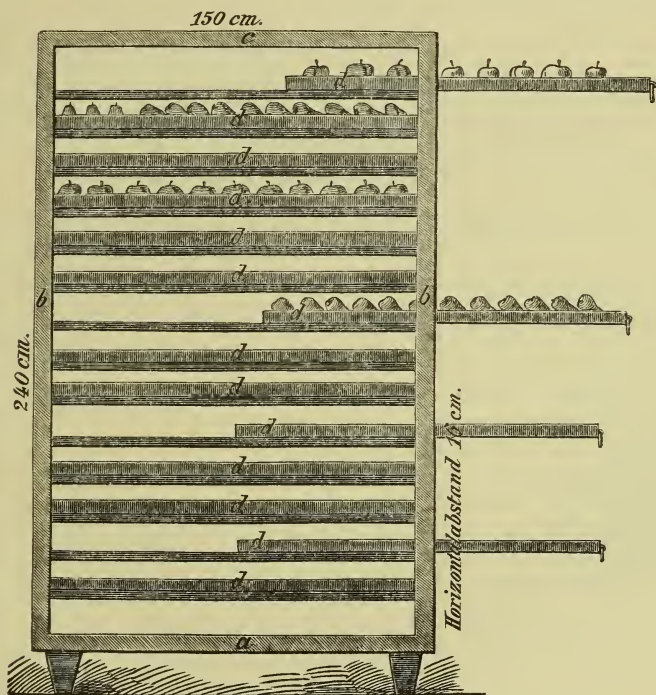
Fig. 273. Obstschrank zum Aufbewahren des Winterobstes.
