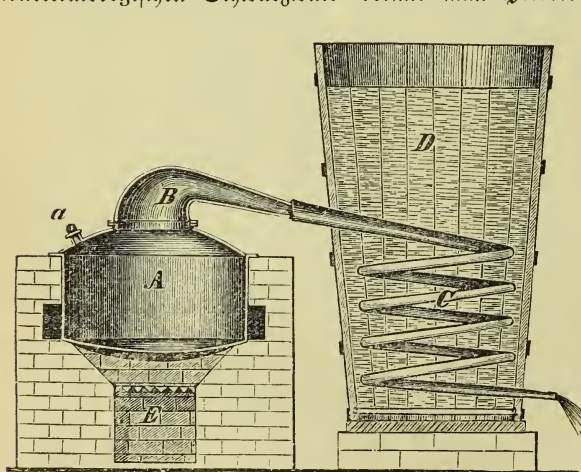
Fig. 314. Destillierapparat.
