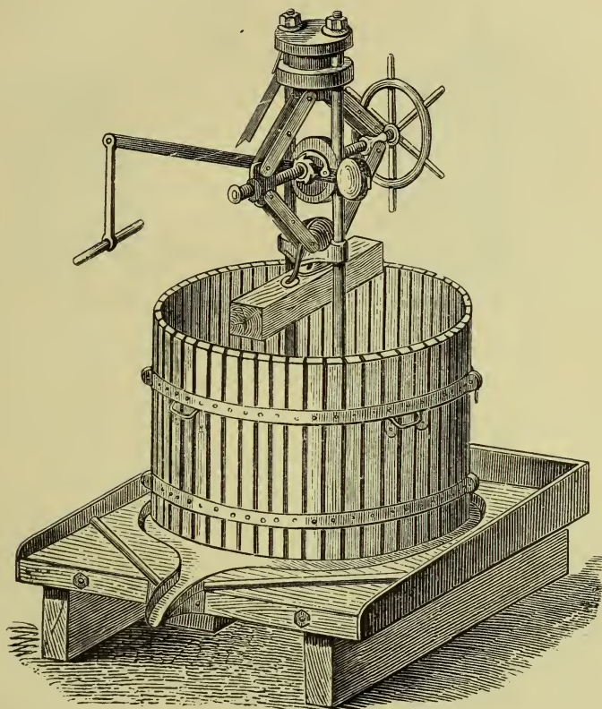
Fig. 302. Kniehebelpresse.
