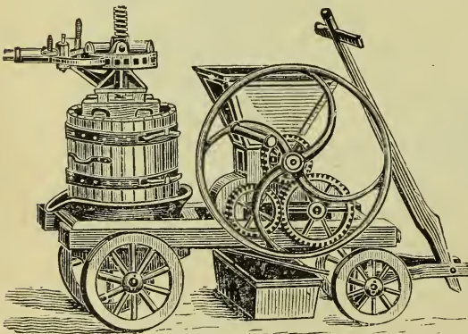
Fig. 305. Fahrbare Obstmühle und Presse von Bleßing und Botteler in Reutlingen.
