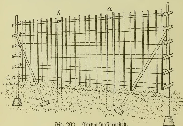
Fig. 262. Cordonspaliergestell.
