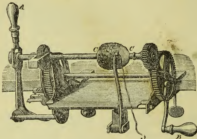
Fig. 292. Schälmaschine „Unikum Nr. 4“ mit einem Messer.
