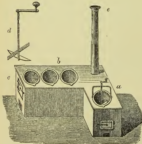
Fig. 316. In Böhmen gebräuchlicher Doppelherd zum Einkochen des „Povidel“.
