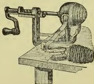
Fig. 291. Schälmaschine „Penn 1885“.
