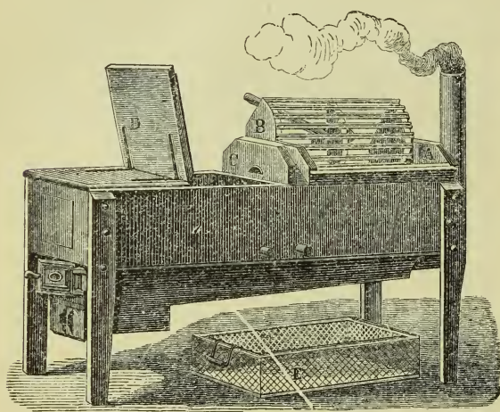
Fig. 320. Amerikanischer Herd zum Dämpfen, Einkochen u. s. w.
