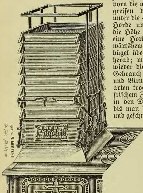
Fig. 298. Geisenheimer Herddörre von R. Mertens.
