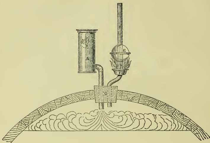
Fig. 310. Apparat zum Einschwefeln.
