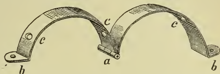
Fig. 112. Geöffneter Eisenreif zum Schutzgestell Fig. 111.
