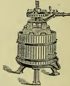
Fig. 304. Verbesserte Spindelpresse mit eisernem Biet.
