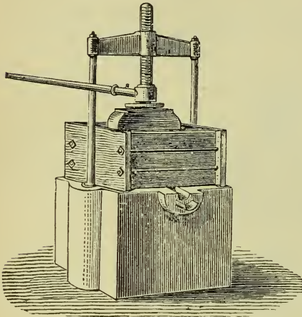
Fig. 303. Gewöhnliche Spindelpresse mit steinernem Biet.
