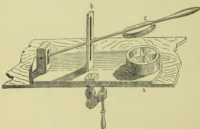
Fig. 287. Obstschneidemaschine.
