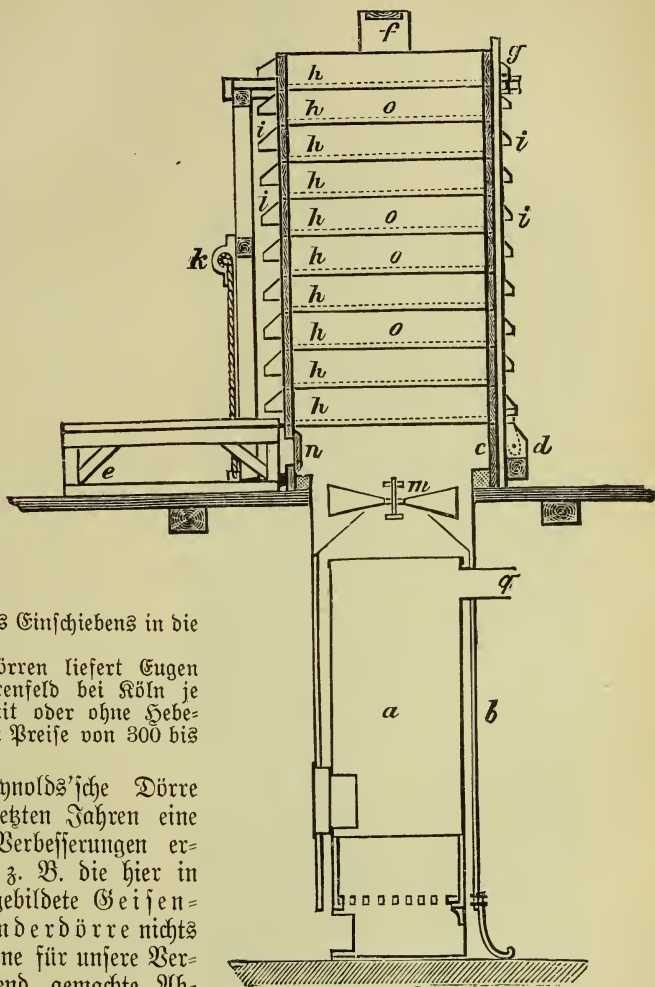
Fig. 296. Reynolds' Dörreapparat.
