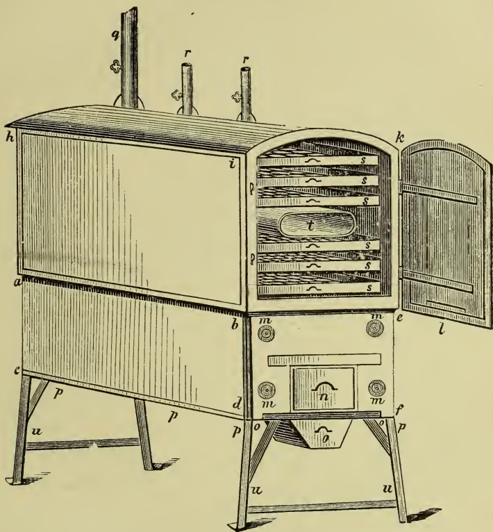
Fig. 295. Lucas'sche Wanderdörre.
