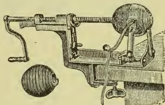
Fig. 290. Schälmaschine „Penn 1883“.
