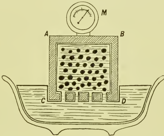
Schema eines Versuchs über osmotischen Druck. CD eine halbdurchlässige Wand. M Manometer.
