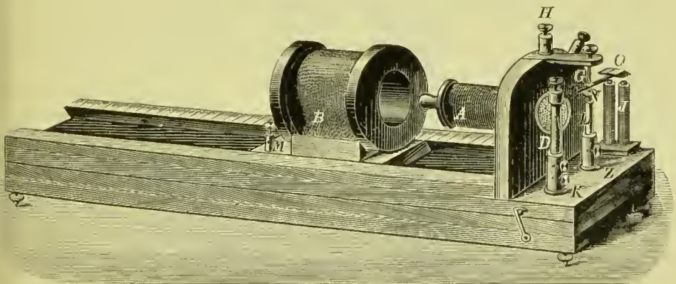
Schlitteninductorium von E. du Bois-Reymond.
