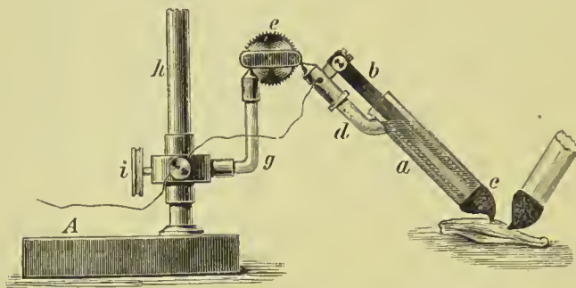
Unpolarisirebare Elektrode.
