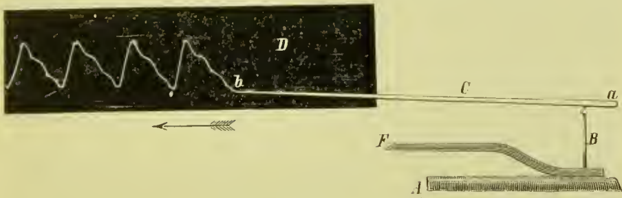
Schema des Sphygmographen von Marey.
