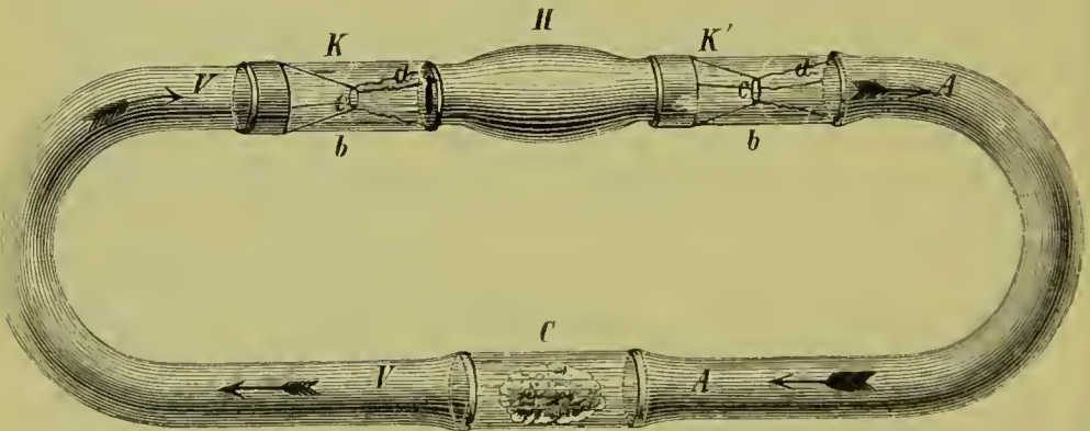
Schema des Kreislaufs nach E. H. Weber.
