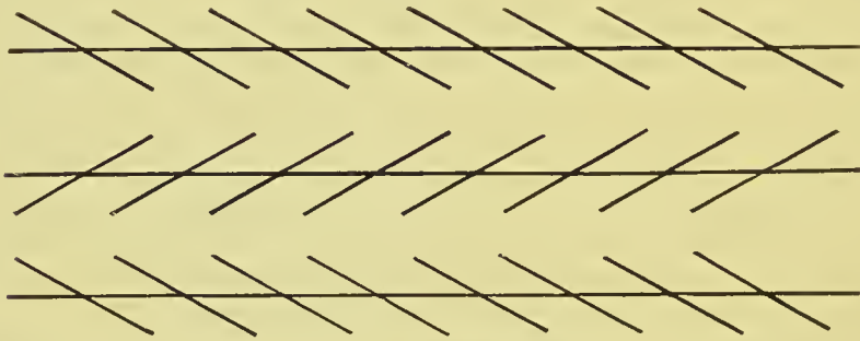
Zöllner's Liniensysteme.
