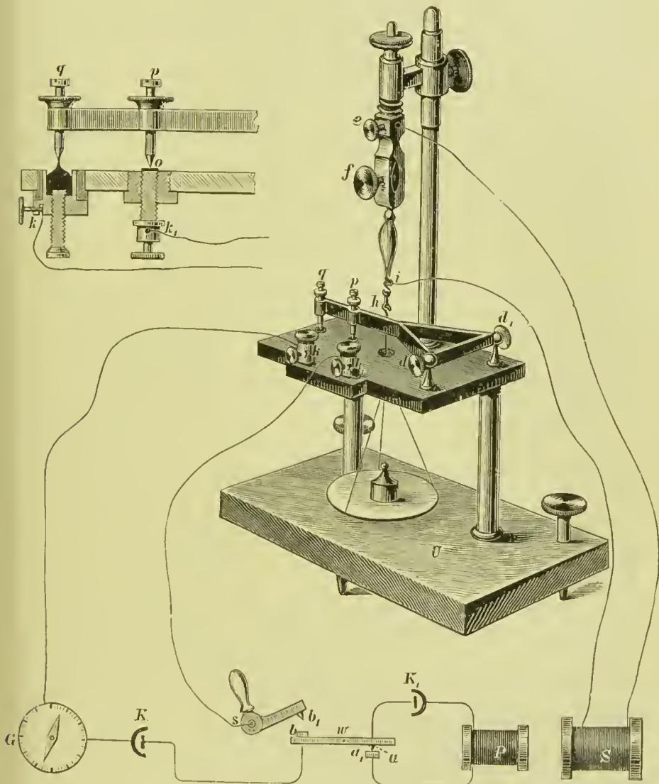
Froschunterbrecher. (Die am unteren Rand der Figur dargestellte Anordnung bezieht sich auf einen in einem weiter unten folgenden Abschnitt zu besprechenden Versuch.)
