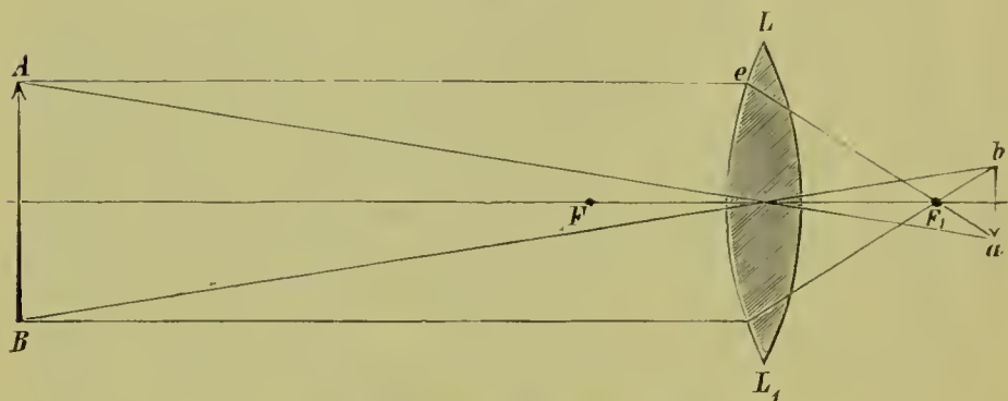
Gang der Lichtstrahlen durch eine Sammellinse.
