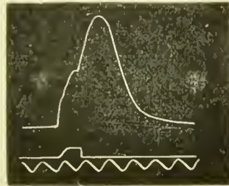
Summation von 2 Reizen, Intervall \frac{1}{50} Secunde.
