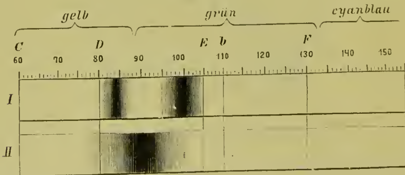
Absorptionsbänder des Oxyhämoglobins (I) und des reduzierten Hämoglobins (II).
