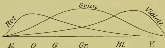
Schematische Darstellung der Erregbarkeit der Netzhaut durch die Grundfarben (nach Helmholtz).
