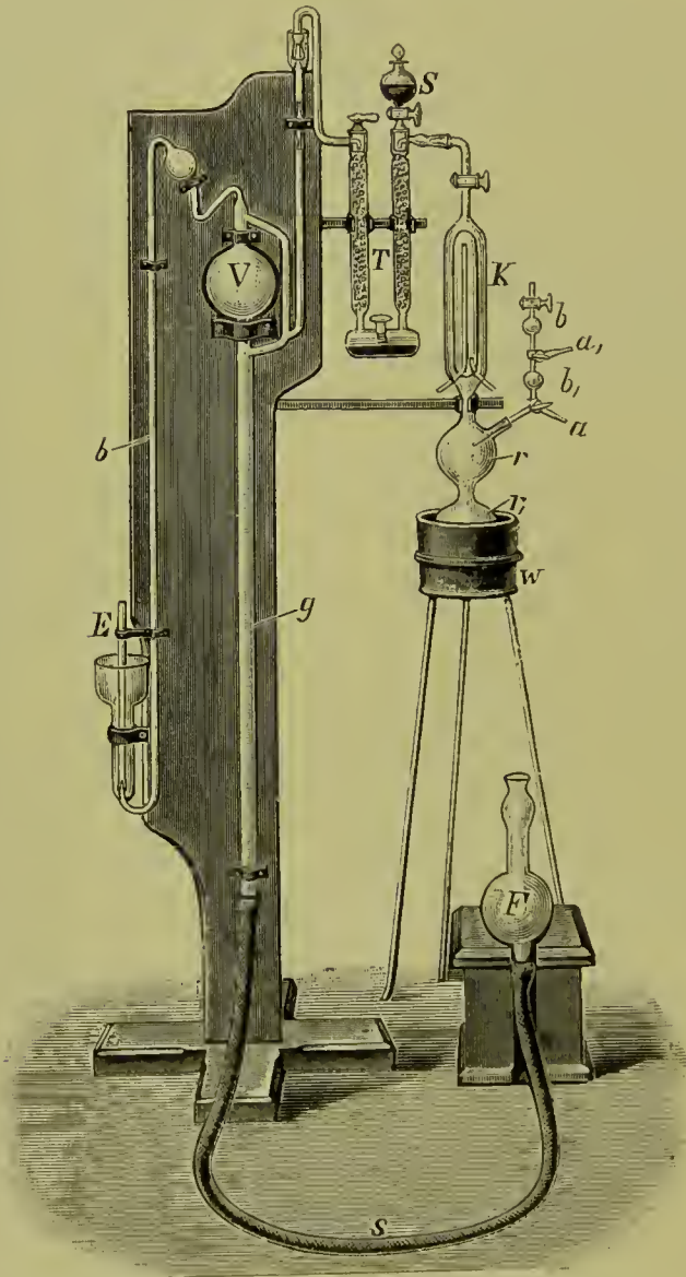
Blutgaspumpe nach Töpler-Hagen, modificirt von Zuntz.
