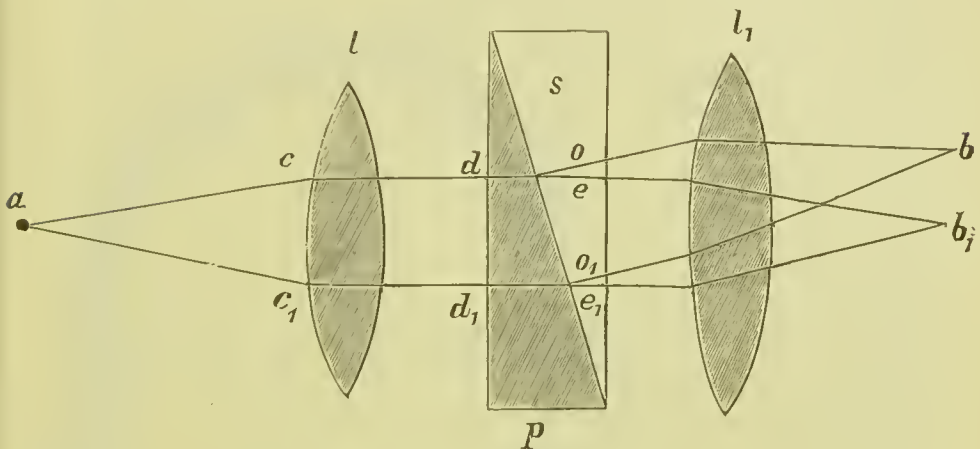
- Ophthalmometer von Javal (schematisch).
