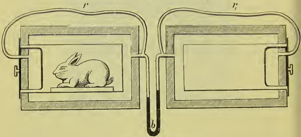
Luftcalorimeter mit Differentialmanometer.
