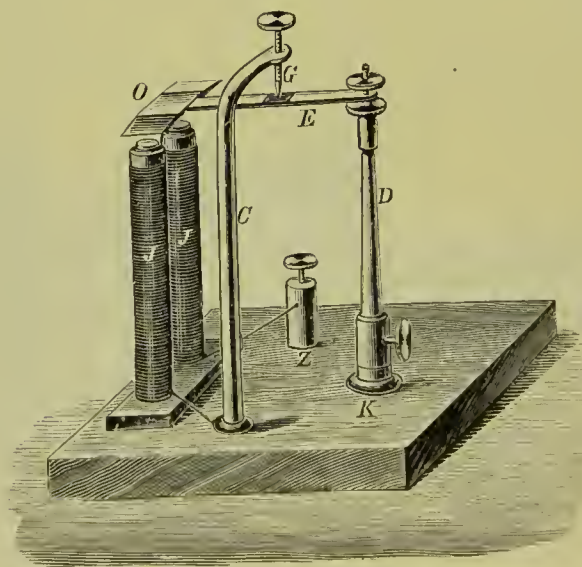
Wagner'scher Hammer.
