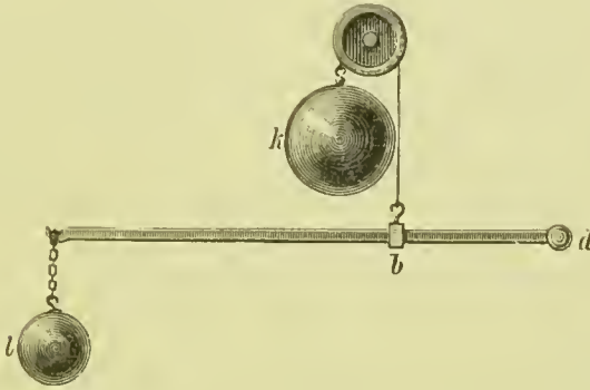
Einarmiger Hebel. Der Hebelarm der Kraft k , bd , ist kürzer als der der Last l , ld .
