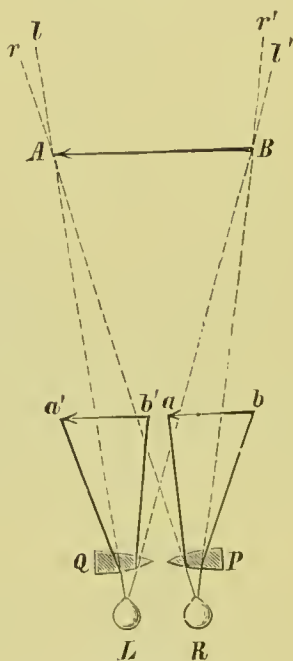
Prismenstereoskop.
