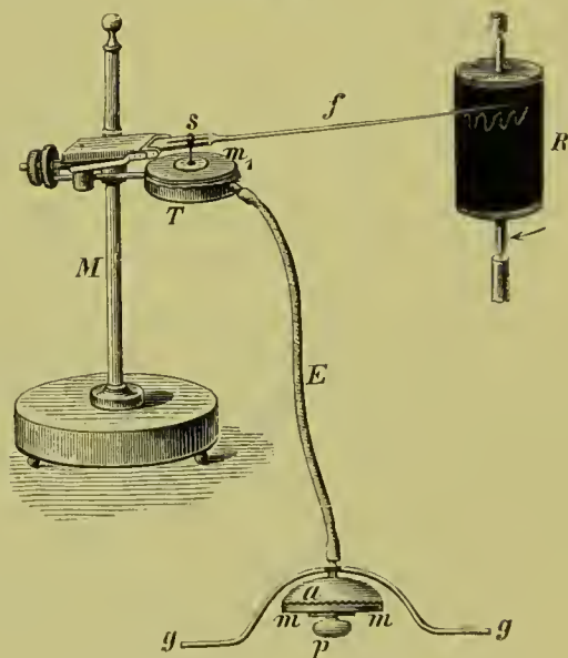
Graphische Darstellung der Herzbewegung.
