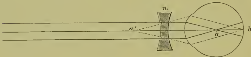
Correction der Kurzsichtigkeit.
