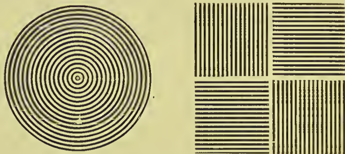
Zur Beobachtung des Astigmatismus des Menschenauges.
