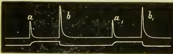
Ungleiche Wirkung des Schliessungs- ( a , a ,) und Oeffnungsinductionsschlages ( b , b ,) auf den Muskel. Oben Zuckungscurven, unten Reizscheiben im primären Kreis.
