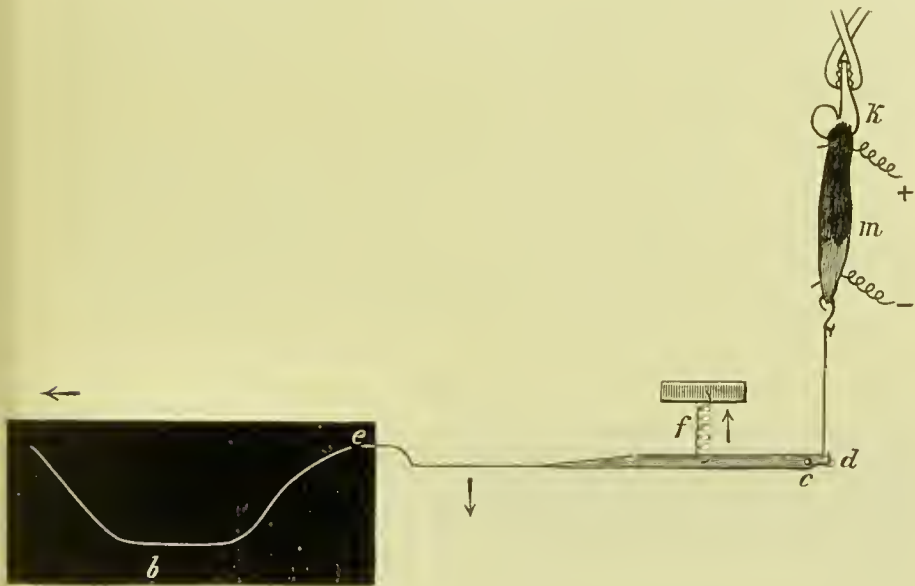
Anordnungen für isometrische Zuckungen.
