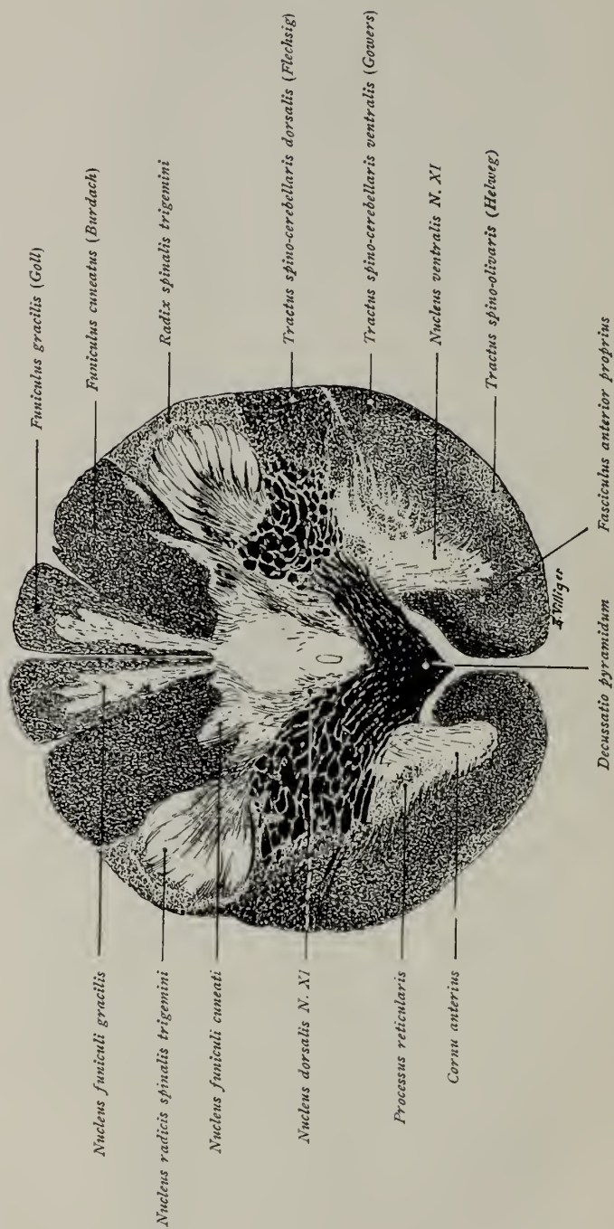
Fig. 205.
