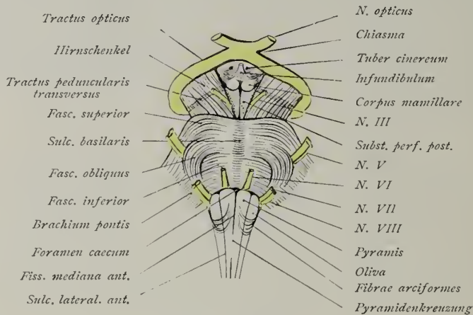
Fig. 75. Hirnbasis.
