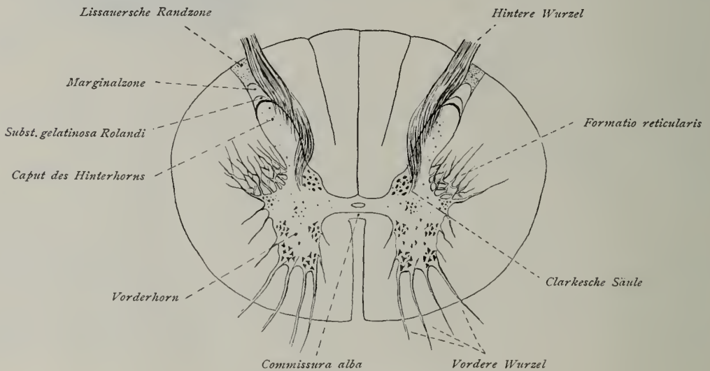
Fig. 94. Rückenmarksquerschnitt.
