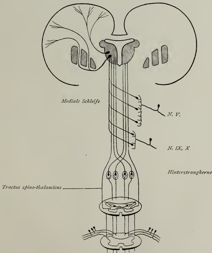
Fig. 168. Sensible Bahn.
