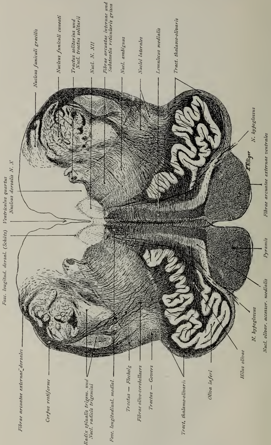
Fig. 210.
