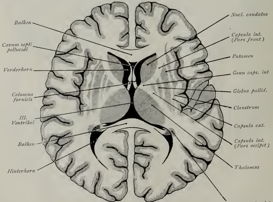
Fig. 53. Horizontalschnitt.
