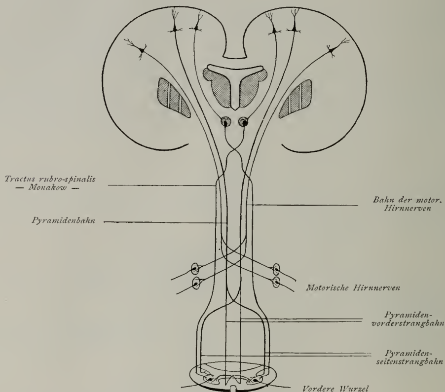
Fig. 171. Motorische Bahn.
