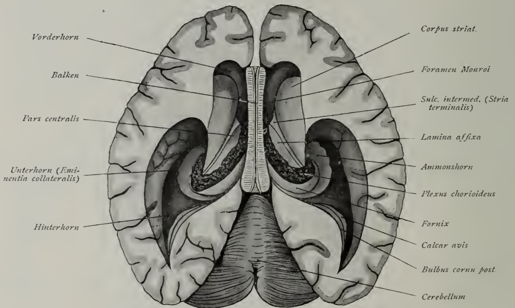
Fig. 42. Seitenventrikel.
