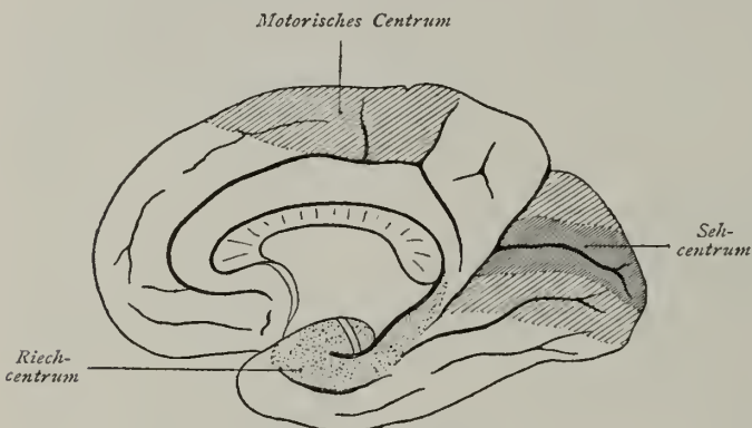
Fig. 118. Hirnlokalisation.
