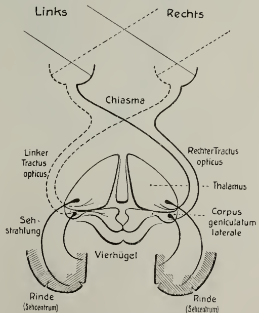
Fig. 154. Sehbahn.
