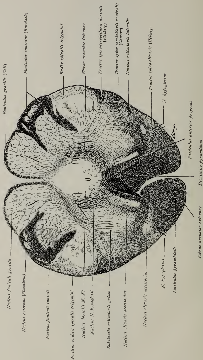
Fig. 207.
