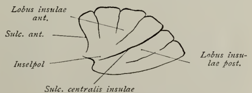
Fig. 21. Insula, schematisch.
