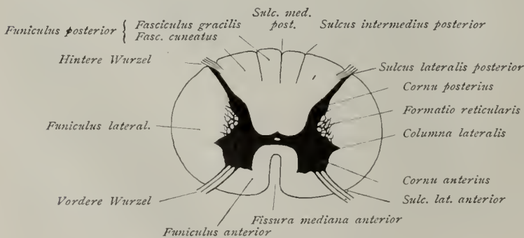
Fig. 92. Rückenmarksquerschnitt.
