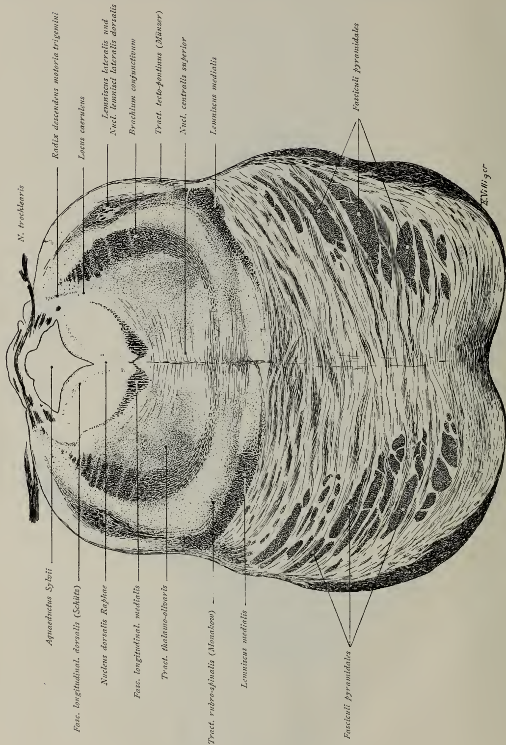
Fig. 220.
