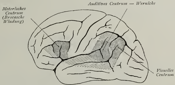
Fig. 119. Hirnlokalisation. Sprachcentrum.
