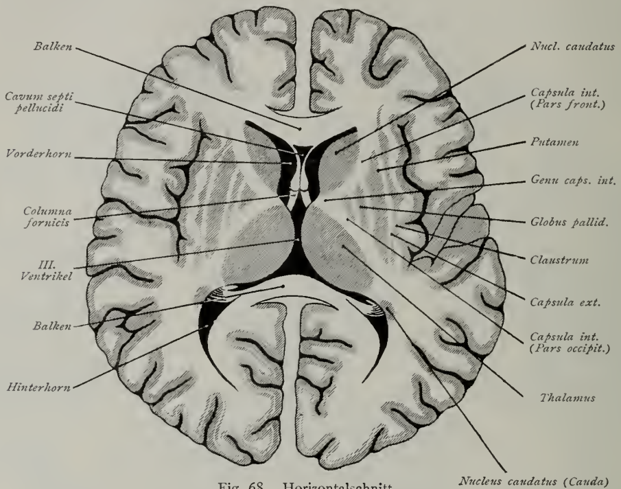
Fig. 68. Horizontalschnitt.
