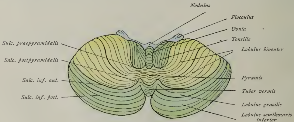
Fig. 77. Untere Kleinhirnfläche.
