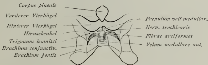
Fig. 74. Isthmus rhombencephali.
