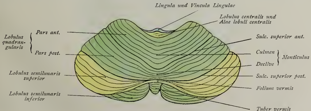
Fig. 76. Obere Kleinhirnfläche.
