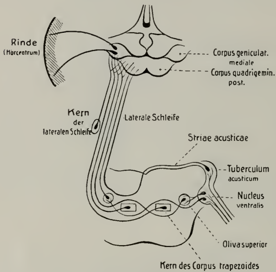
Fig. 161. Hörbahn.
