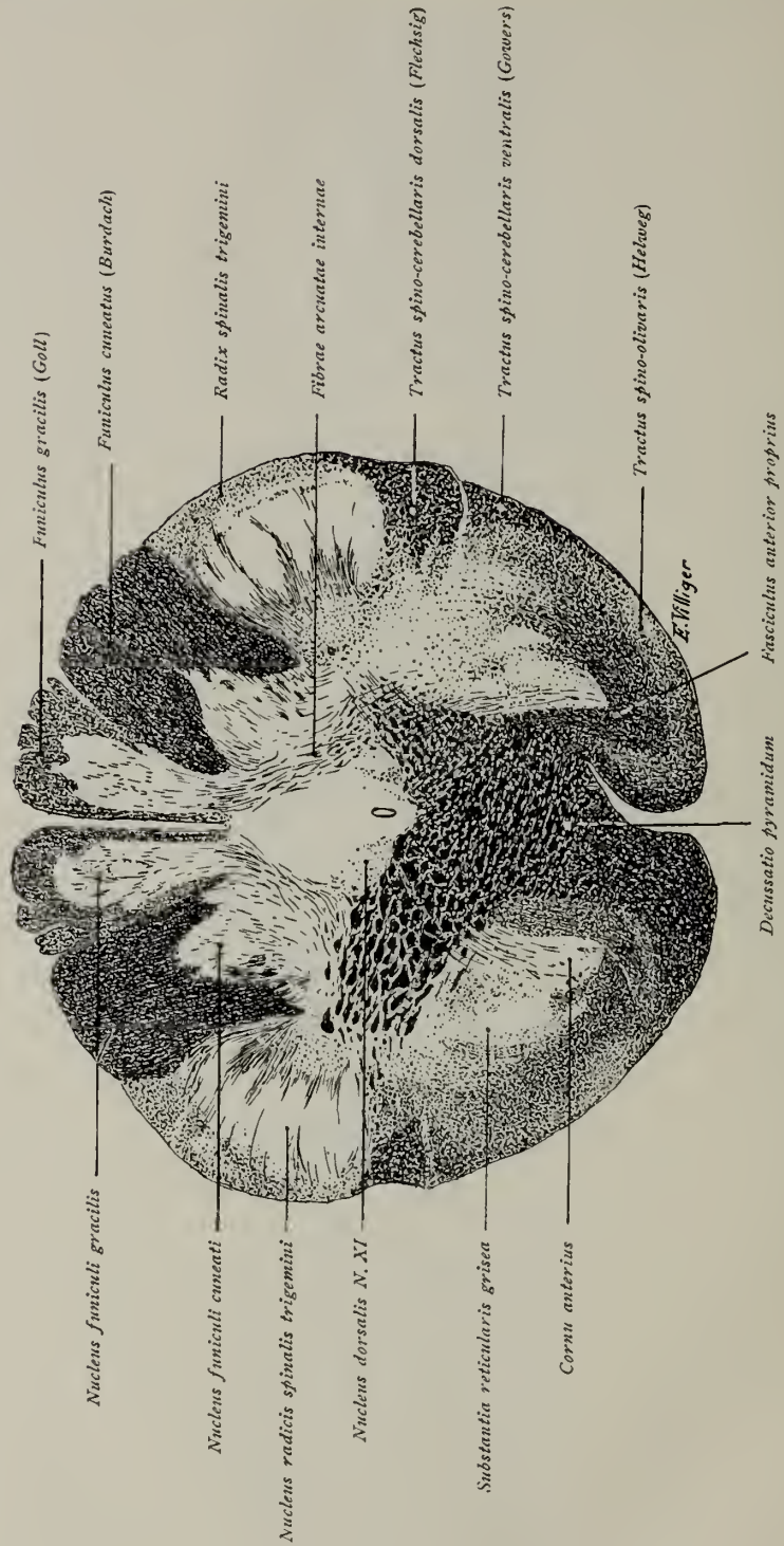
Fig. 206.
