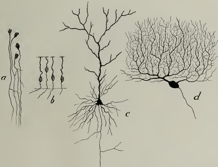
Fig. 108. Nervenzellen.
