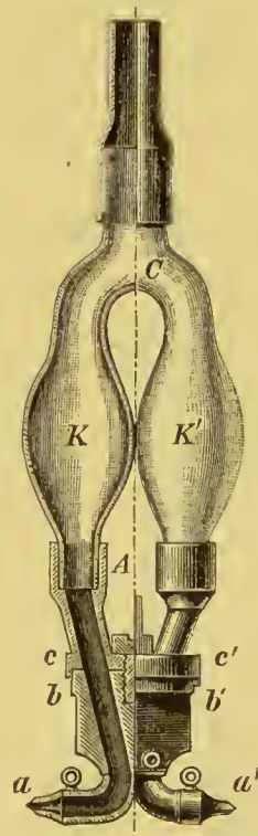
Ludwig's Stromuhr.
