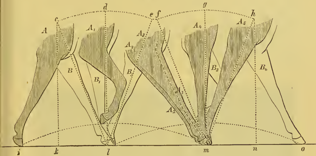
Ausschreitendes und stützendes Vorderbein des Pferdes.
