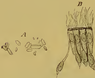
A Otolithen vom Pferd. B Epithel der Crista acustica mit Hörhaaren vom Kaninchen.
