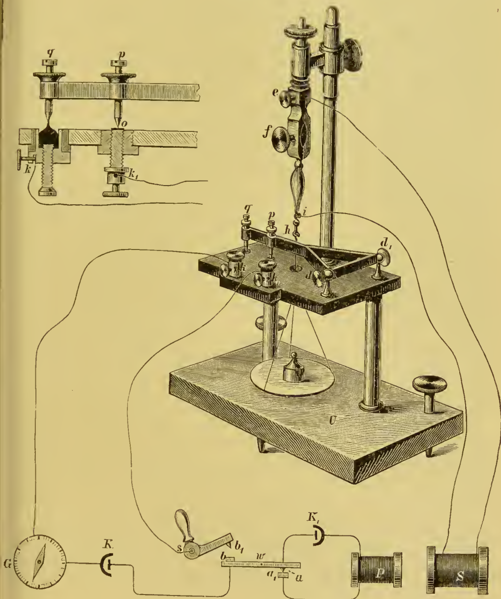
Zeitmessung der Muskelzuckung nach v. Helmholtz. U der Froschunterbrecher von du Bois-Reymond.
