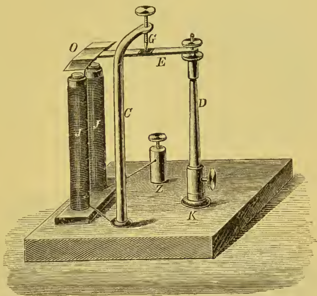
Wagner'scher Hammer.
