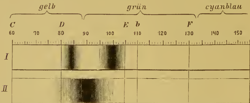
Absorptionsbänder des Oxyhaemoglobin (I) und des reducirten Haemoglobin (II).
