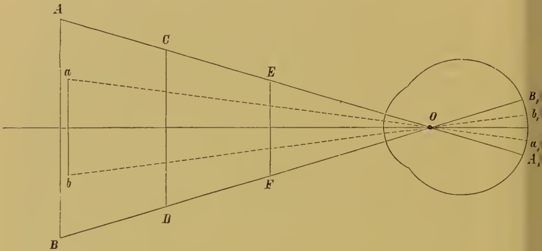
Schätzung der Grösse und Entfernung aus dem Sehwinkel.
