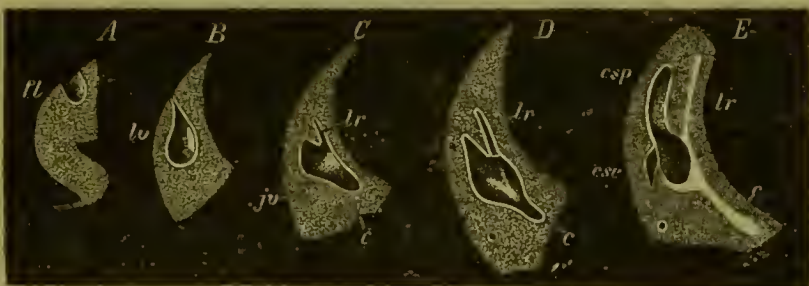
Fig. 268. Entwicklung des Labyrinthes beim Hühnchen. Senkrechte Querschnitte der Schädelanlage. fl Labyrinthgrube. lv Labyrinthbläschen. c Anlage der Schnecke. lr Recessus labyrinthi. csp Hinterer Bogengang. cse Aeusserer Bogengang. vj Jugularvene. (Nach REISSNER.)
