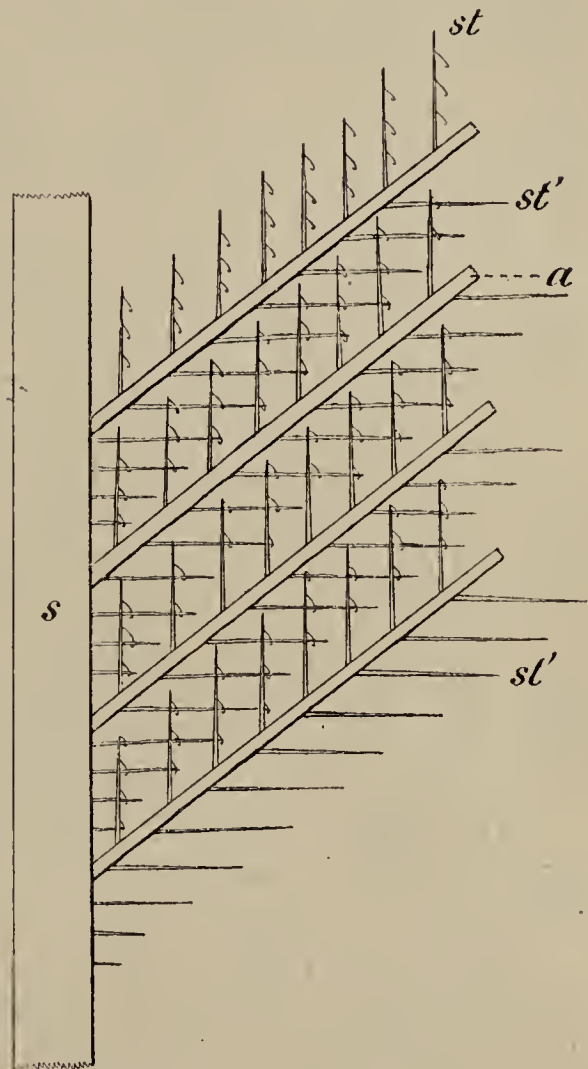
Fig. 316. Stückchen einer Feder, Schema. s Schaft, a Ast, st Strahlen einer vorderen Reihe mit Häkchen, st' Strahlen der hinteren Reihen; erstere decken über letztere hin und greifen mit den Häkchen um ihren Rand. — Orig.
