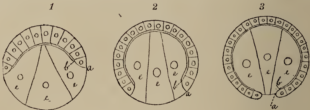
Fig. 26. Schematische Figuren zum Verständniss der epibolischen Gastrula (vergl. den Text). 1 jüngstes, 3 ältestes Stadium. e Entodermzellen. Die Buchstaben a und b bezeichnen in allen drei Figuren dieselben Stellen. — Orig.
