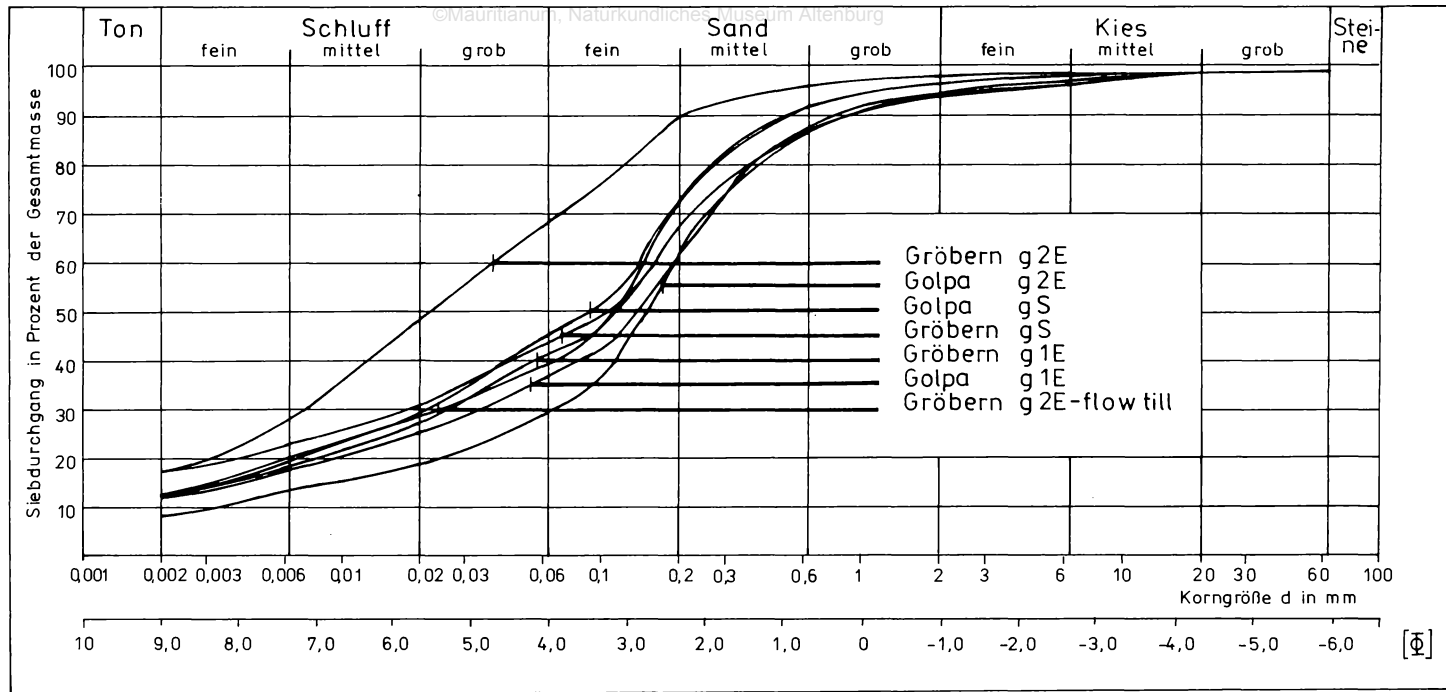
Abb. 7. Mittlere Kornsummenkurven
