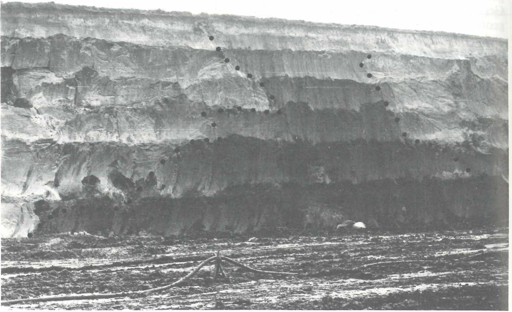
Abb. 9. Gekappter und von Geschiebedecksand überlagerter Till-Diapir (g2E), elsterkataglaziale Schmelzwassersande in den Randsenken; Tagebau Gröbern, März 1988, Stoßhöhe ca. 15 m
