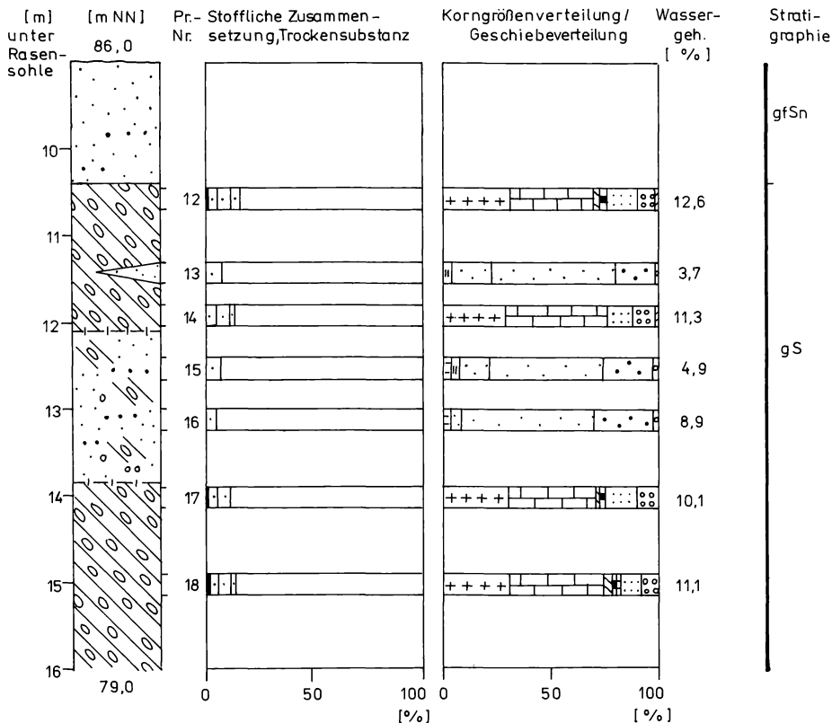
Abb. 5. Profil 2, Proben 2/12–18 – Gröbern
