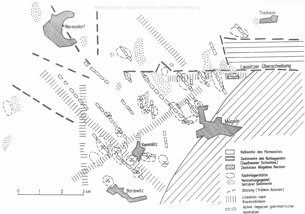
Abb. 4. Verbreitungsschema von Kaolinlagerstätten und Vorkommen von Tertiärsedimenten im nordwestsächsischen Kaoliningebiet; Kaolinverbreitung nach SCHWERTNER u. STÖRR 1983, PENTZEL 1989, ALEXOWSKY 1990 und WALTER 1990. Gravimetrische Angaben nach GRIMMER; Kosmoslineationen nach KRENTZ; tektonische Elemente nach verschiedenen Autoren (zusammengestellt nach WALTER et al., in Vorber.)
