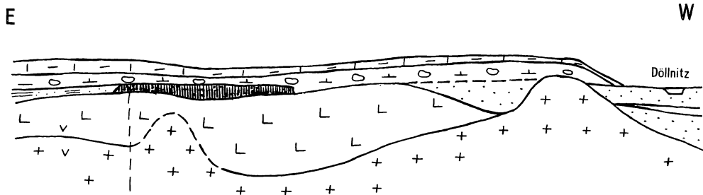
Abb. 1. Geologischer Schnitt durch die Kaolinlagerstätte Gröppendorf auf ca. 400 m Länge; Zeichen-erklärung siehe Abb. 3; nach STÖRR u. SCHWERTNER 1974, SCHWERTNER u. STÖRR 1983
