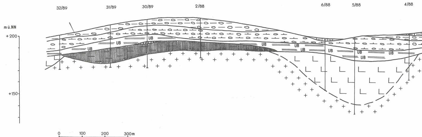
Abb. 2. Geologischer Schnitt durch die Kaolinlagerstätte Seelitz und des westlich angrenzenden Gebietes im Norden von Mügeln; Zeichenerklärung siehe Abb. 3; nach WALTER 1990
