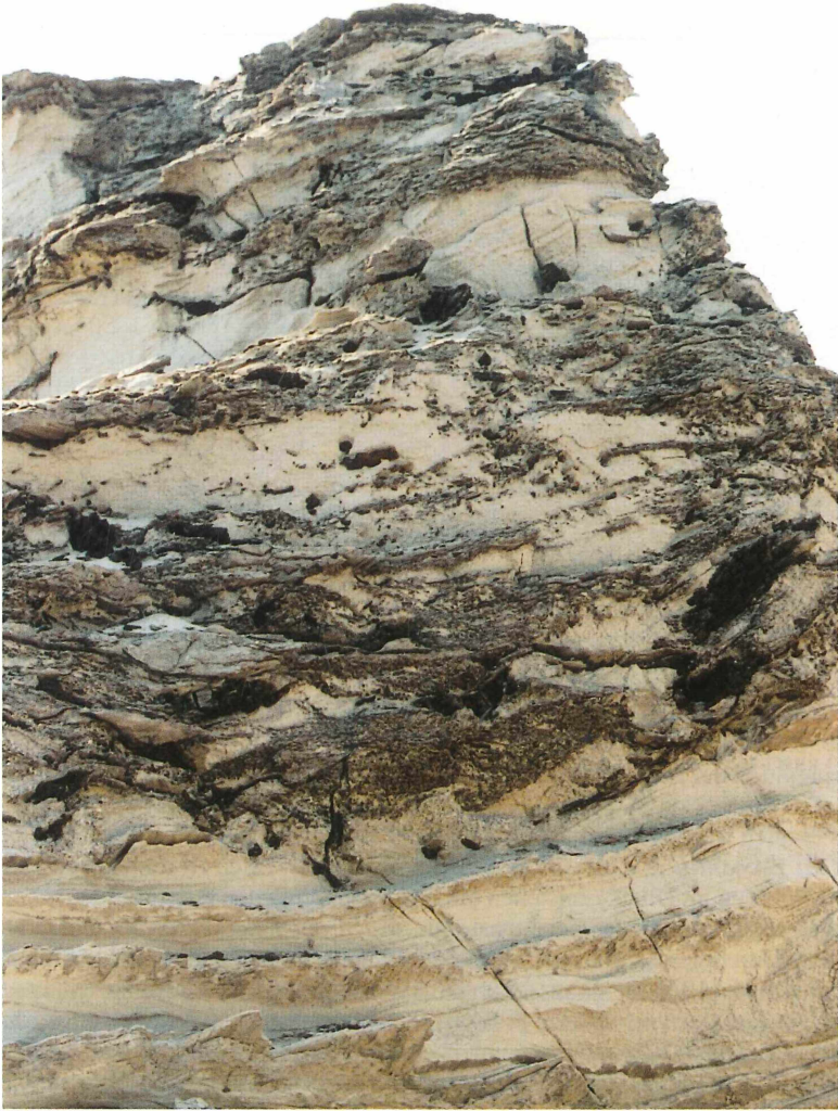
Foto 5. Charakteristischer Ausschnitt einer turbulenten Abfolge in den Hainer Sanden, die im ästuarinen Bereich abgelagert wurde (Schicht 3)
