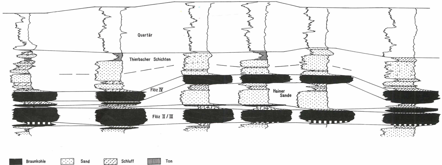
Abb. 2a. Bohrlochgeophysikalisches Korrelationsprofil (Bereich der dokumentierten Hainer Sande im Tagebau Witznitz) zur Verdeutlichung der lateralen Mächtigkeitsabnahme und der lithologischen Veränderungen (Bezugsniveau: Oberfläche des Flöz II/III-Komplexes, Länge unmaßstäblich)
