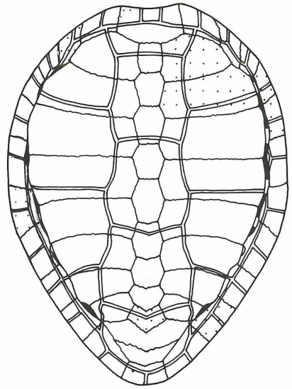
Abb. 4. Tropidemys langii RÜTIMEYER 1873, dorsale Carapaxansicht nach verschiedenen Autoren, umgezeichnet. Vorhandene Plattentypen punktiert
