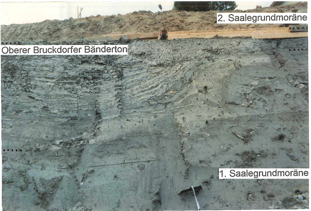
Bild 8. Glazigen gestörter Oberer Bruckdorfer (Vorstoß-)Bänderton (Typ „Eutritzscher Bänderton“; g_{1,S} ) in lokaler muldenartiger Eintiefung zwischen Erster ( g_{1,S} ) und Zweiter ( g_{2,S} ) Saalegrundmoräne in Leipzig-Eutritzsches (temporärer Aufschluß beim Brückenbau Essener Straße/Dübener Landstraße).
