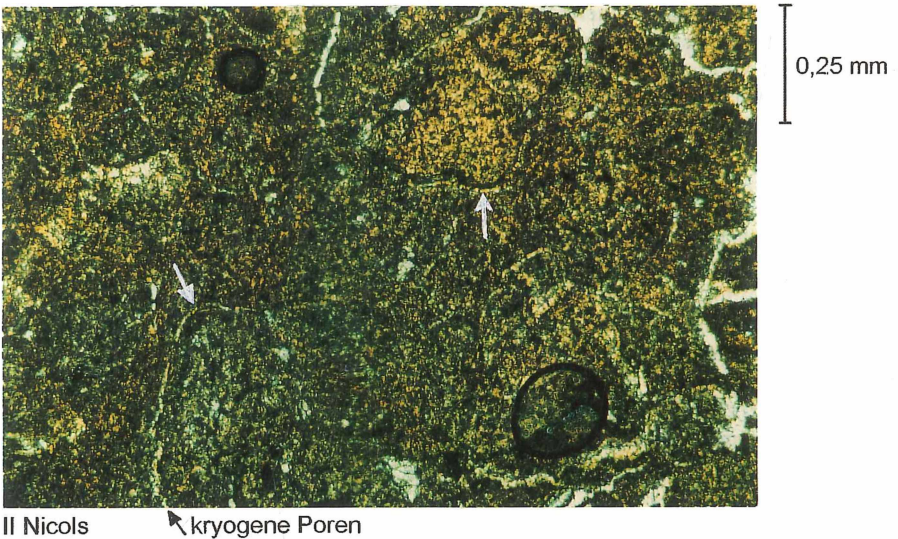
Bild 4. Detailaufnahme der Schlufflagen des Unteren Bruckdorfer (Rückzugs-)Bändertons. Tagebau Delitzsch-Südwest. Feine linsenartige kryogene Poren mit teilweise fiederartiger Anordnung, dabei die brekziöse Struktur nachzeichnend, kennzeichnen die Mikrotextur der Schlufflagen. Kreise = Luftblasen präparativer Natur.
