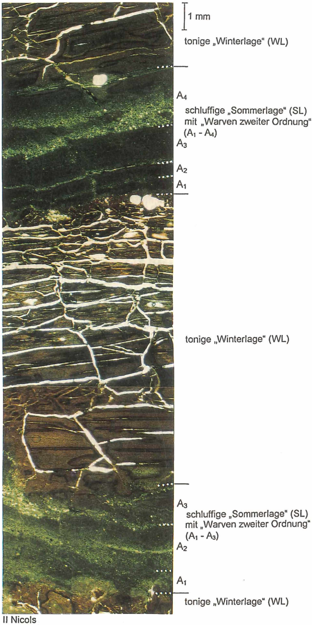
Bild 9. Lagenaufbau des Oberen Bruckdorfer (Vorstoß-)Bänderton im Dünnschliff. Temporärer Aufschluß Landsberger Straße 23. Die tonigen Winterlagen sind durch eine kryogene netzartige Mikrotexur (Lattice-like or reticulate cryogenic microstructure) gekennzeichnet.
