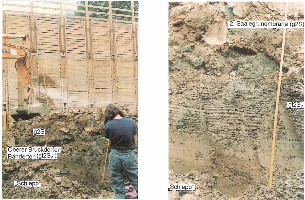
Bild 6. Auftreten des Oberen Bruckdorfer (Vorstoß-)Bändertons in Leipzig-Gohlis (temporärer Aufschluß Landsberger Straße 23). Deutlich erhöhte Lagenmächtigkeiten („Riesenwarven“) kennzeichnen den Liegendübergang des unter der zweiten Saalegrundmoräne lagernden Oberen Bruckdorfer (Vorstoß-)Bändertons. Foto JUNGE 1993.
