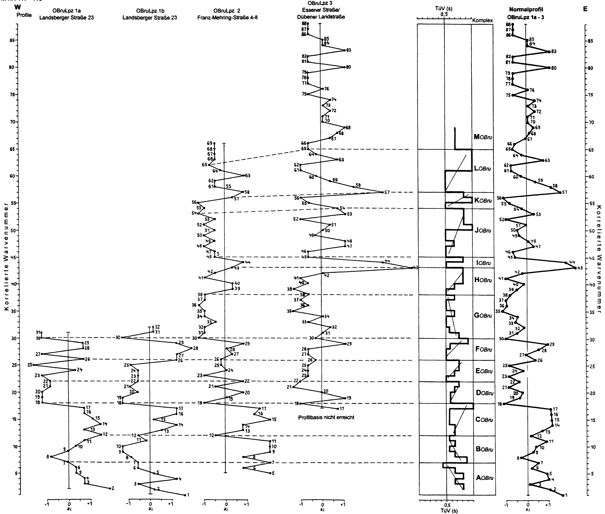
Abb. 2. Konnektierung der tonigen „Winterlagen“ des Oberen Bruckdorfer (Vorstoß-)Bändertons im nördlichen Stadtgebiet von Leipzig. Die Lagenkonnektierung erfolgt auf der Methode nach KÜHL (1991). Die konnektierte West-Ost-Profilstrecke im Stadtgebiet von Leipzig umfaßt ca. 3 Kilometer. Dargestellt sind von links nach rechts: (a.) die lokalsystematischen Mächtigkeitsänderungen a_i der „Winterlagen“ innerhalb der 4 untersuchten Einzelprofile im Stadtgebiet; (b.) Profilverlauf des Trendübereinstimmungskoeffizienten (TüV(s)) als Gradmesser für die Höhe der Übereinstimmung der konnektierten Lagen; (c.) nach dem Profilverlauf des TüV(s) (Trendwechsel) unterschiedene Komplexe; (d.) Normalprofil der lokalsystematischen Mächtigkeitsänderungen a_i der „Winterlagen“ des Oberen Bruckdorfer (Vorstoß-) Bändertons im Stadtgebiet von Leipzig.
