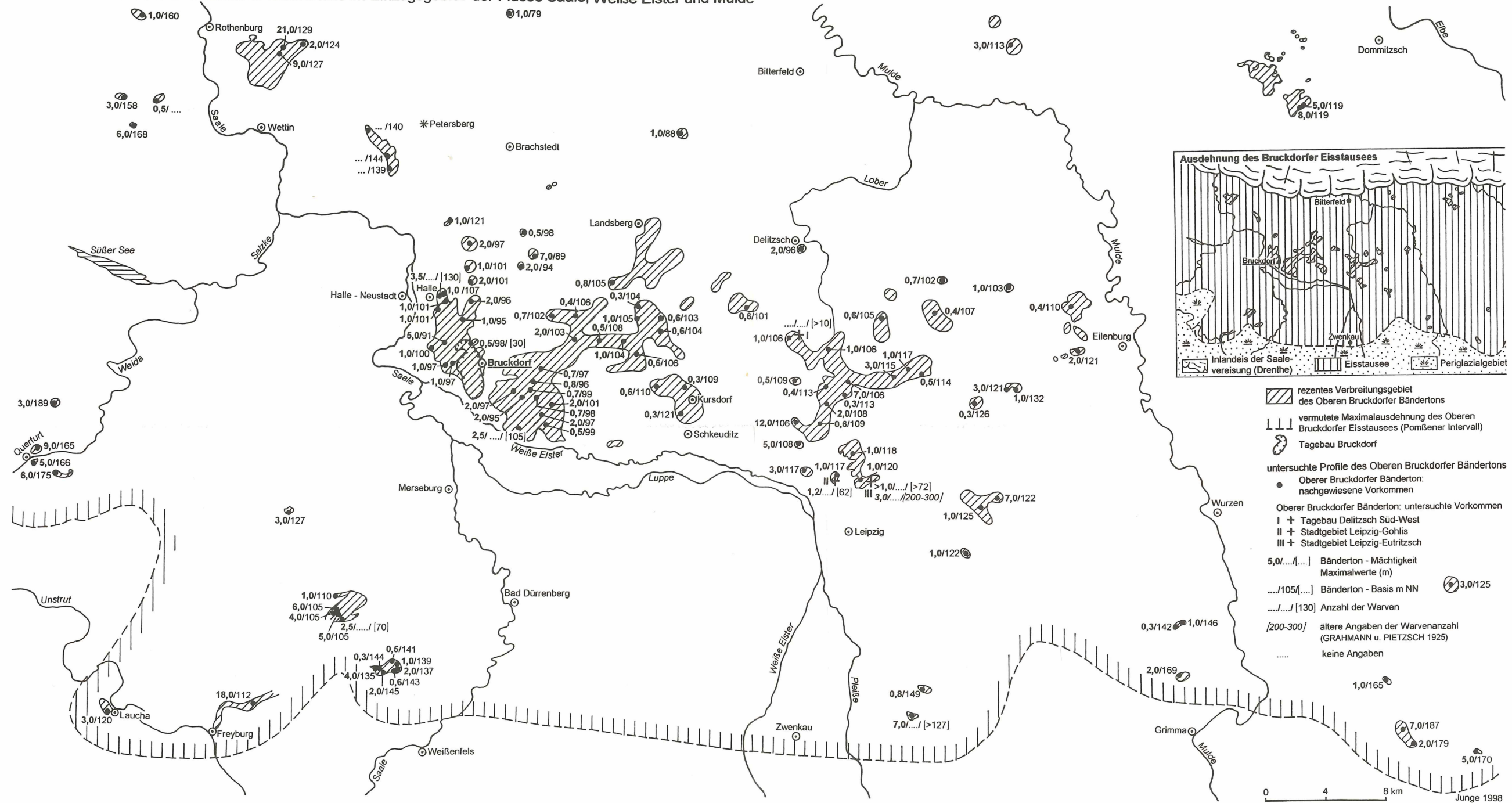
Abb. 1. Verbreitung und Merkmale (Basishöhe, Mächtigkeit, Warvenanzahl) des Oberen Bruckdorfer (Vorstoß-)Bändertons in Mitteldeutschland. Die Zusammenstellung der mit Angaben zur Basishöhe (in Meter über Normalniveau, mNN), zur Mächtigkeit (in Meter) und zur Warvenanzahl versehenen Vorkommen des Oberen Bruckdorfer (Vorstoß-)Bändertons erfolgte unter Verwendung der Lithofazieskarten Quartär 1 : 50 000 (Horizontkarten g S1 -S 2v der Blätter Halle-Nord (2464), Bitterfeld (2465), Eilenburg (2466), Halle Süd (2564), Leipzig (2565) und Wurzen (2566), unter Verwendung von Literaturangaben und eigenen Beobachtungen.
