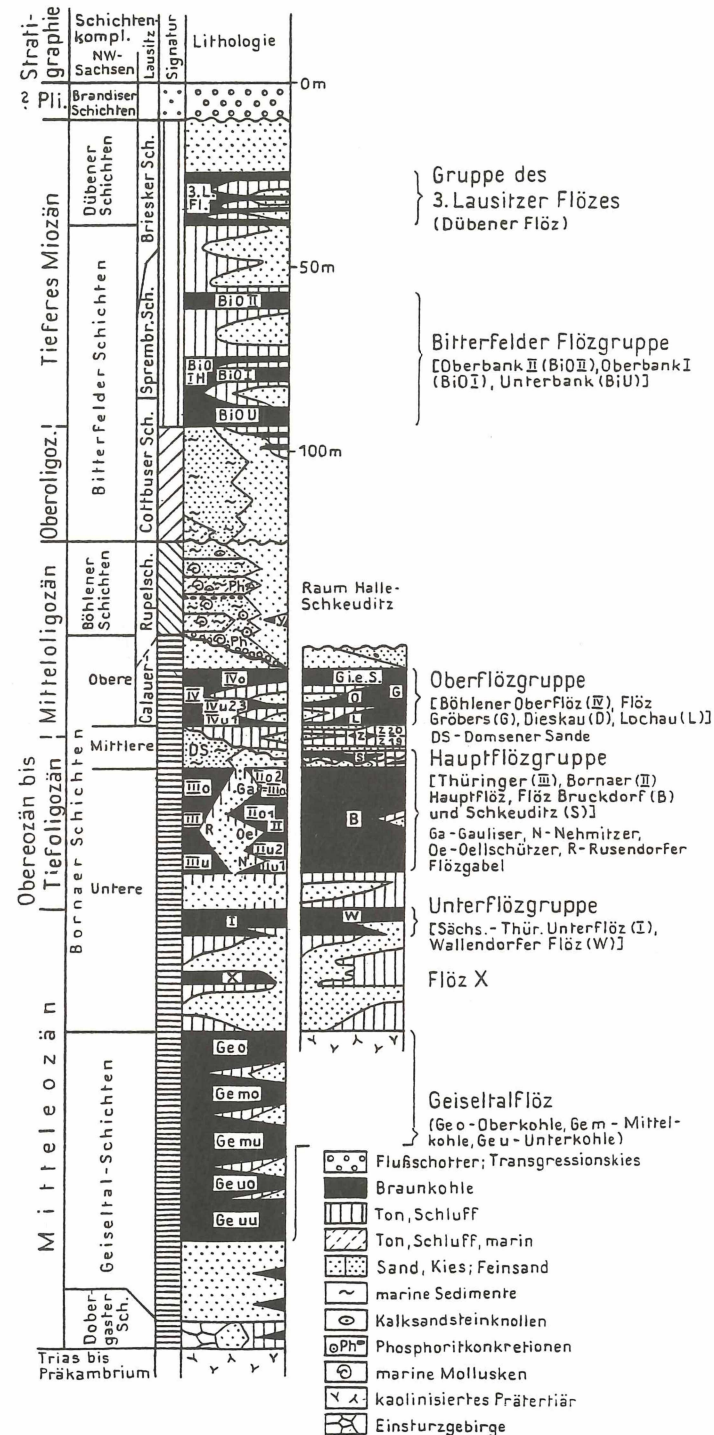
Abb. 4b. Das Tertiär Nordwestsachsens und des angrenzenden Gebietes in vereinfachter Darstellung in den neunziger Jahren dieses Jahrhunderts. Der größte Fortschritt wurde zwischen 1960 und 1980 erreicht.
