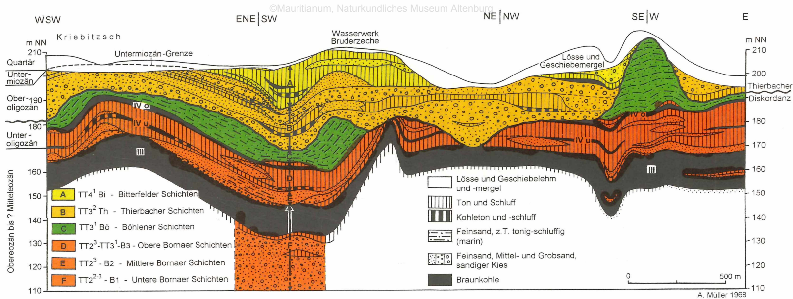
Abb. 2. Referenzschnitt durch das Unteroligozän (Bitterfelder Schichten), das Oberoligozän (Thierbacher Schichten) und das ältere Tertiär im südlichen Weißelsterbecken bei Kriebitzsch (Entwurf Ansgar Müller, 1968; leicht verändert)
