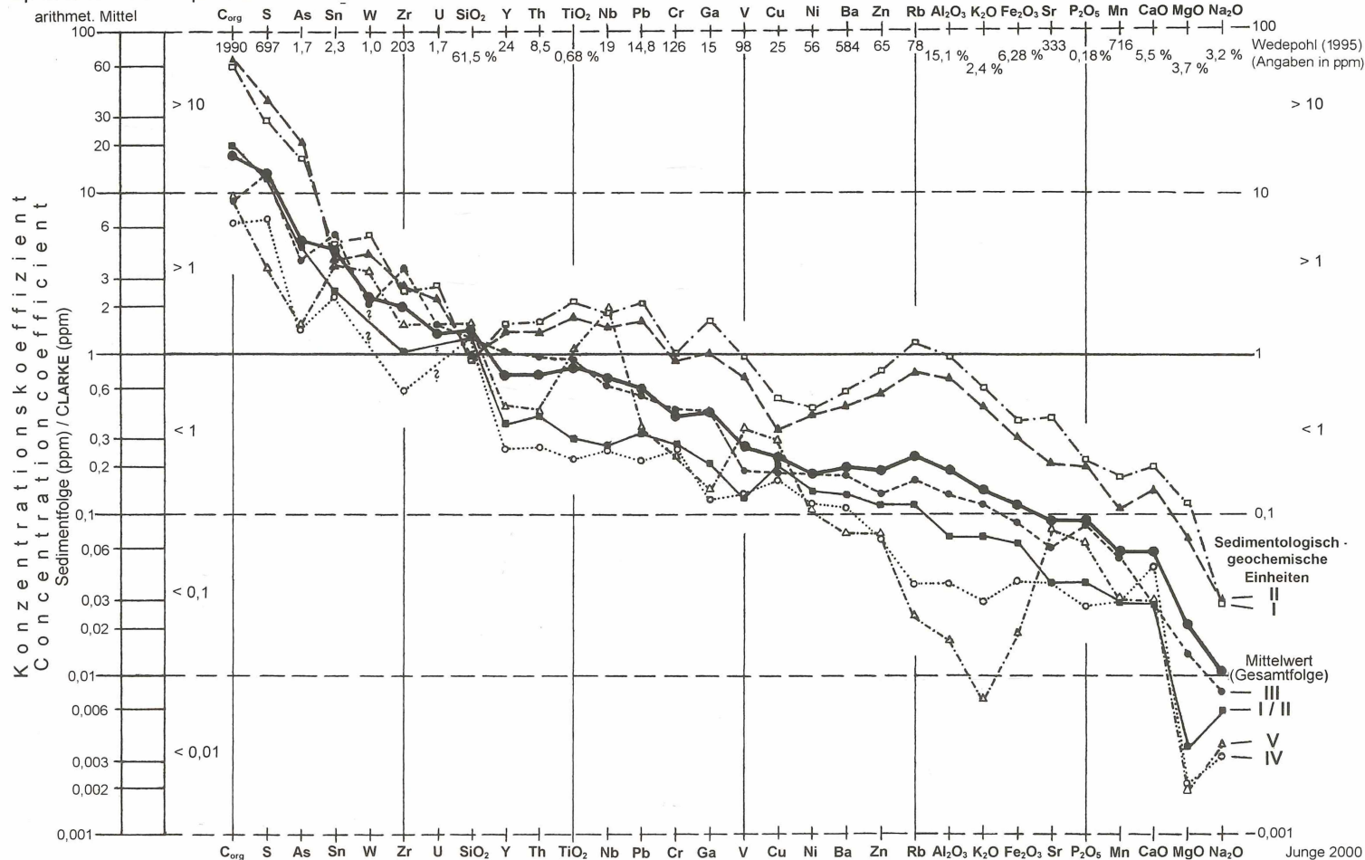
Abb. 7. Mittlere An- und Abreicherungsfaktoren der untersuchten Haupt- und Spurenelemente gegenüber dem Clarke-Wert der kontinentalen Kruste nach Wedepohl (1995) in der obereozän-unteroligozänen Sedimentfolge und ihrer sedimentologisch-geochemischen Einheiten.
