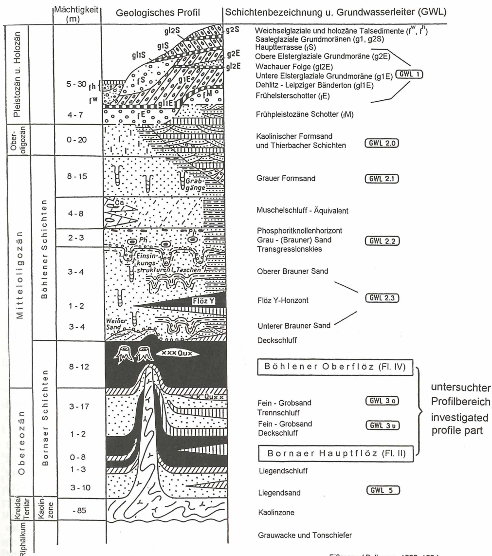
Abb. 1. Typusprofil der känozoischen Schichtenfolge im Tagebau Espenhain (nach EISSMANN/BELLMANN 1990, 1994).
