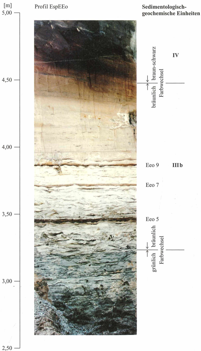
Bild 1. Ausschnitt aus der obereozän-unteroligozänen Sedimentfolge des Profils EspEEo mit den sedimentologisch-geochemischen Einheiten IIIb und IV
