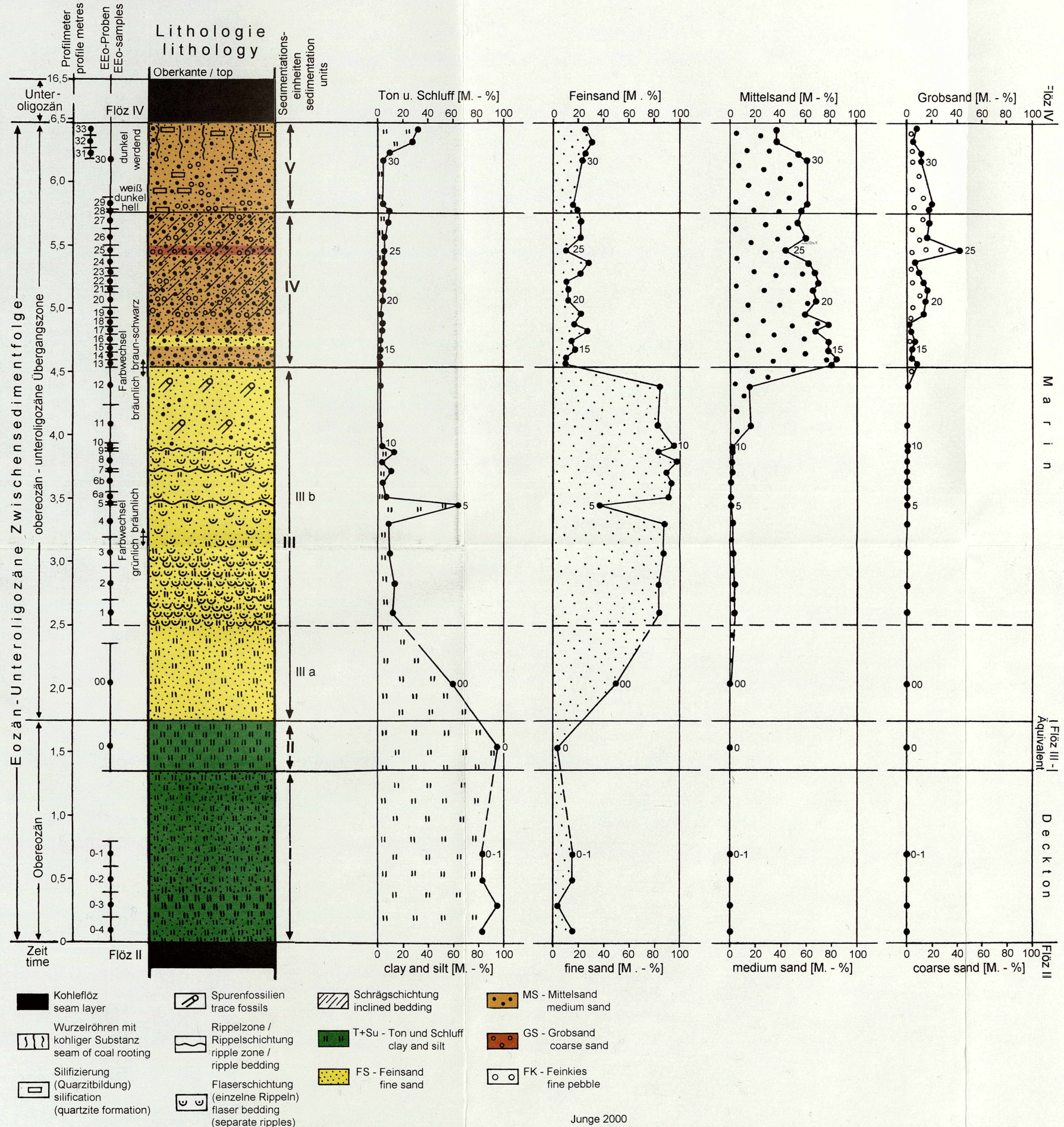
Abb. 3. Lithologischer Aufbau, Korngrößenzusammensetzung und sedimentologisch-geochemische Einheiten des obereozän-unteroligozänen Zwischenmittels im Profil EspEEO.
