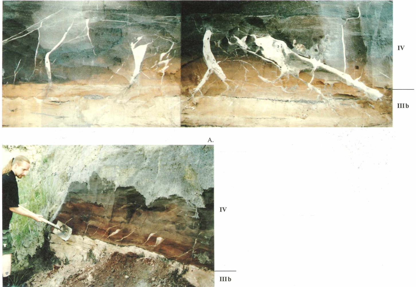
Bild 2. Setzungsbedingtes Kluftsystem mit hellen Feinsanden im Übergangsbereich der sedimentologisch-geochemischen Einheiten IIIb und IV des Profils EspEEo. A. Übersichtsaufnahme; B. Detailausschnitt.
