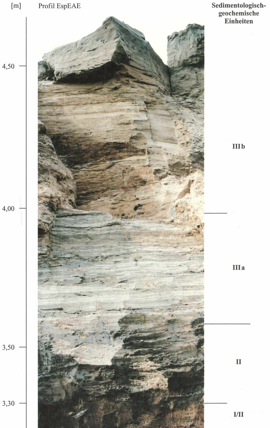
Bild 4. Ausschnitt aus dem oberen Teil der obereozän-unteroligozänen Sedimentfolge des Profils EspEAE mit den sedimentologisch-geochemischen Einheiten I/II, II und III.
