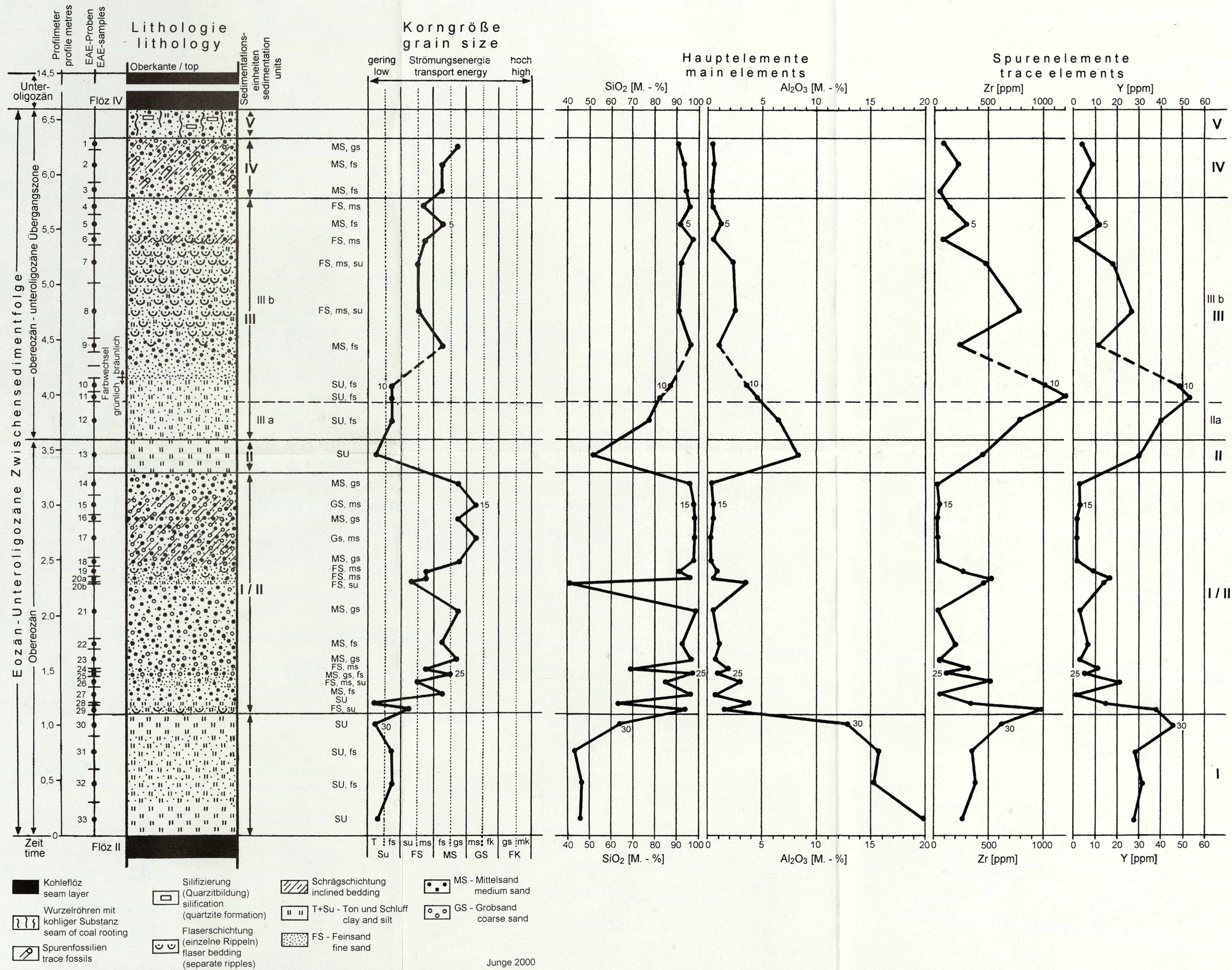
Abb. 6. Verteilung der Hauptelemente SiO 2 , Al 2 O 3 und der Spurenelemente Zr, Y in der obereozän-unteroligozänen Sedimentfolge des Profils EspEAE. Erläuterungen siehe Abb. 4.
