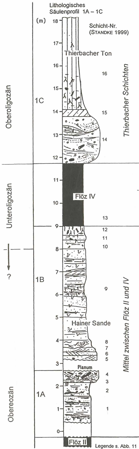
Abb. 10. Geologisch dokumentiertes Profil des „Zwischenmittels“ zwischen Flöz II und IV (Hainer Sande, Profil 1A, 1B) und Thierbacher Schichten über Flöz IV (Profil 1C) im NW-Bereich des Tagebaus Bockwitz
