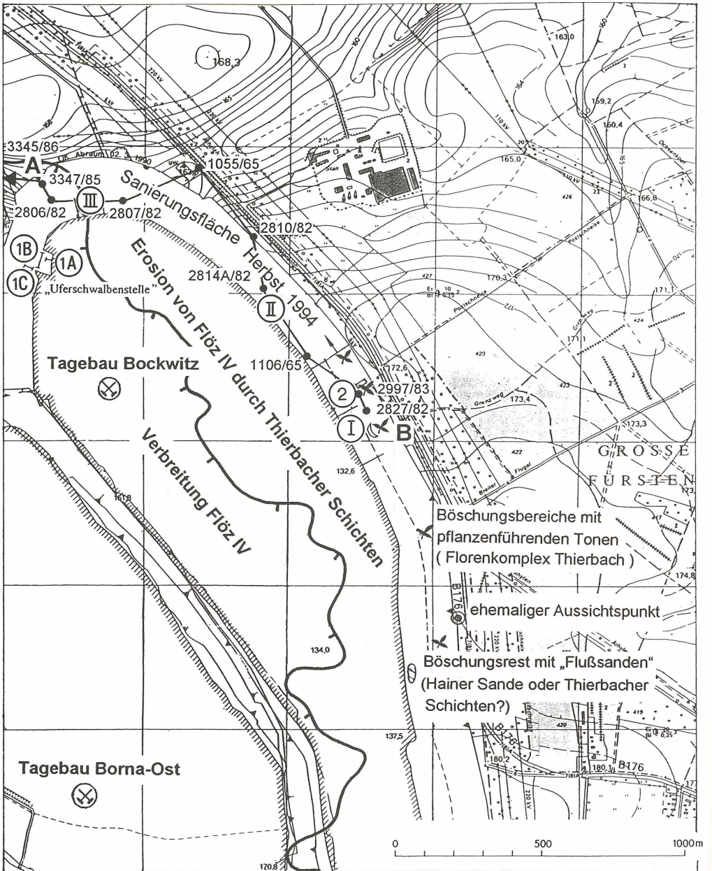
Abb. 6. Lageplan des Tagebaus Bockwitz mit dokumentierten Profilabschnitten (Profile 1A–C, 2: STANDKE 1994; Profile I, II, III: PÖPPELREITER 1992) und Erosionsgrenze von Flöz IV durch Thierbacher Schichten (nach FEHR u. a. 1984) und Schnittspur, vgl. Abb. 12
