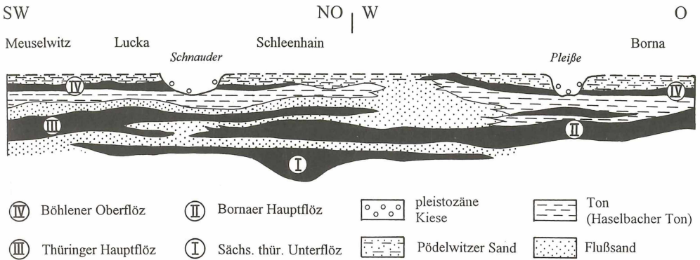
Abb. 5. Flözgliederung und Aufspaltung des Flözes II und III durch Flußsande (aus MEYER 1950, umgezeichnet)
