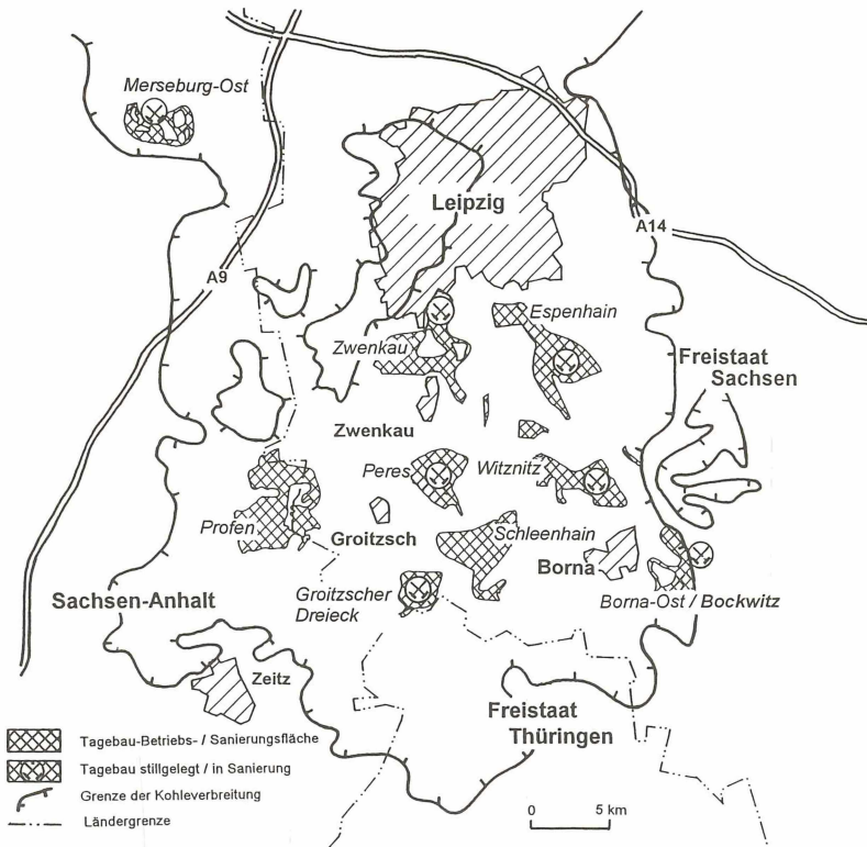
Abb. 1. Übersicht über die Braunkohlentagebaue im Südraum von Leipzig (nach LMVB, Stand 3/96)
