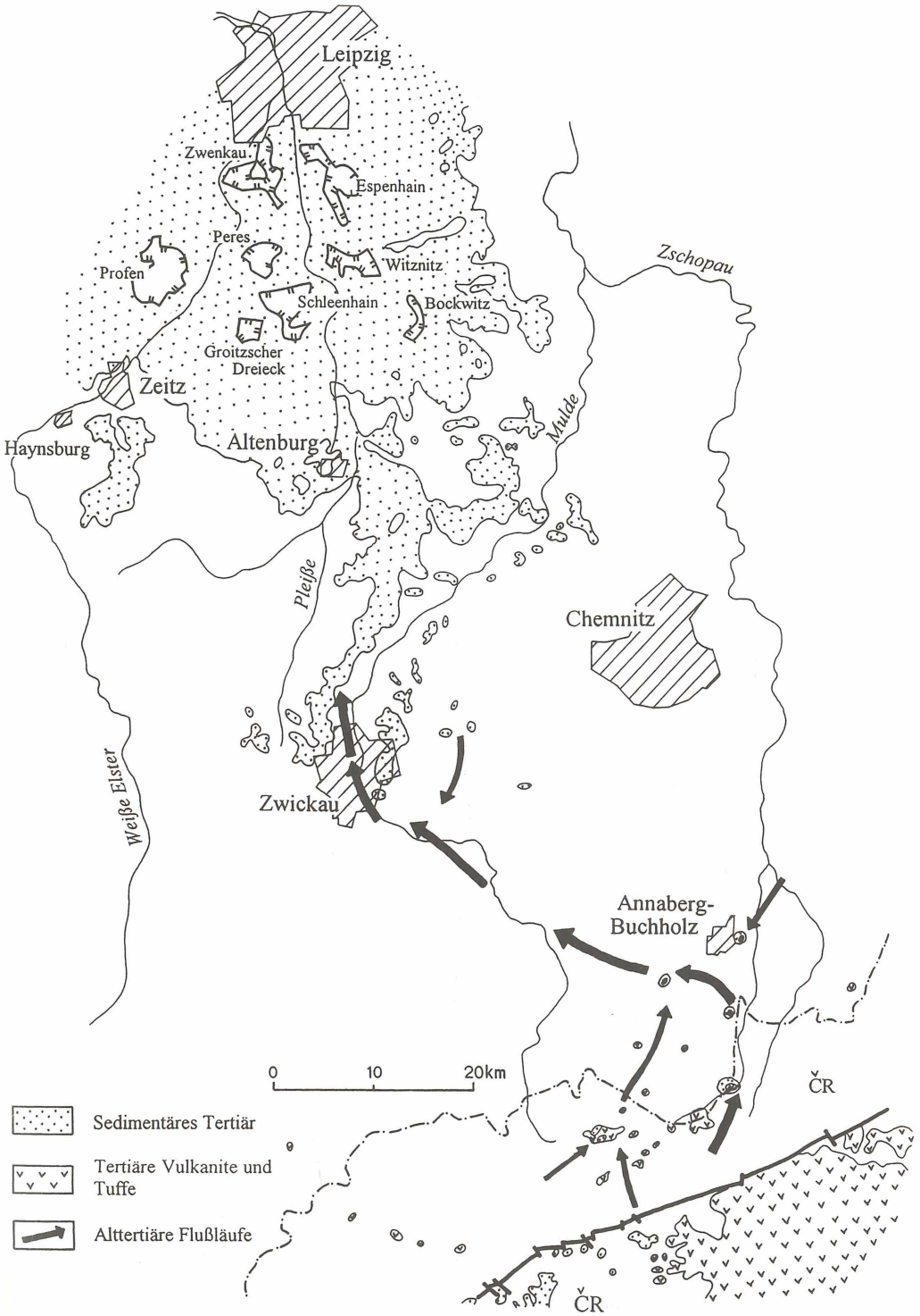
Abb. 2. Heutige Tertiärverbreitung im Südraum Leipzigs und alttertiäre Flußläufe (STANDKE & SUHR 1998)
