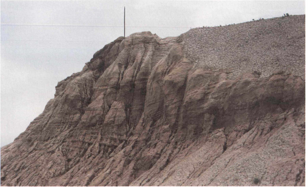
Foto 10. „Thierbacher Schichten“ oder Hainer Sande“? im Tagebau Bockwitz, Ostböschung (vgl. Abb. 6, Böschungrest mit „Fluvsanden“)
