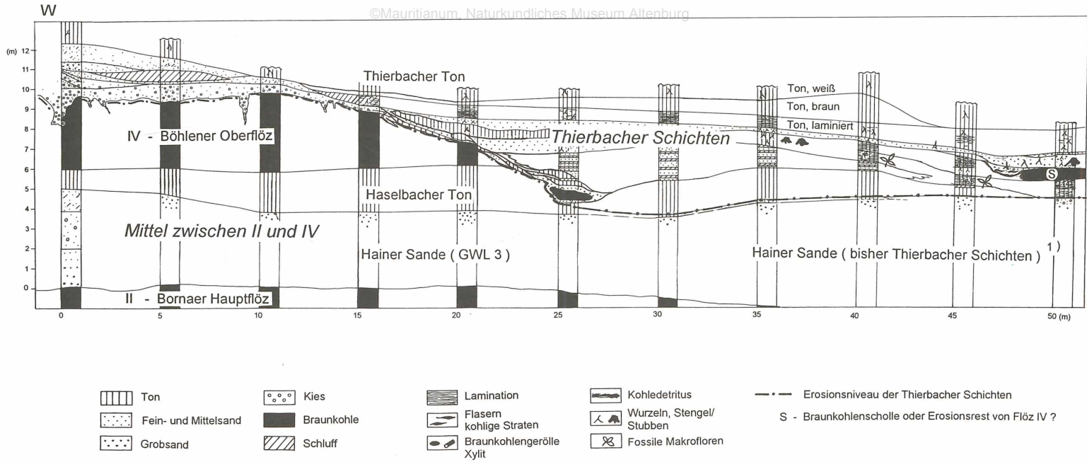
Abb. 11. Lithologische Profildokumentation im Erosionsbereich von Flöz IV durch Tierbacher Schichten (PÖPPELREITER 1992; umgezeichnet und verändert)
