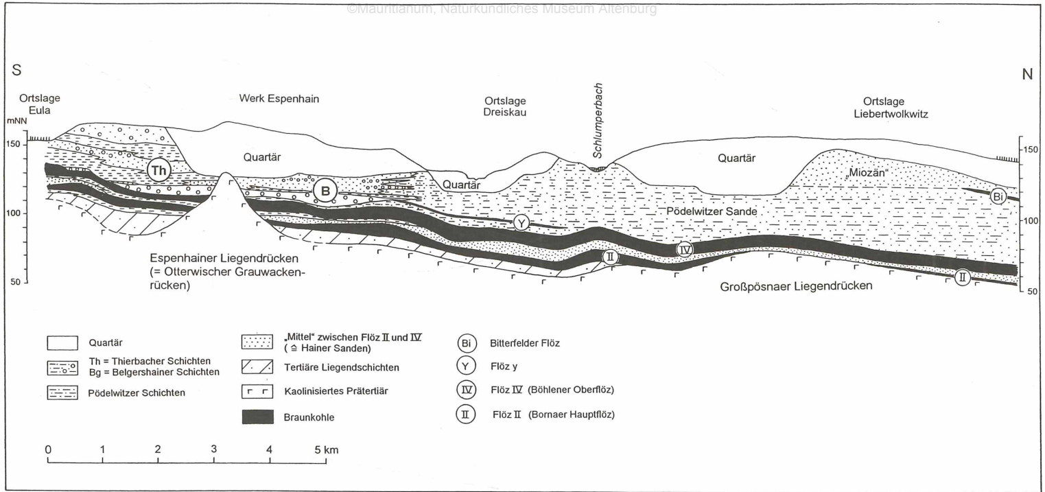
Abb. 8. Süd-Nord-Schnitt mit Verzahnungsbereich der Thierbacher/Belgershainer Schichten mit den „Pödelwitzer Sanden“ im Hangenden von Flöz IV im Raum Espenhain-Liebertwolkwitz (aus: MEYER 1952, umgezeichnet), Schnittspur s. Abb. 7
