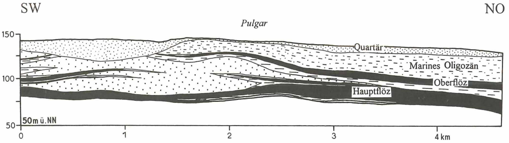
Abb. 4. Aufspaltung des Hauptflözes durch einen SE–NW durch das Braunkohlenmoor verlaufenden Fluß (aus PIETZSCH 1962, umgezeichnet)
