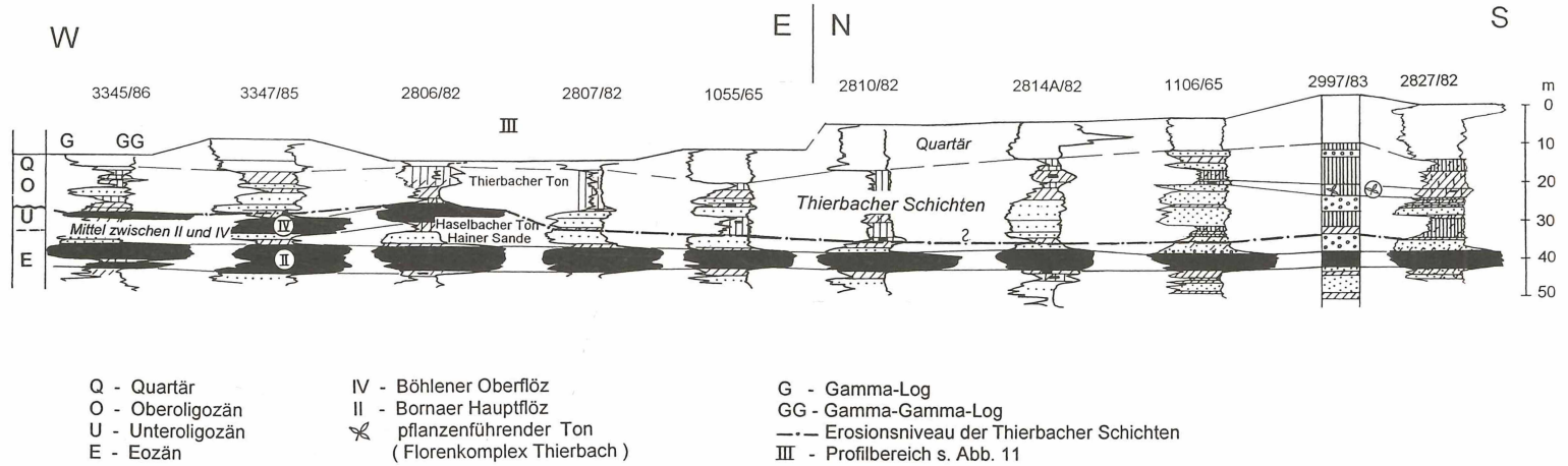
Abb. 12. Bohrlochgeophysikalisch-lithologisches Korrelationsprofil im Bereich der Thierbacher Schichten an der Nord- und Ostböschung des Tagebaus Bockwitz (Bezugsniveau: Flöz II)
