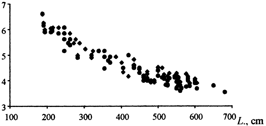
Abb. 3. Altersbedingte Veränderung des Verhältnisses L. cap./L. bei Vipera nikolskii aus dem Gebiet Saratow: \blacklozenge – Männchen, \bullet – Weibchen
