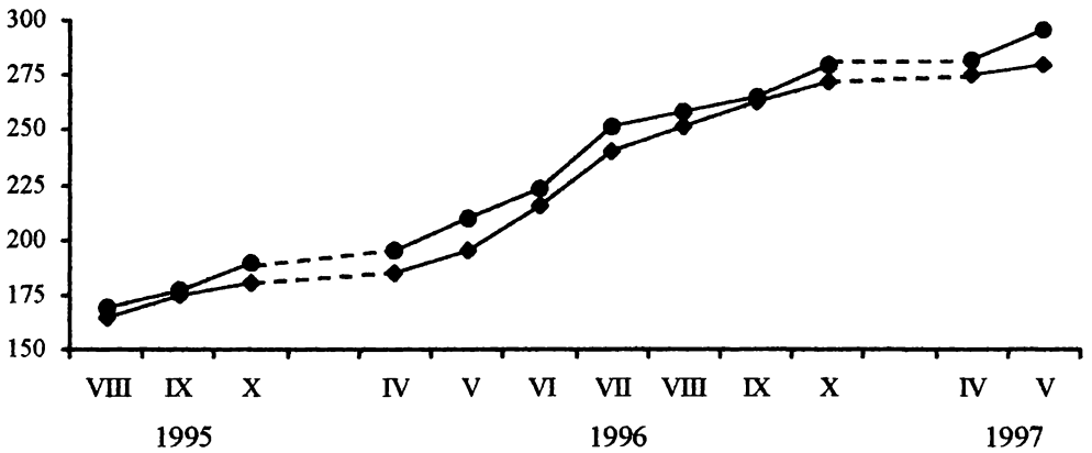
Abb. 1. Längenwachstum bei Vipera nikolskii im Norden der Niederwolgaregion: ◆ – Männchen, ● – Weibchen. Die Punktlinie zeigt den vermutlichen Trend der Wachstumskurve
